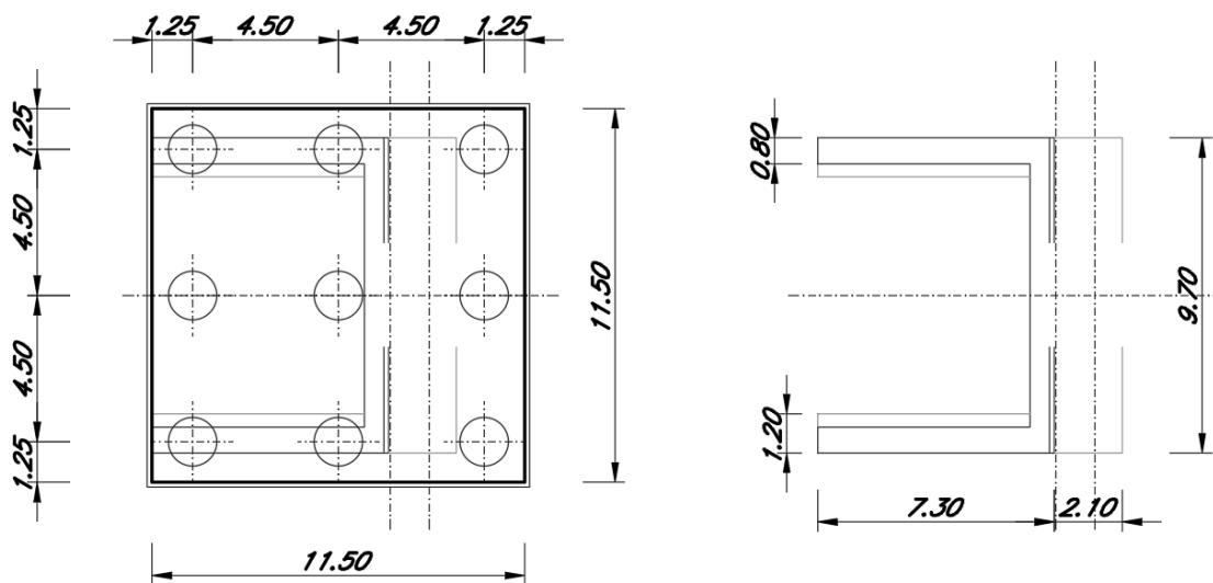
Figura 1-5 - elaborati grafici spalla A (mobile)
