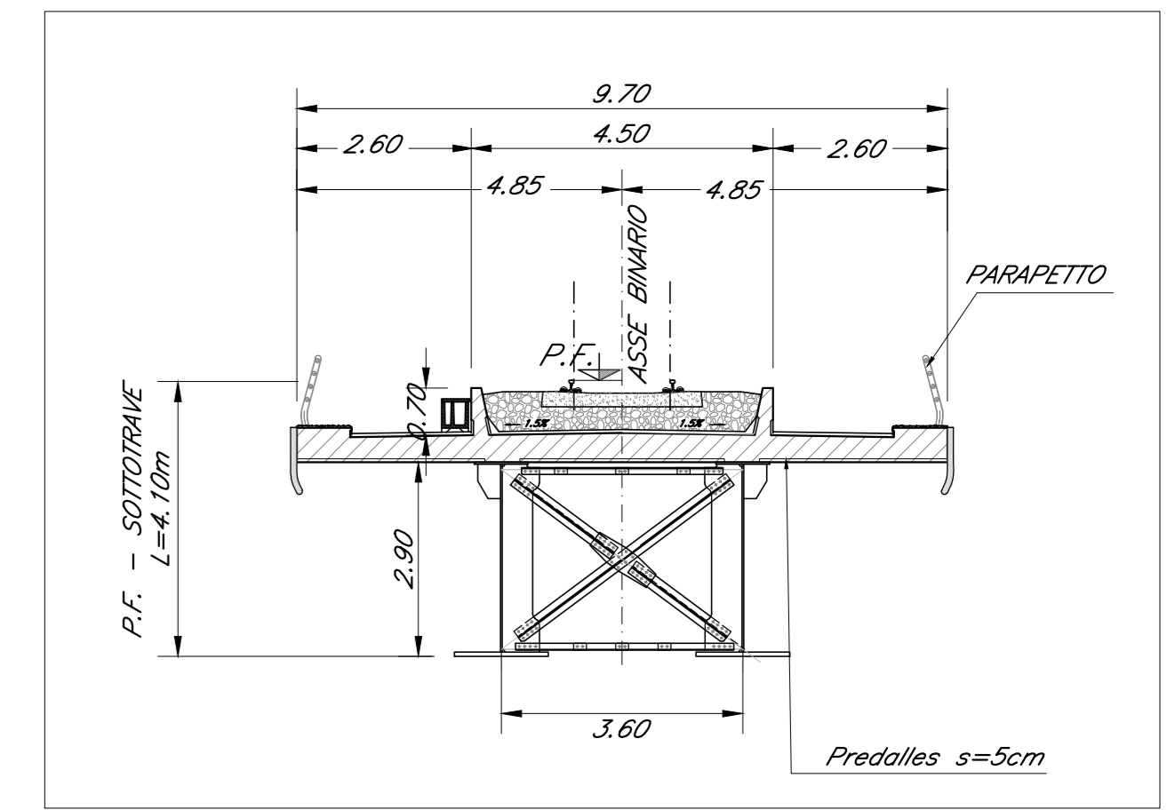
SEZIONE TIPO ACCIAIO 40M Scala 1:100
