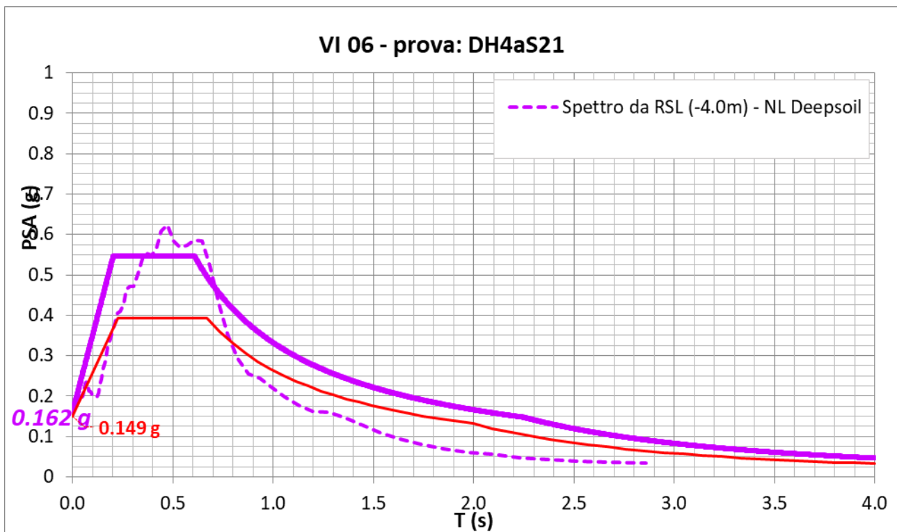
Figura 4-20 - Confronto spettro NTC (rosso) con spettro RSL (blu)
