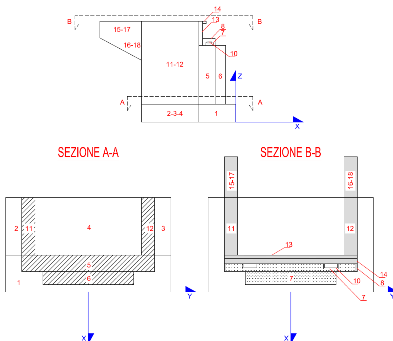
Figura 4-4: Schema qualitativo della geometria della spalla
