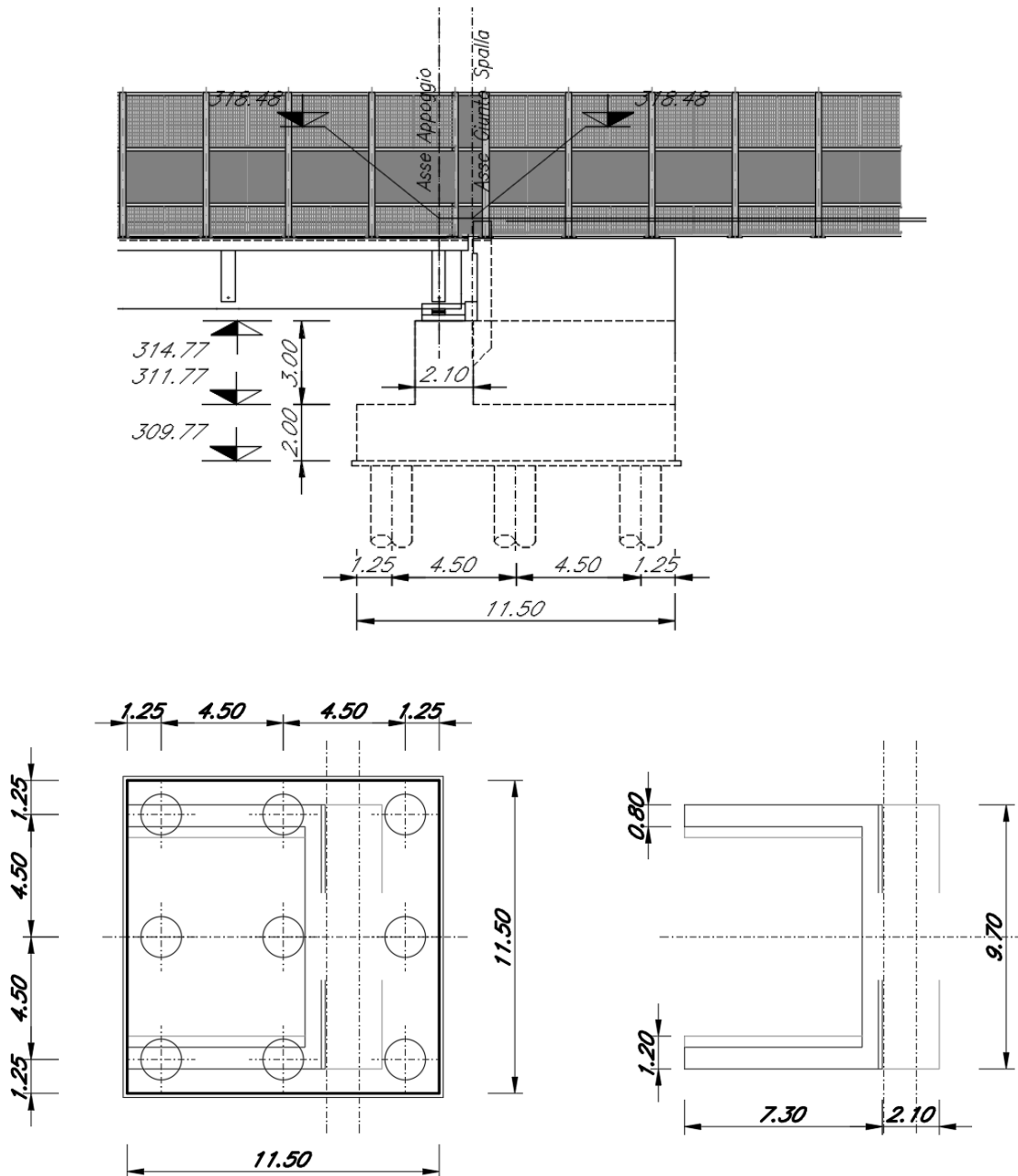
Figura 1-5: elaborati grafici spalla B (fissa)
