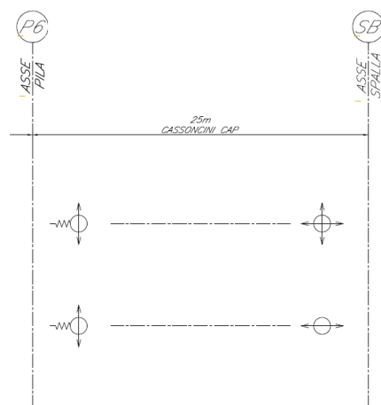
Figura 1-1-1: schema appoggi
