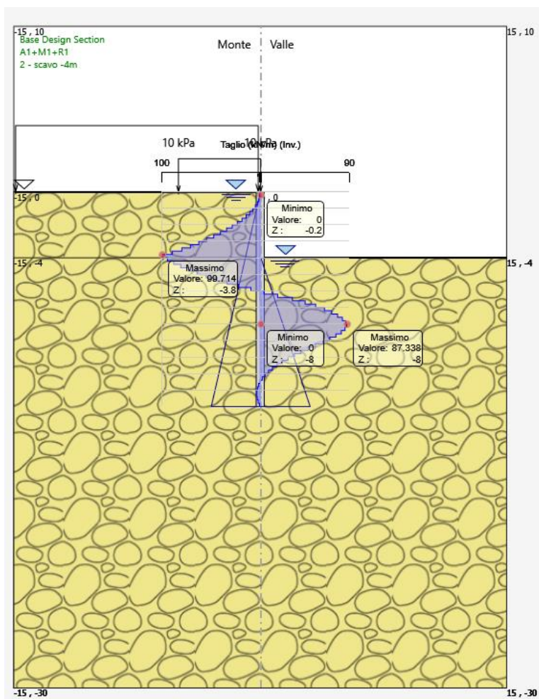
Figura 4: forza di taglio allo SLU-STR
