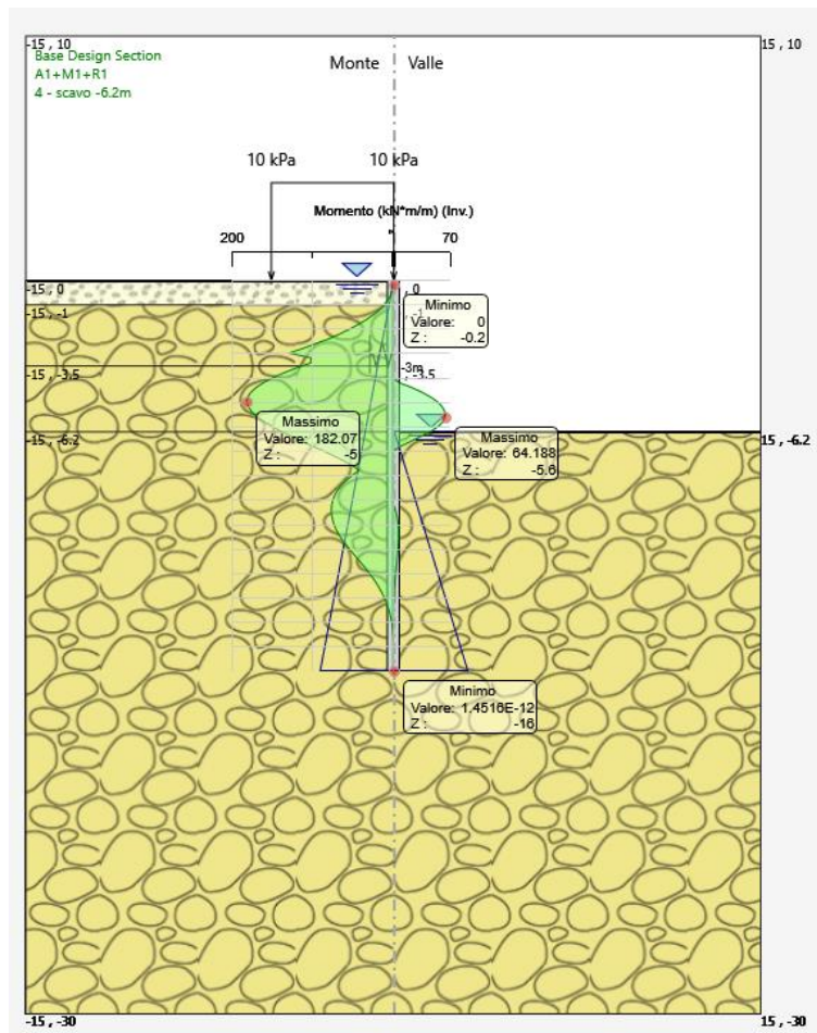
Figura 5: momento flettente allo SLU-STR
