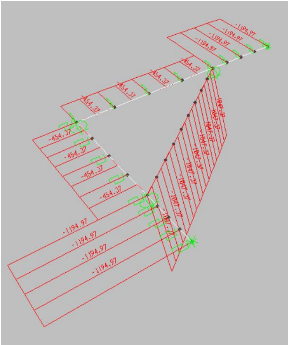
Figura 8: forza assiale allo SLU-STR
