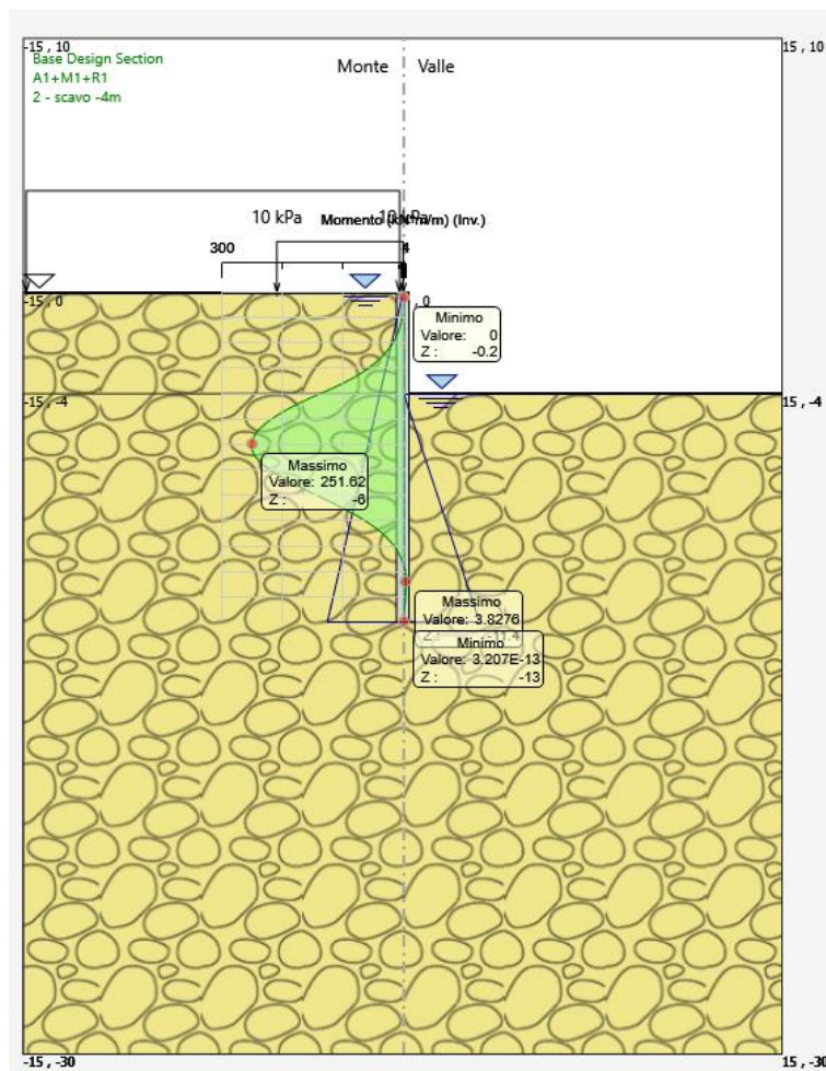
Figura 3: momento flettente allo SLU-STR
