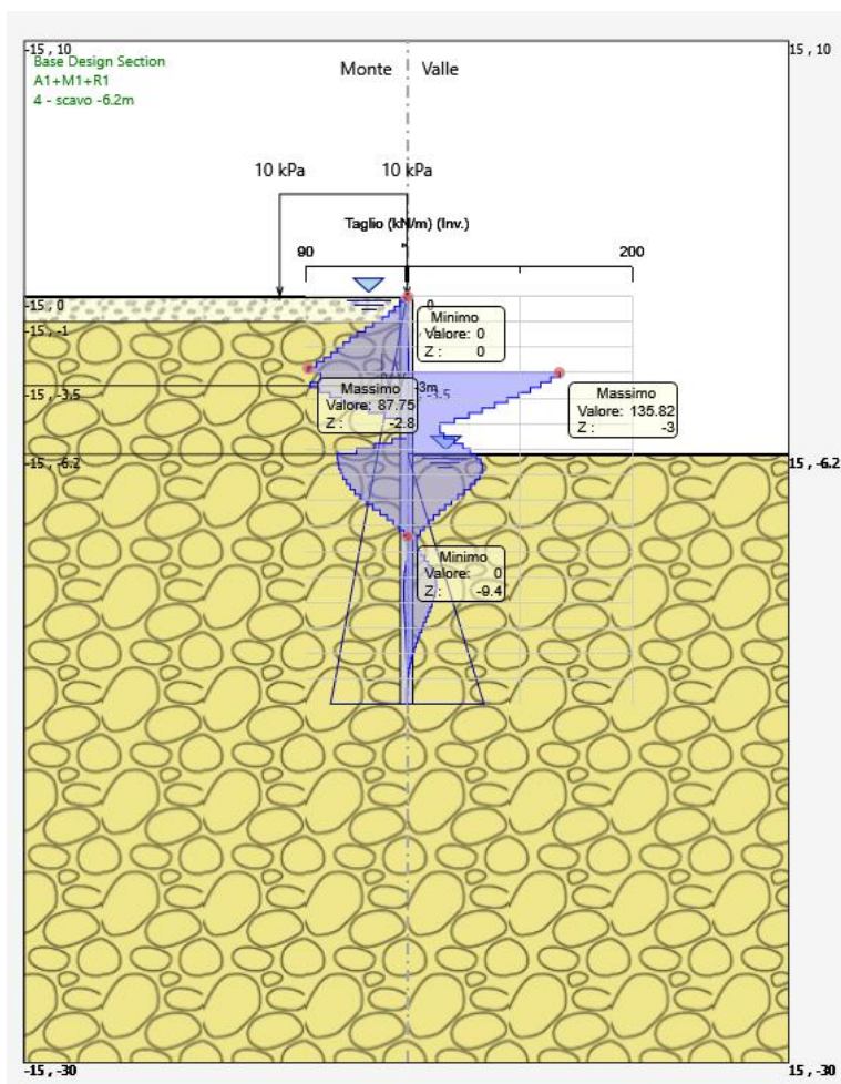
Figura 6: forza di taglio allo SLU-STR
