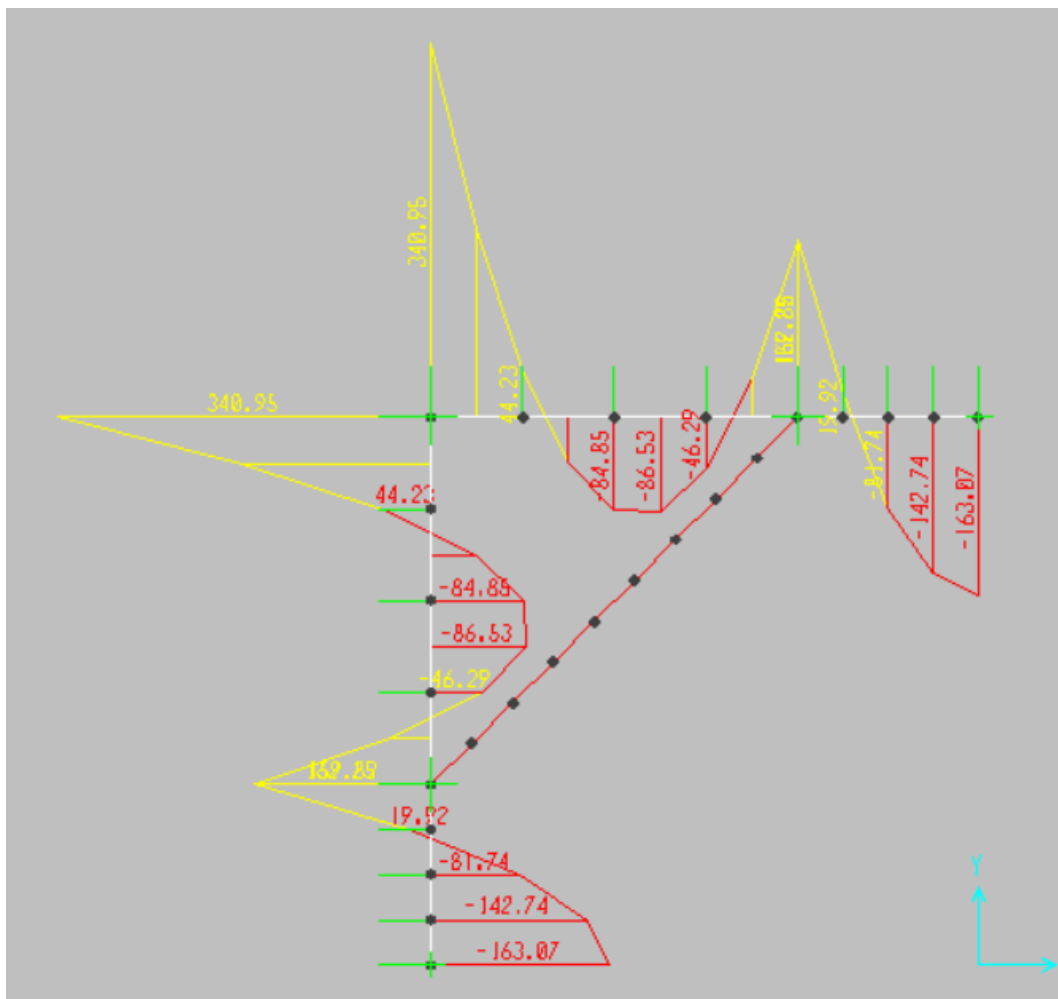
Figura 7: momento flettente allo SLU-STR
