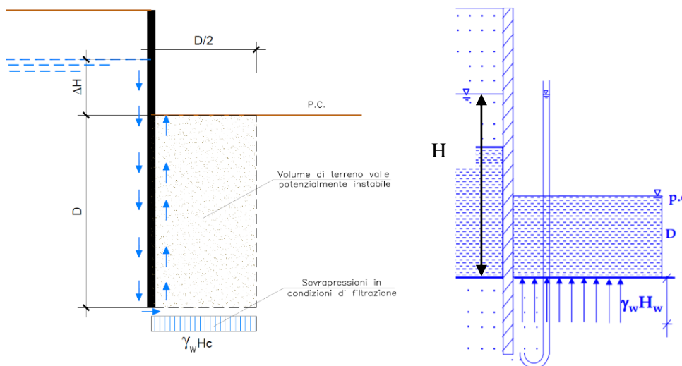
Figura 10: Schema di filtrazione per effetto di scavi sotto falda a valle di opere di sostegno
