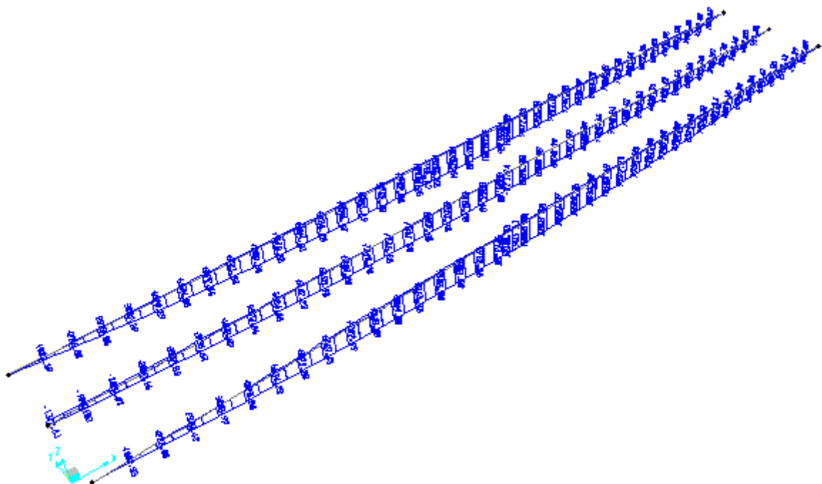
Figura 3. Fase 2 M-V-N (kN-m)
