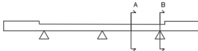
Figura 13: sezioni di interesse per la massimizzazione delle sollecitazioni
