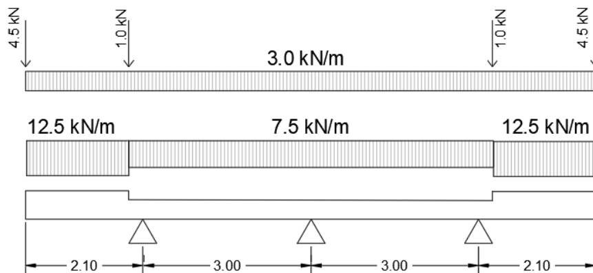
Figura 8: carichi permanenti sulla soletta
