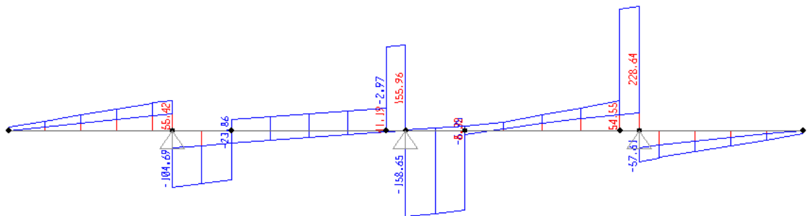
Figura 17: involuipo del taglio SLU
