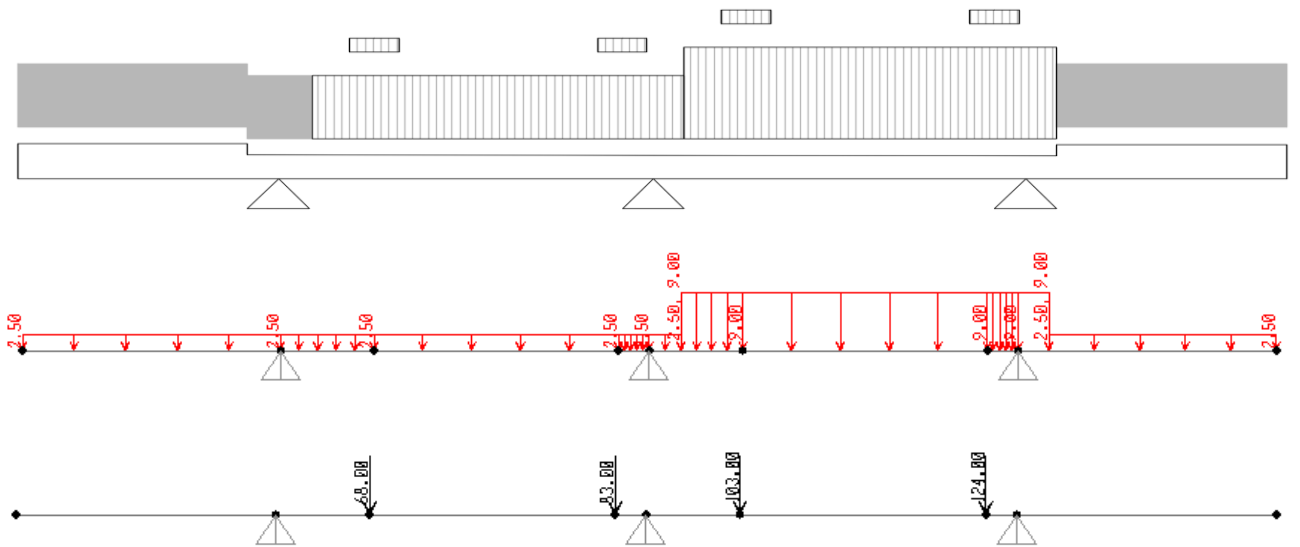
Figura 15: condizione di carico 2
