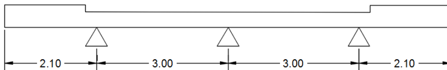
Figura 7. Schema statico
