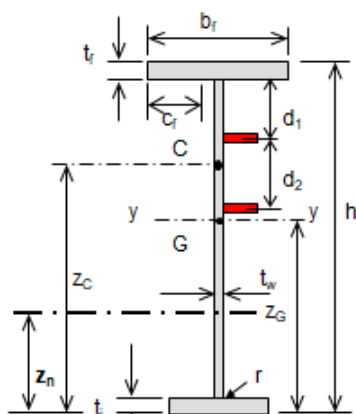
SEZIONE MONO-SIMMETRICA
