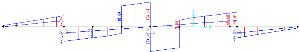
Figura 16: involuipo momento flettente SLU
