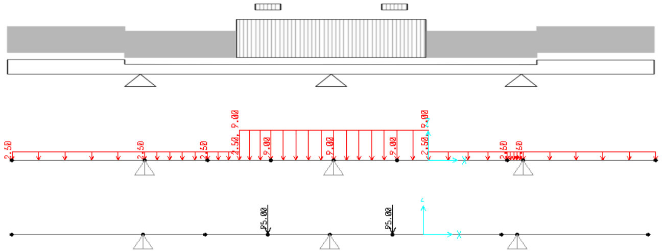
Figura 14: condizione di carico 1
