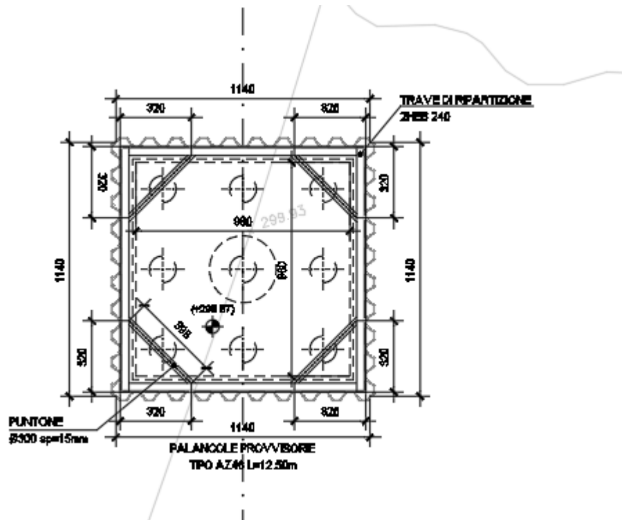
Fig. 2 –Pianta dell'opera
