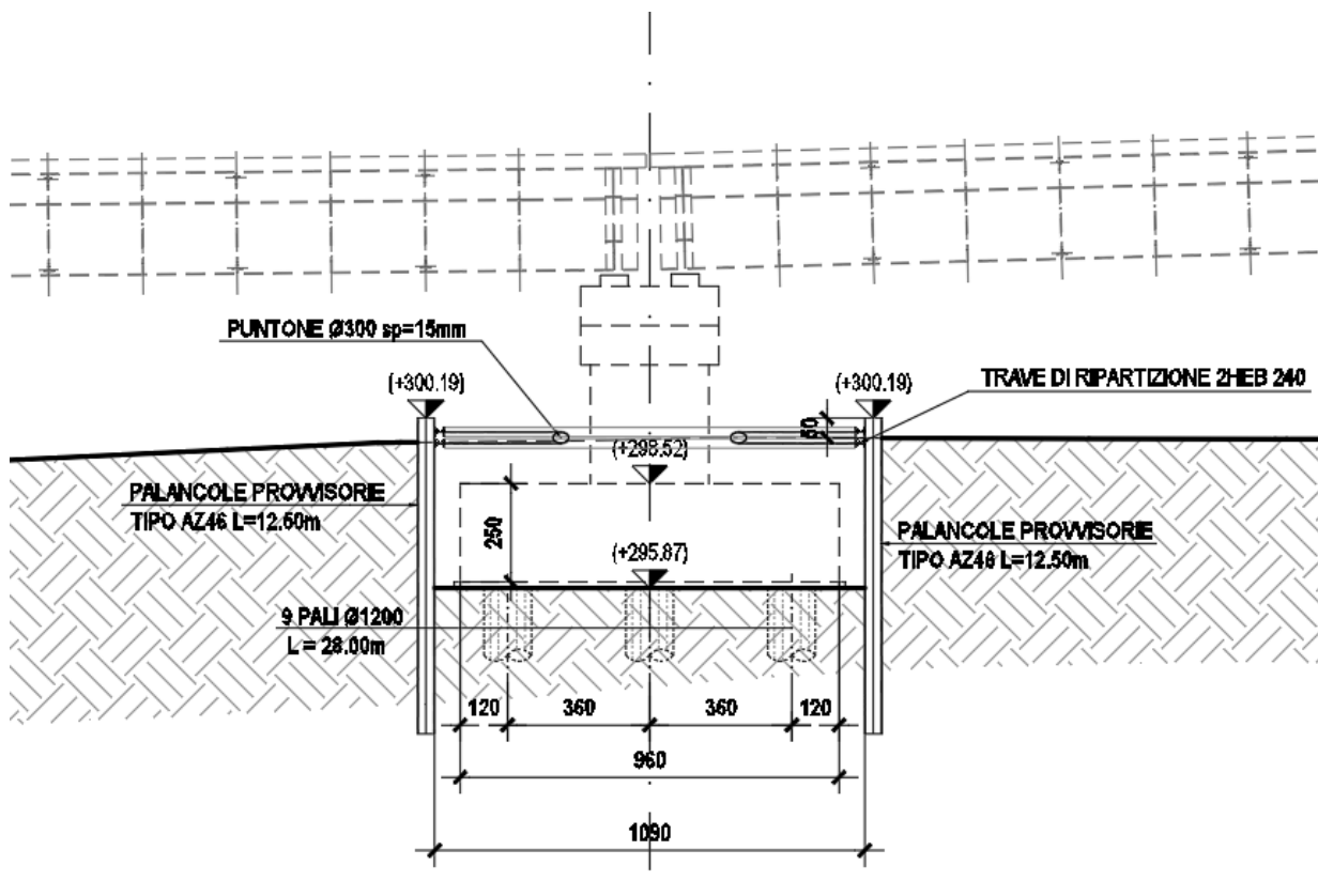
Fig. 1 – Sezione trasversale dell'opera
