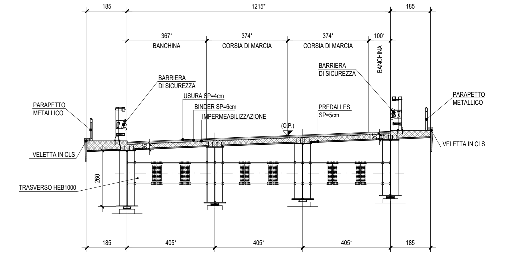
SEZIONE TRASVERSALE IMPALCATO 4 TRAVI CAMPATA - Scala 1:100
