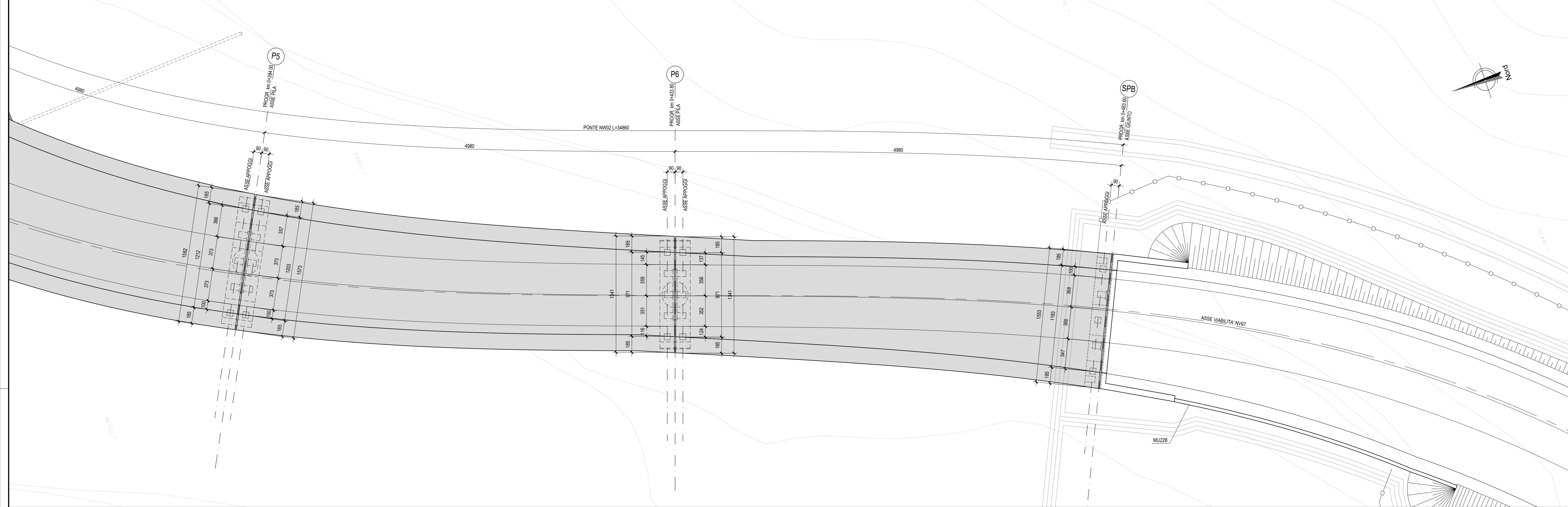
PIANTA TRAVI - Scala 1:200
