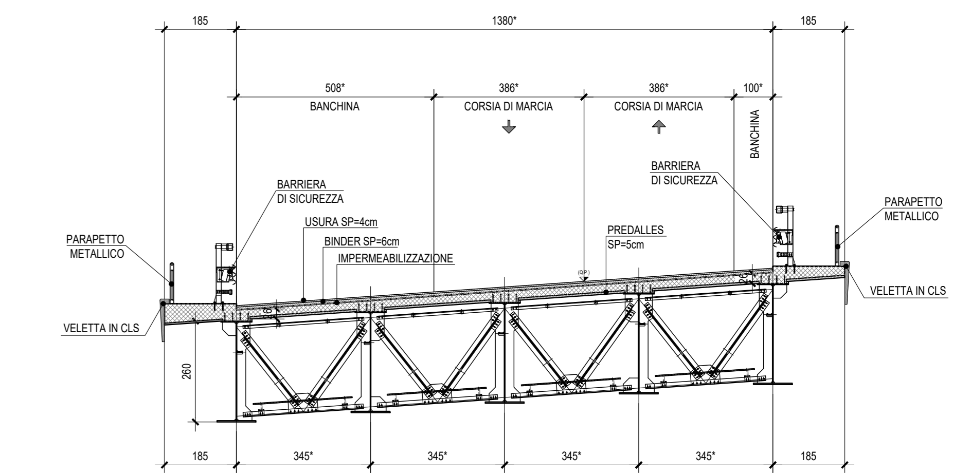
SEZIONE TRASVERSALE IMPALCATO 5 TRAVI CAMPATA - Scala 1:100
