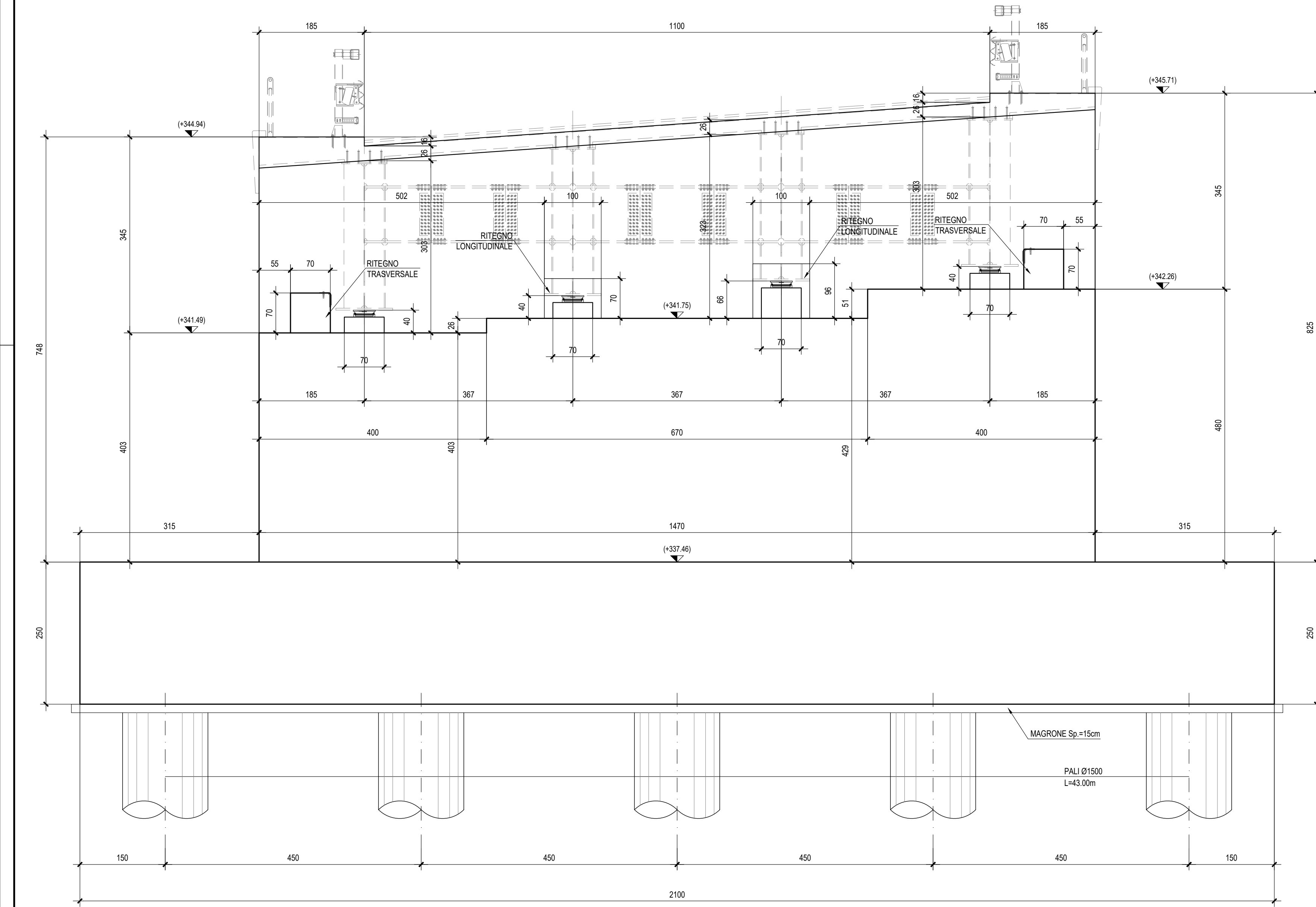
VISTA A-A - Scala 1:50
