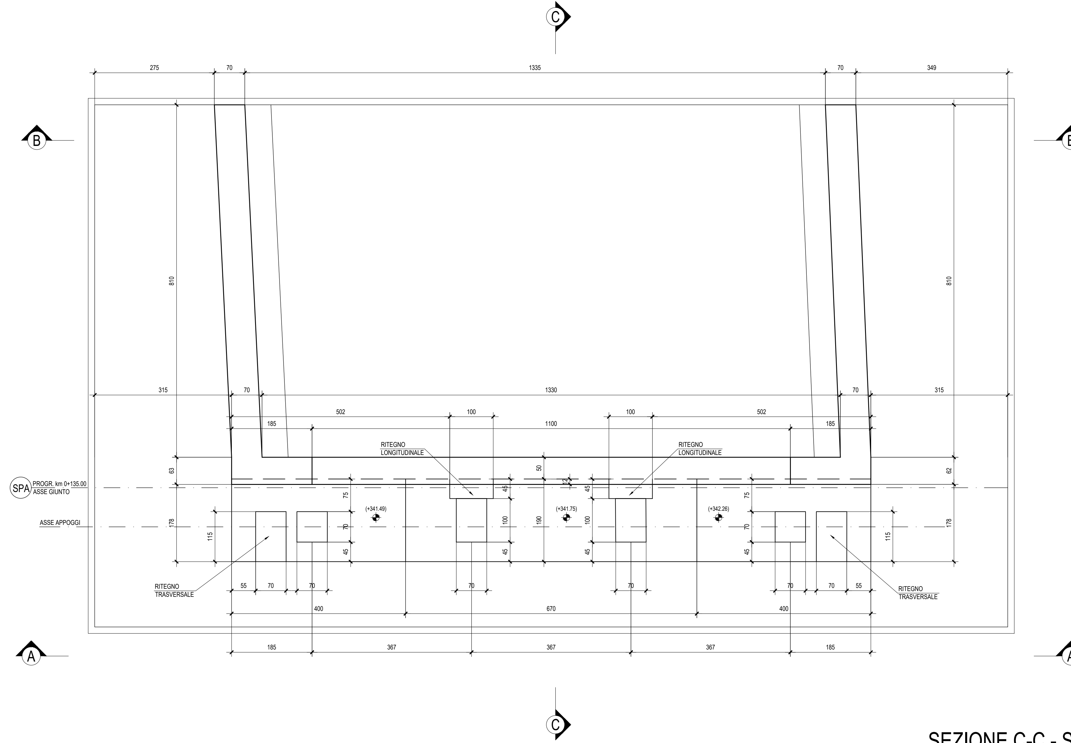
SEZIONE C-C - Scala 1:50
