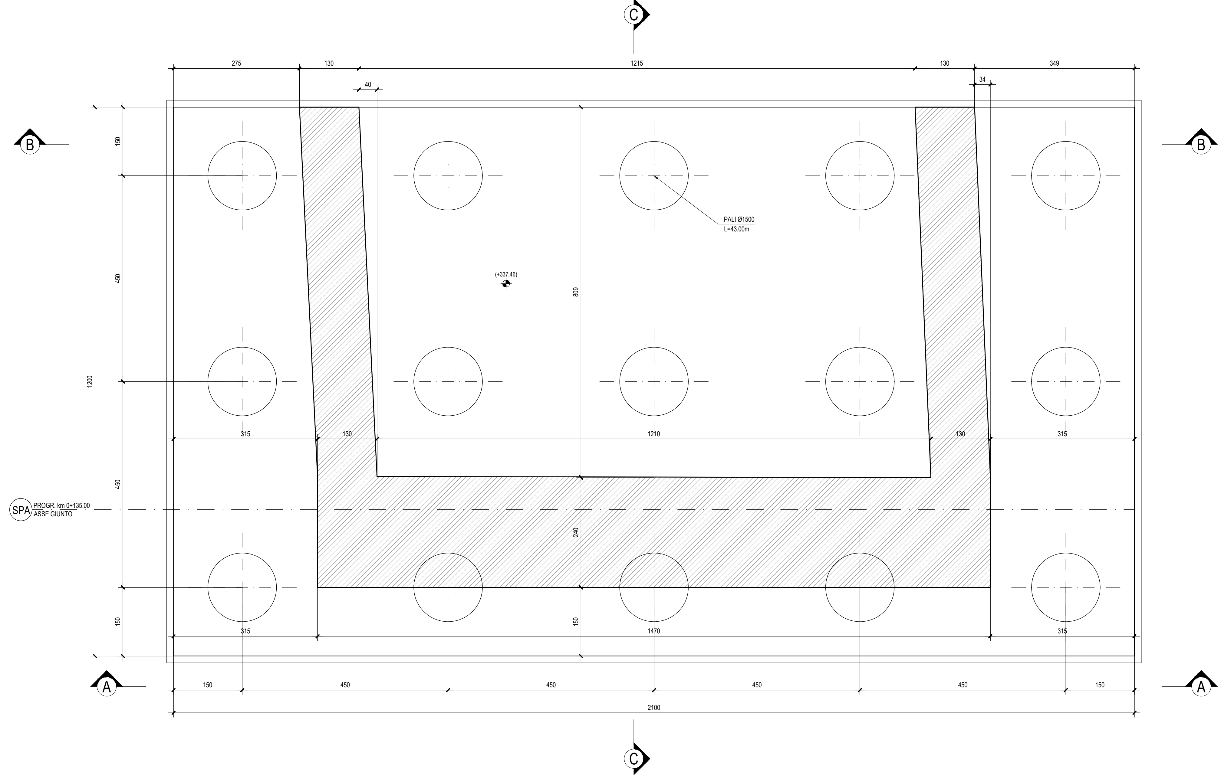
PIANTA SPICCATO - Scala 1:50
