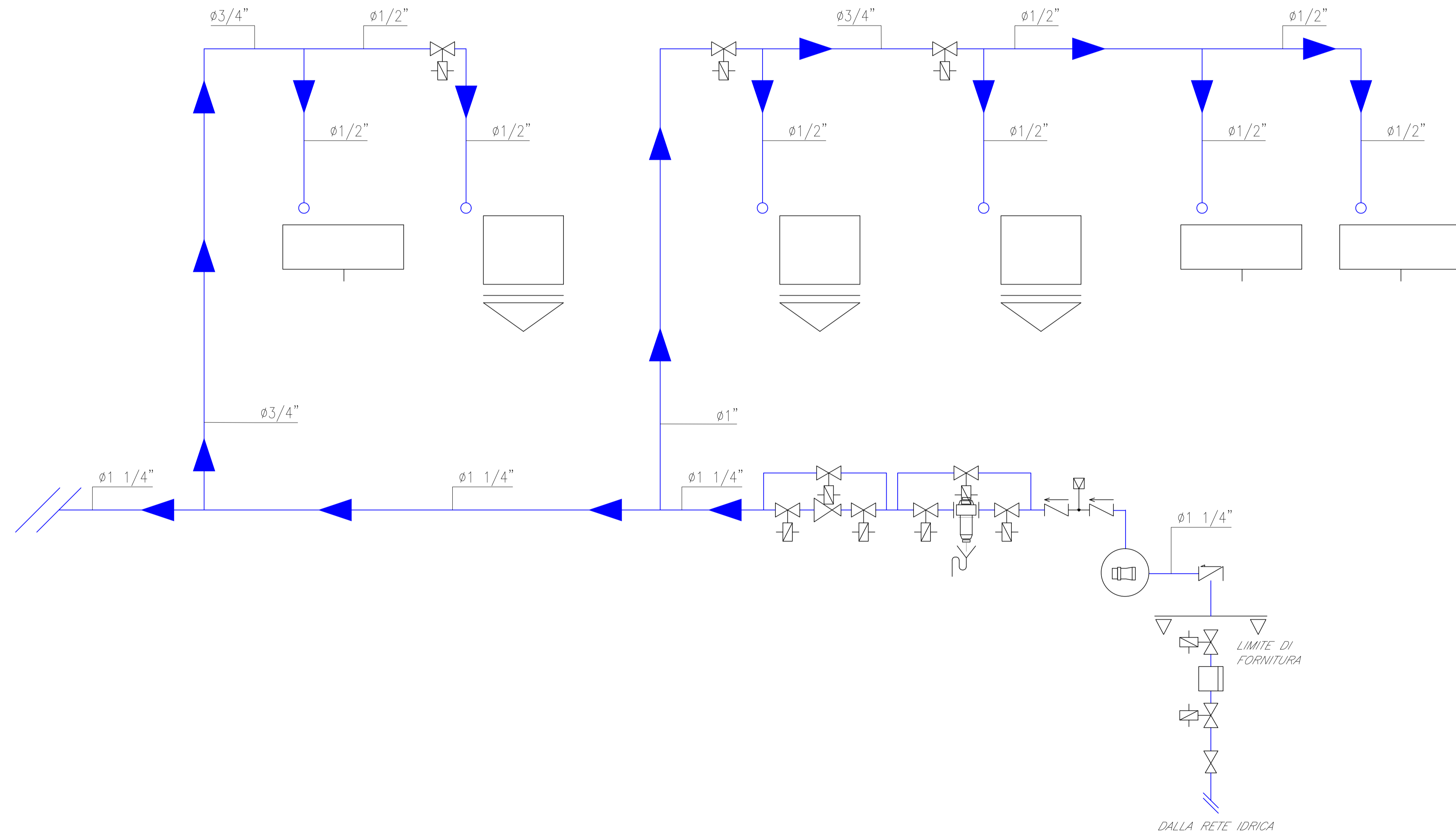
SCHEMA FUNZIONALE IMPIANTO IDRICO SANITARIO - IMPIANTO ADDUZIONE
