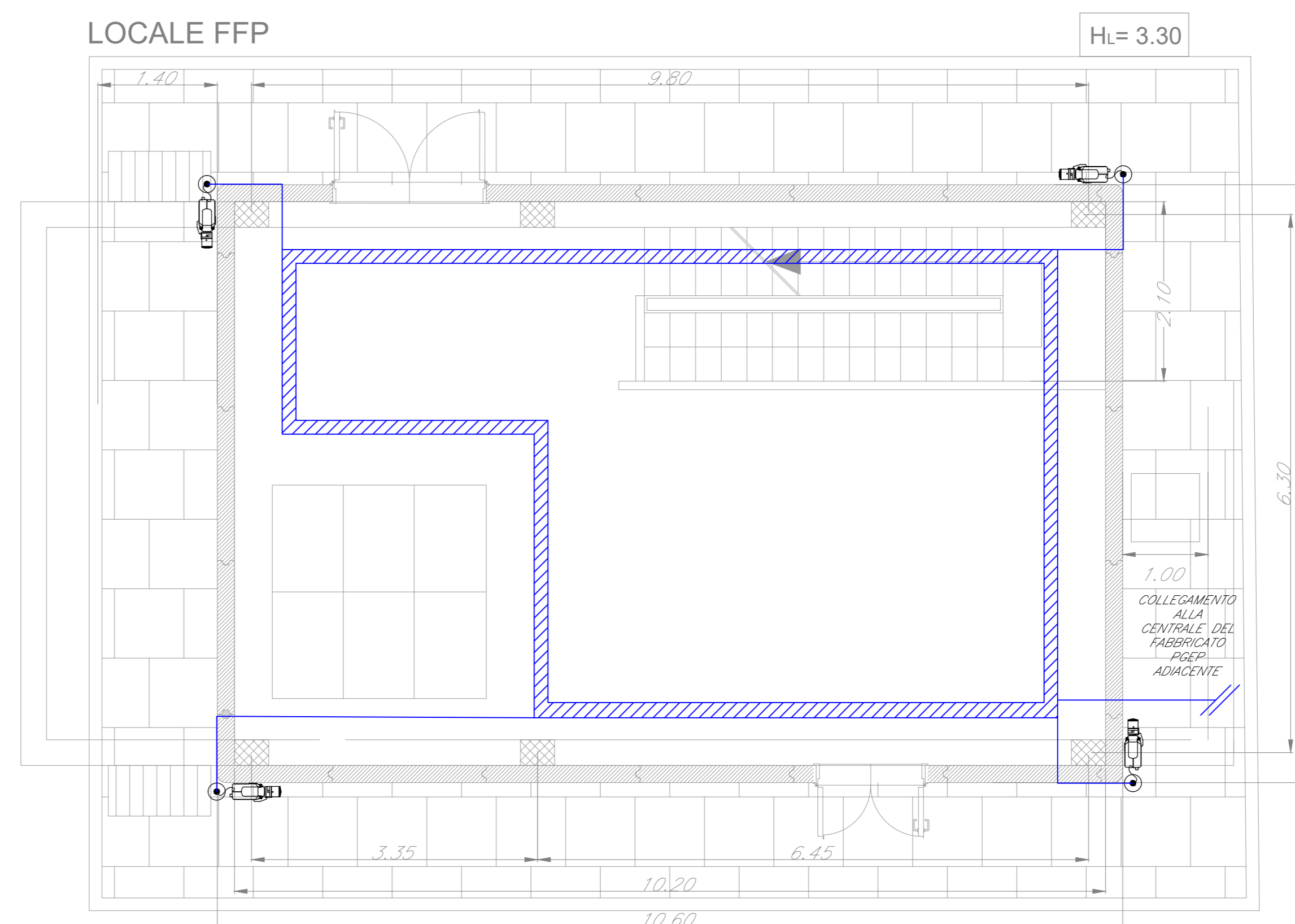
LAYOUT IMPIANTO TVCC - PIANO TERRA FABBRICATO FFP
