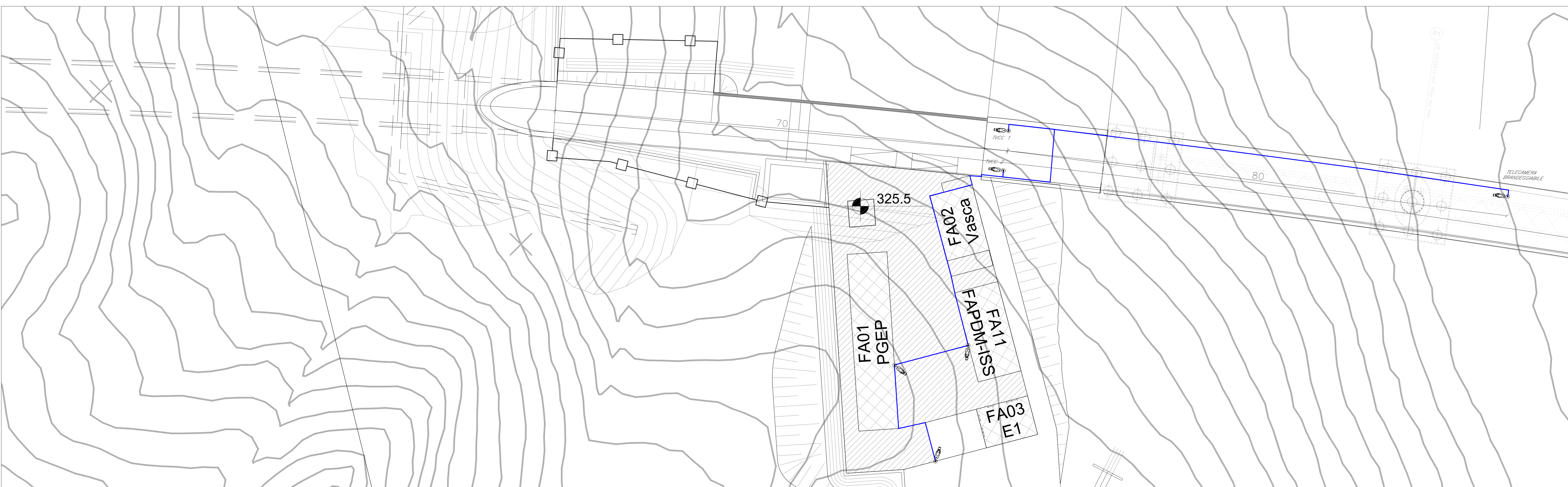
LAYOUT IMPIANTO TVCC - IMBROCCO GALLERIA E PIAZZALE SCALA 1:250
