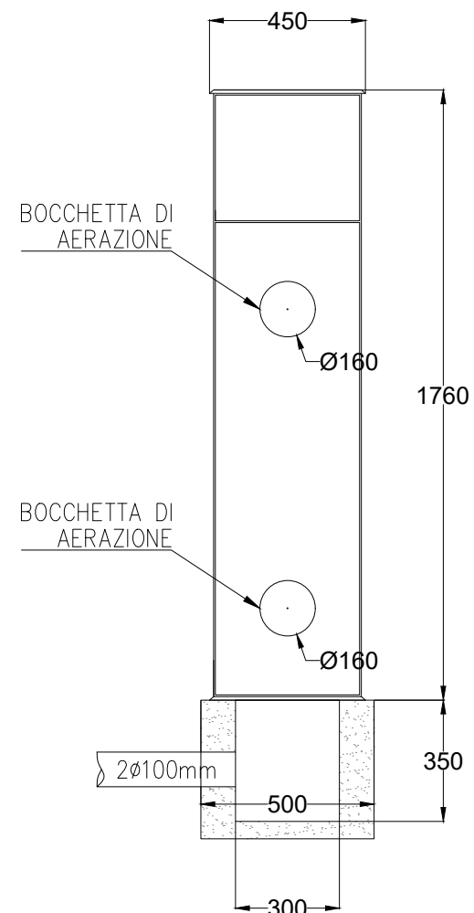
VISTA LATERALE
