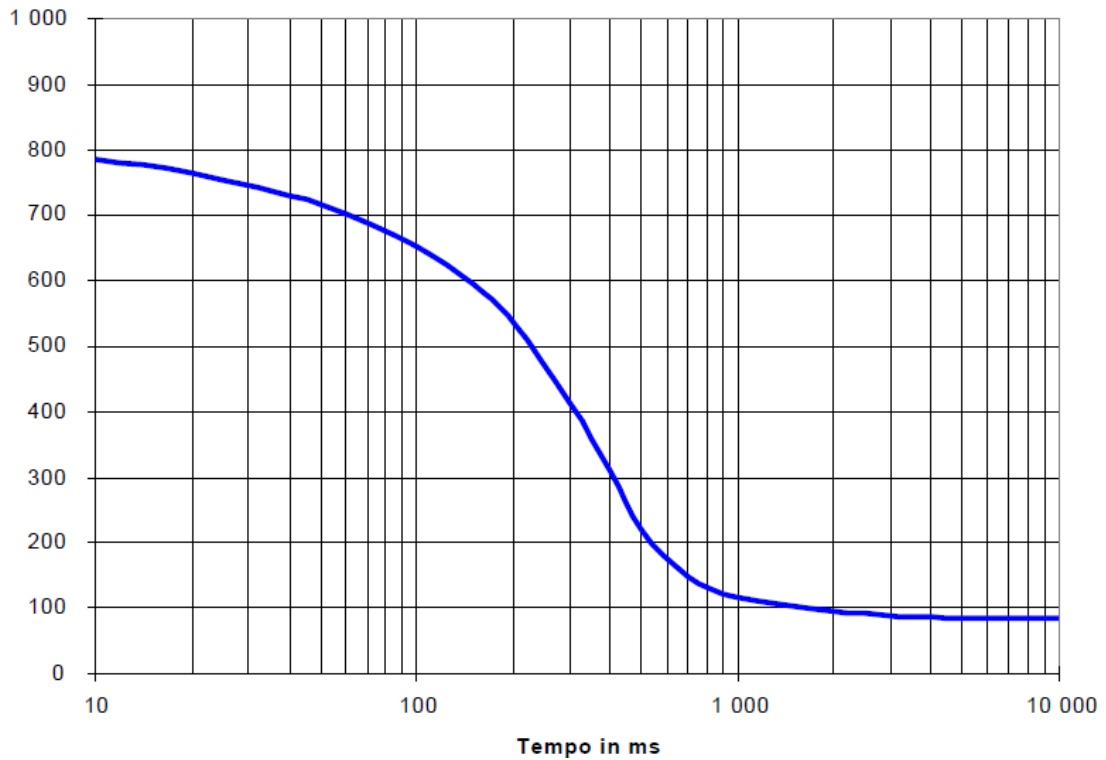
Figura 4 – Curva Tempo-Tensione (Norma CEI EN 50522 § 5.4.3)
