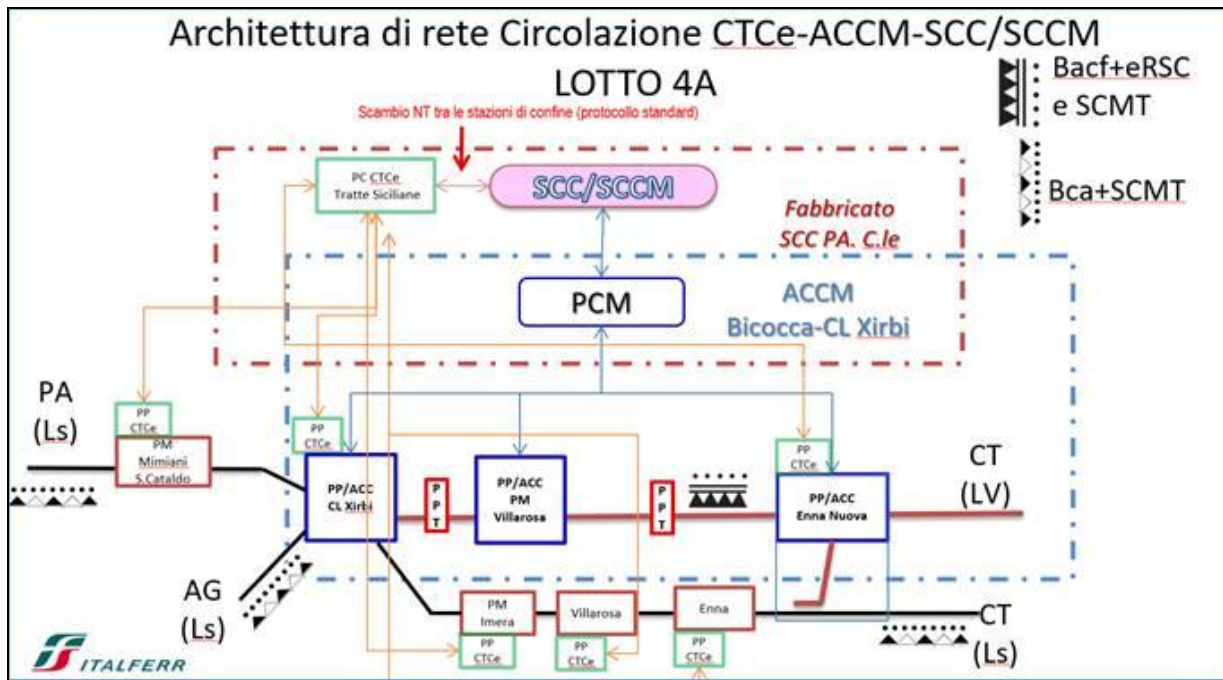
Figura 20 Architettura ACCM - SCCM - CTce
