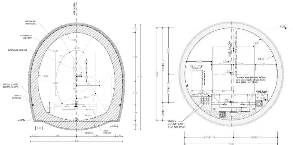
Figura 2 Sezione di intradosso galleria di linea a singolo binario per scavo in tradizionale (sezione corrente a sx) e per scavo in meccanizzato (sezione corrente a dx)
