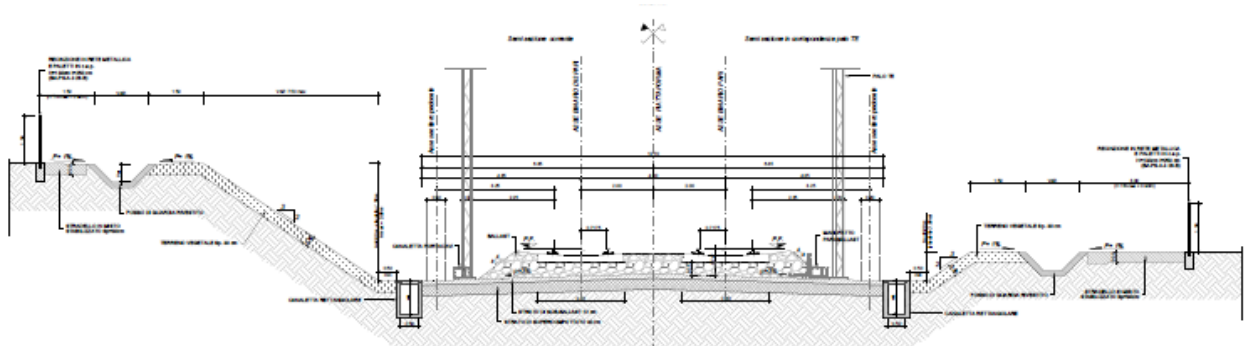
Figura 19 – Sezione Tipo Trincea a doppio binario
