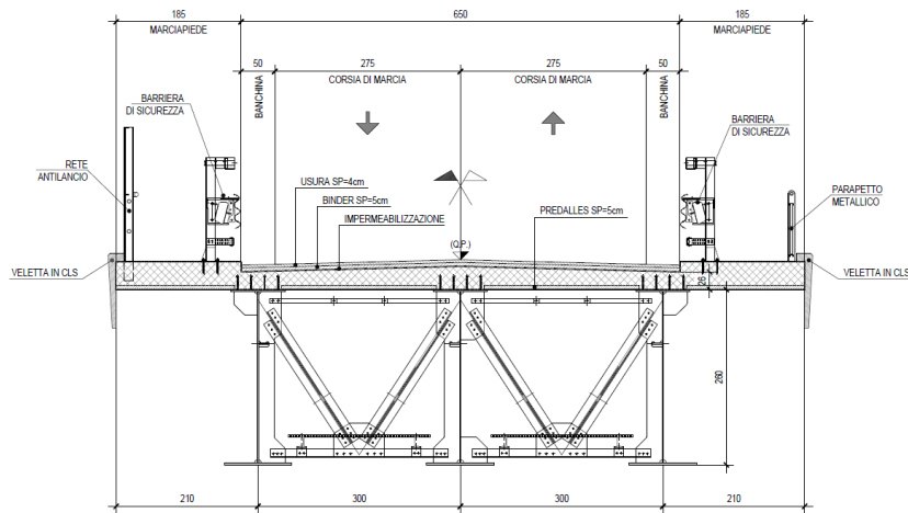
Figura 11 – Sezione tipo NW01 impalcato in cap da 40 m
