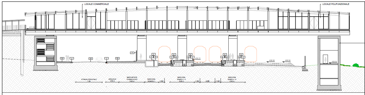
Figura 7 -Stazione Caltanissetta Xirbi – sezione rappresentativa del sovrappasso STAZIONE NUOVA ENNA
