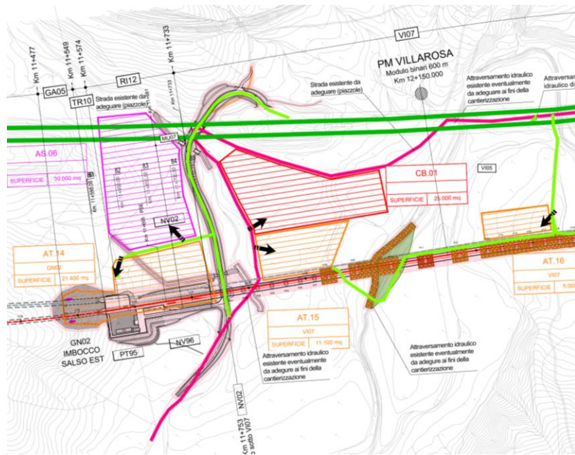
Figura 22 Stralcio nuova viabilità locale (NV02)
