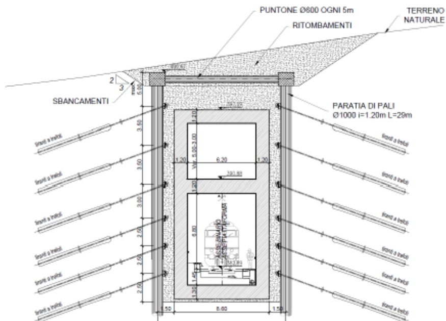
Figura 4 Sezione tipo GA01
