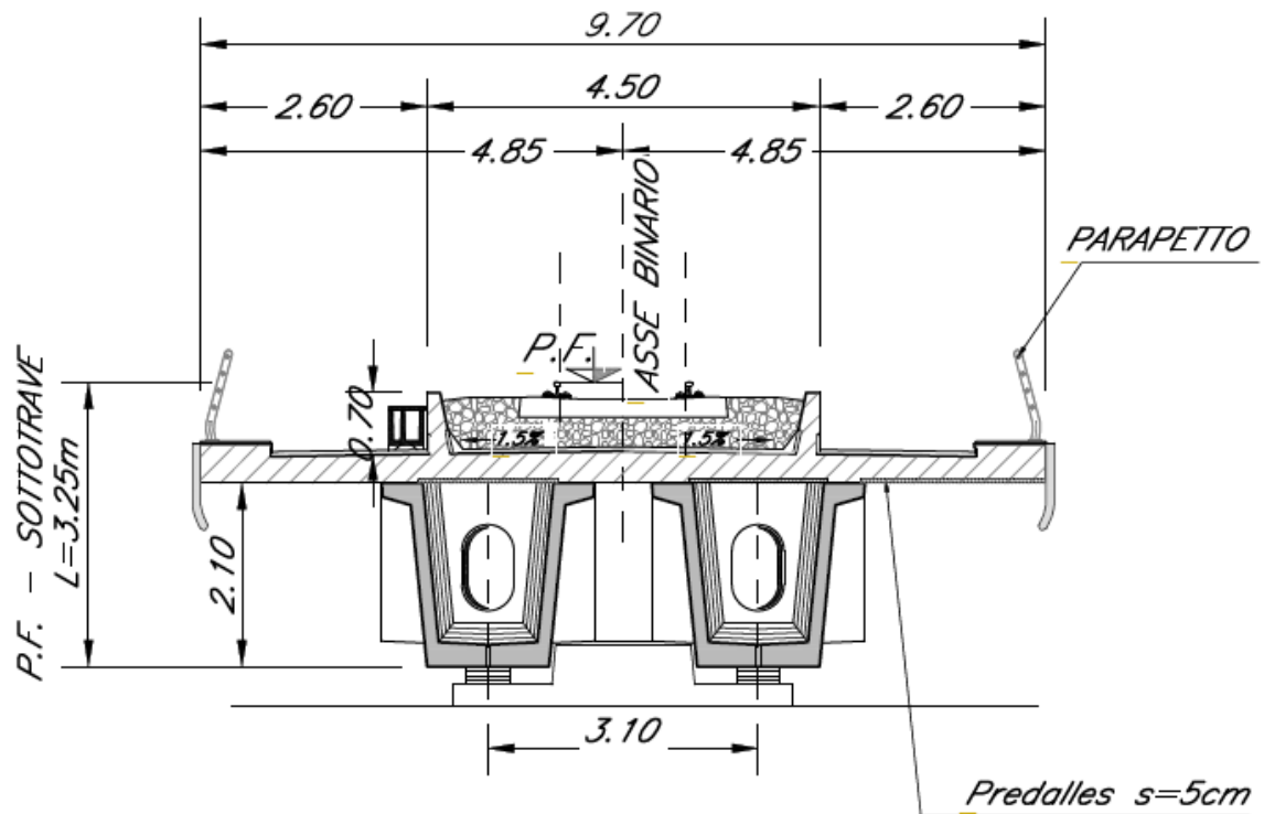
Figura 8 -Sezione impalcato in cap da 25 m – singolo binario
