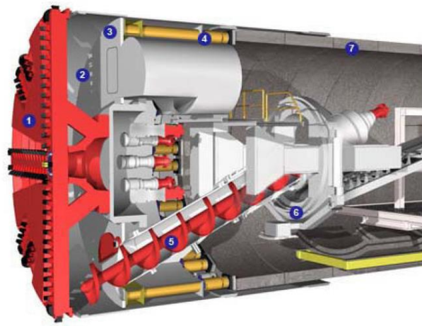
Figura 3 Schema di una macchina TBM, tipo EPB (1. Testa Fresante; 2. Camera di scavo; 3. Parete di contenimento dotata di sistema d'accesso (camera iperbarica) alla camera di scavo; 4. Pistoni di avanzamento; 5. Coclea; 6. Erettore dei conchi; 7. Anelli di sostegno già posti in opera)
