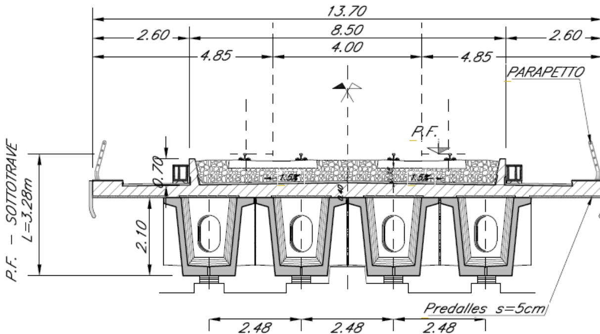
Figura 10 - Sezione impalcato in cap da 25 m – doppio binario
