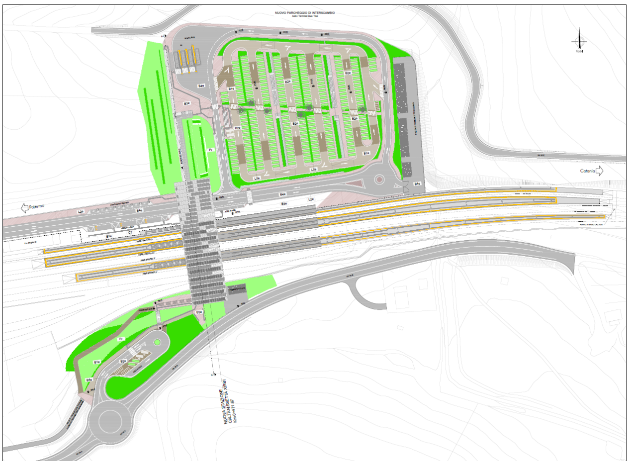
Figura 6 - Stazione Caltanissetta Xirbi - Planimetria assetto generale
