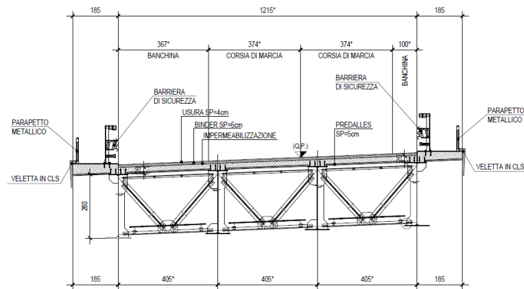
Figura 12 – Sezione tipo NW02 con impalcato in cap da 49 m
