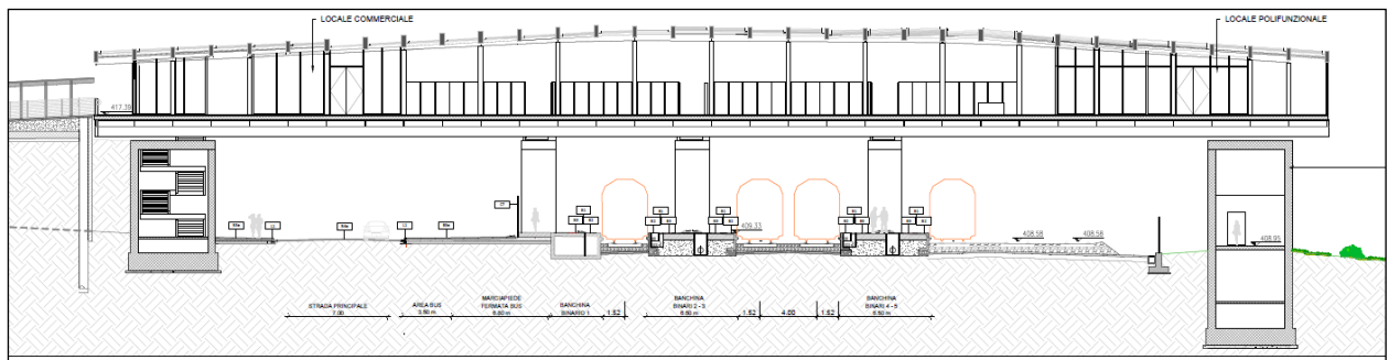
Figura 13 -Stazione Caltanissetta Xirbi – sezione rappresentativa del sovrappasso
