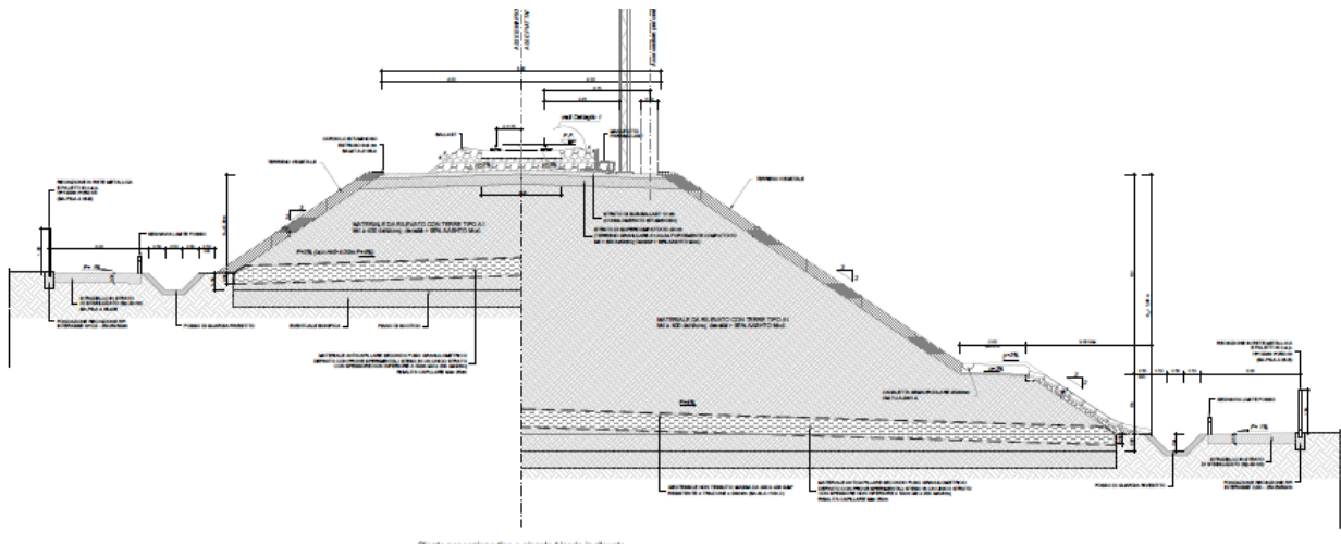
Figura 18 – Sezione Tipo Rilevato a singolo binario
