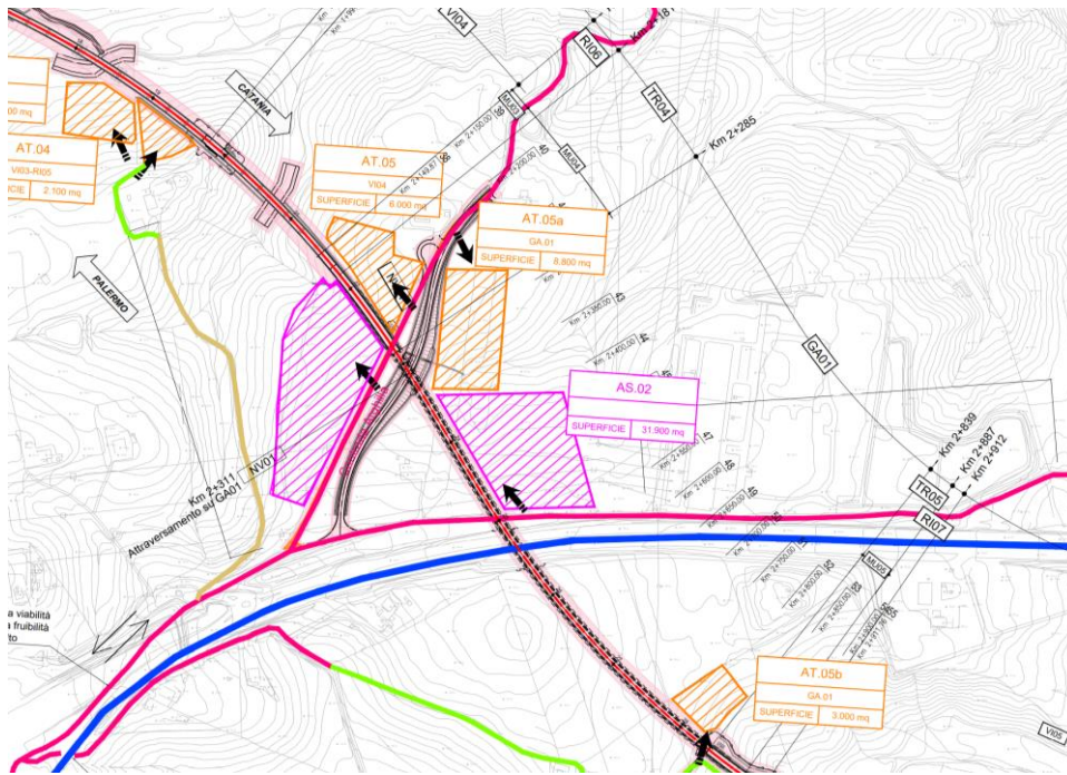
Figura 21 Stralcio deviazione viabilità locale contrada Arghillà e interferenza GA01 –SS640
