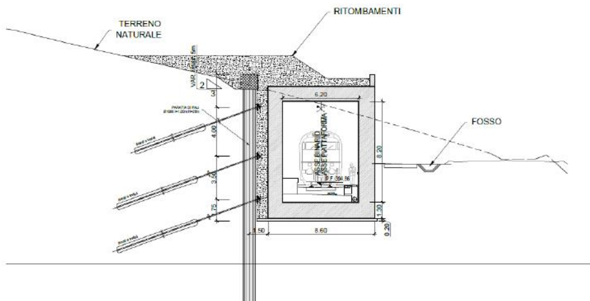
Figura 5 Sezione tipo GA51
