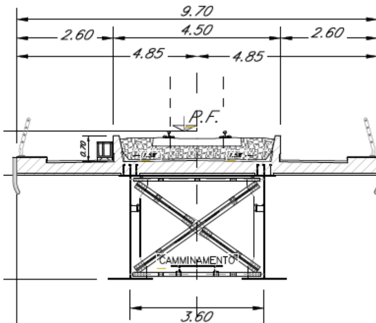
Figura 9 -Sezione tipo campate a sezione mista acciaio – cls (da 40 - 50 – 60 m) a singolo binario
