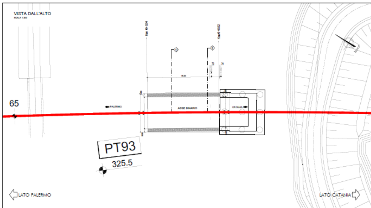
Figura 15 Vista dall'alto SL02
