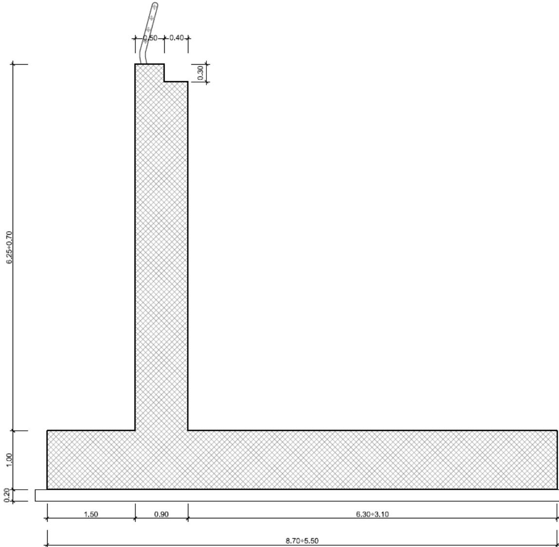
Figura 2 – Sezione trasversale 1
