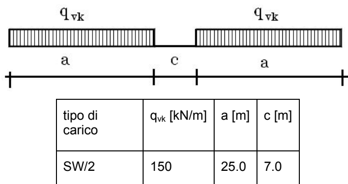
Figura 13 – Treno di carico SW/2.
