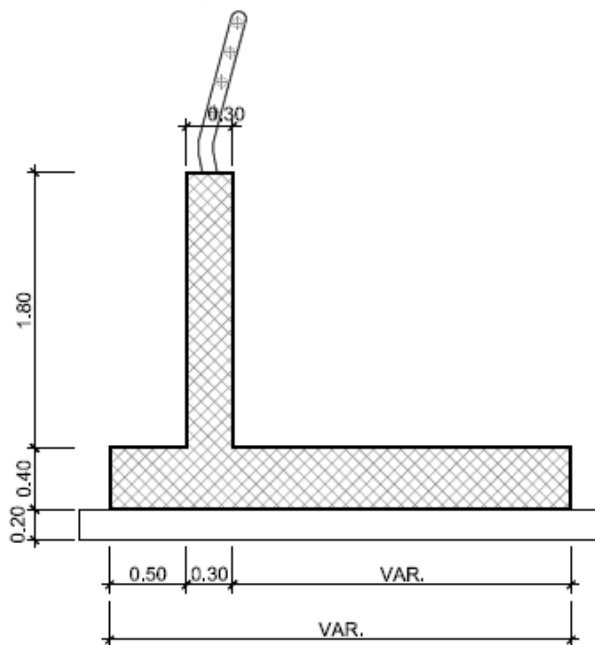
Figura 3 – Sezione trasversale 2
