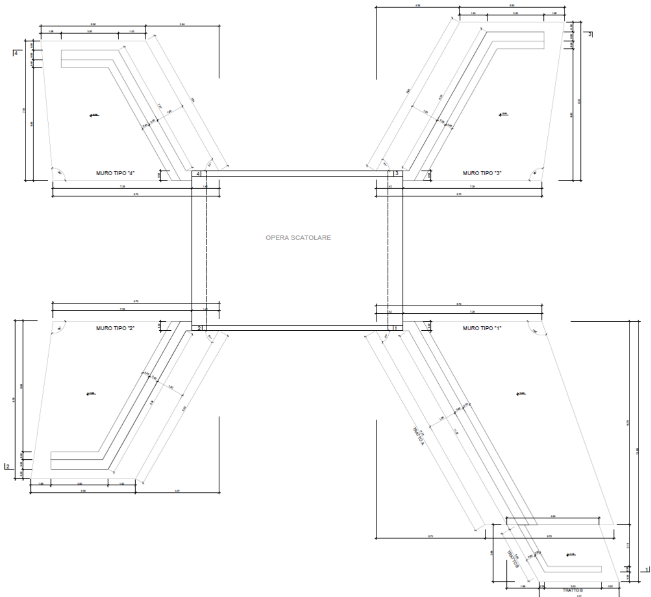
Figura 1 – Planimetria
