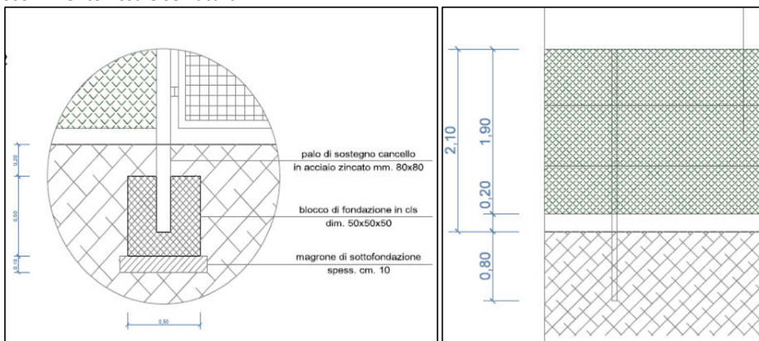
Figura 2 – Particolare della recinzione delle aree di progetto.
