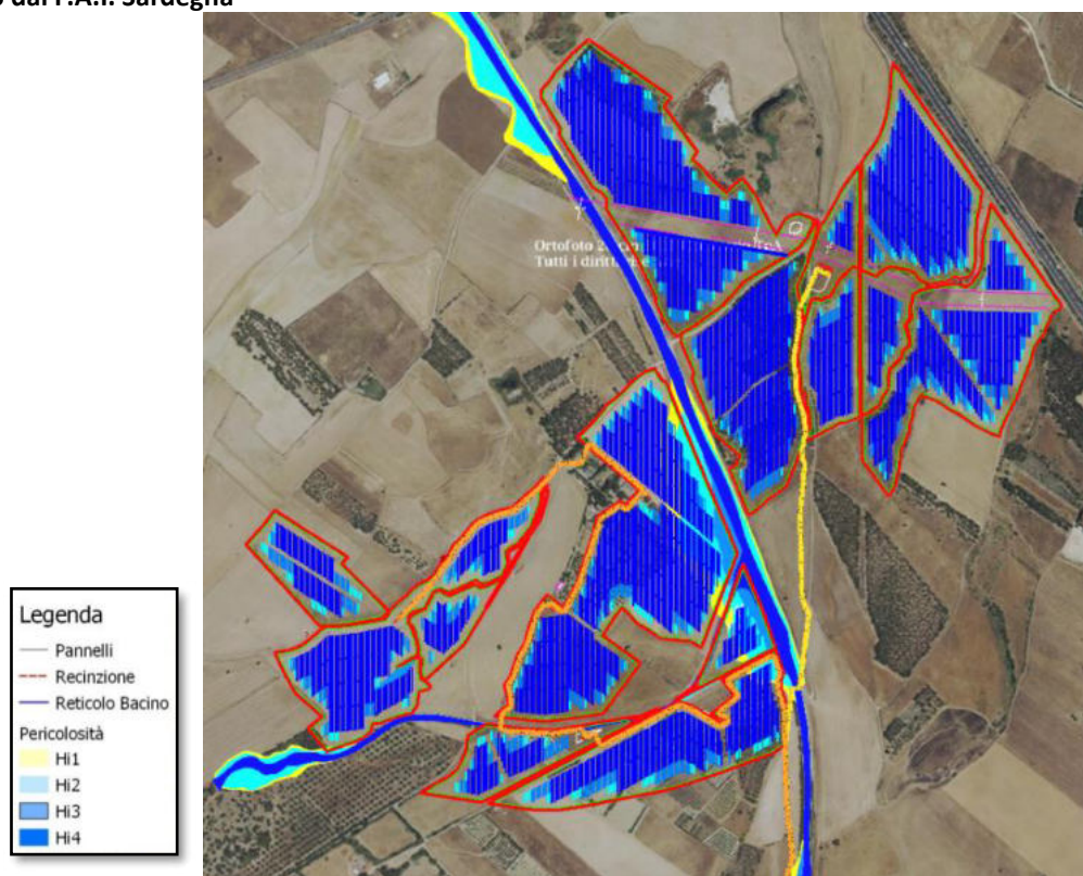
Figura 10 – Studio idraulico aree di progetto.
