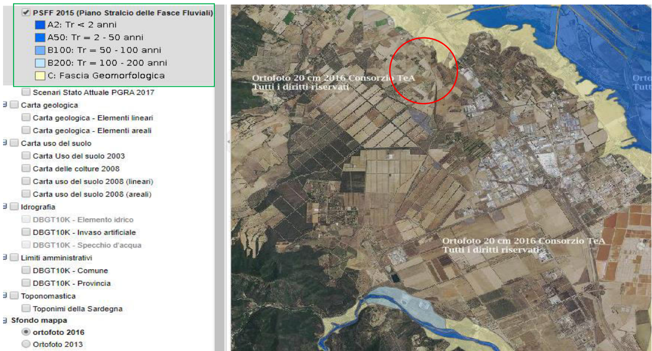
Figura 7 – Stralcio del Piano Fasce Fluviali (PSFF)_Fonte Geoportale Sardegna.
