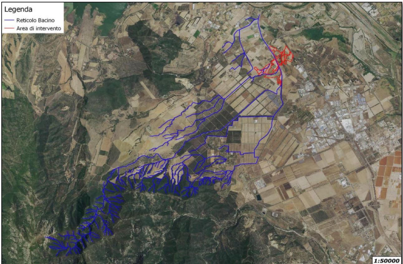
Figura 6 – Elaborazione GIS reticolo bacino idrografico Riu S'isca de Arcosu.
