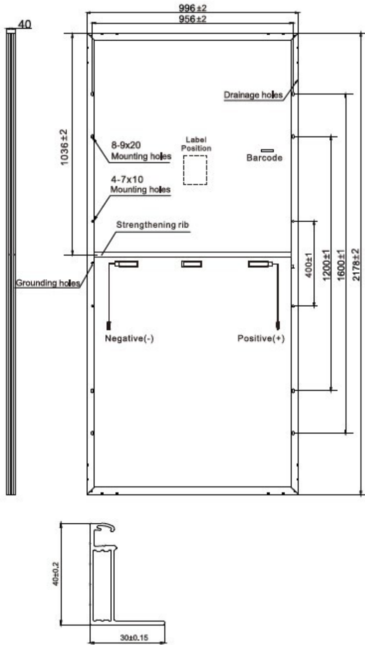
figura 3 – caratteristiche dimensionali dei moduli
