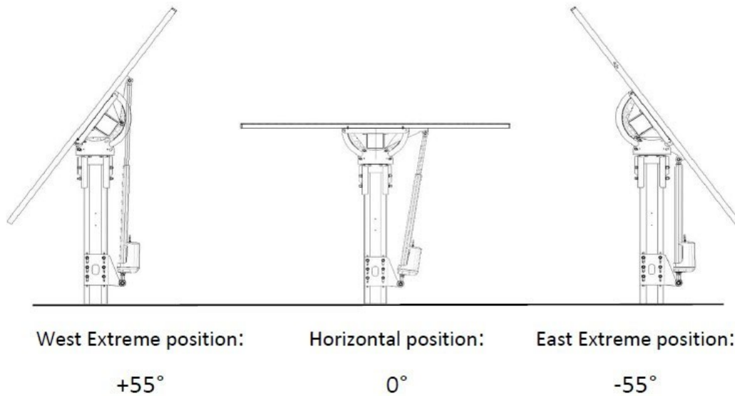
Fig. 5 - Angolo di rotazione del tracker
