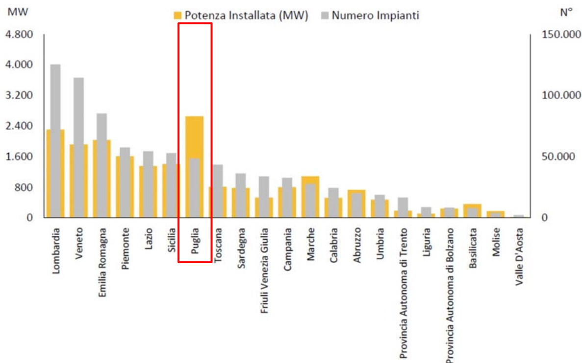
Distribuzione Regionale della numerosità e della potenza a fine 2018 (Italia – fonte Rapporto GSE 2018)
