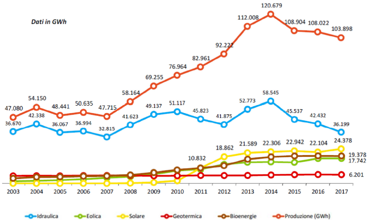
Evoluzione della produzione da fonti rinnovabili (Italia – fonte Rapporto GSE 2017 sulle FER)
