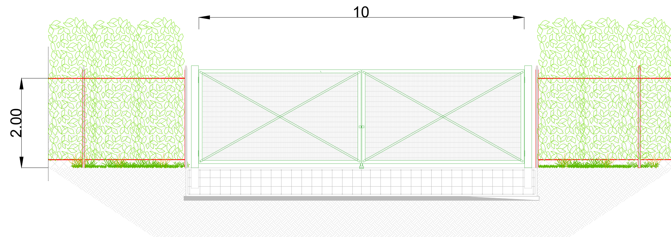
SEZIONE 2 - CANCELLO DI INGRESSO
