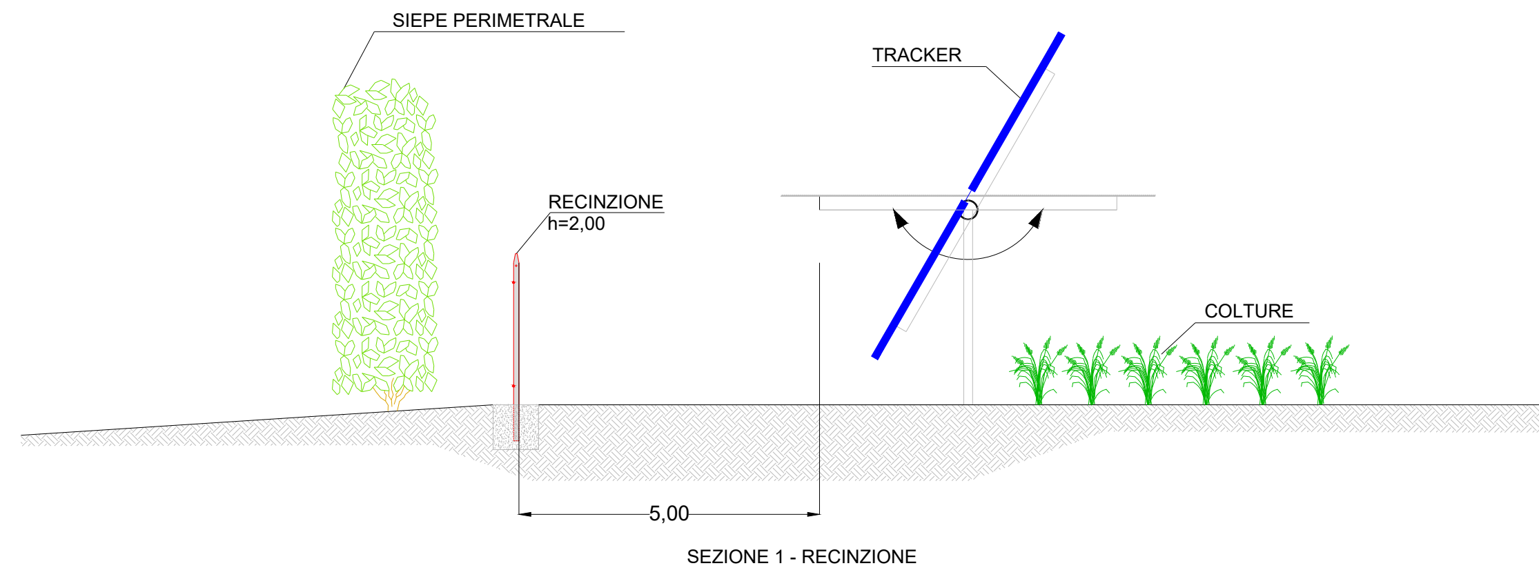
SEZIONE 1 - RECINZIONE
