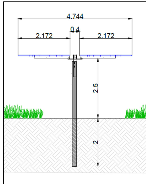
Prospetto laterale del Tracker in posizione orizzontale
