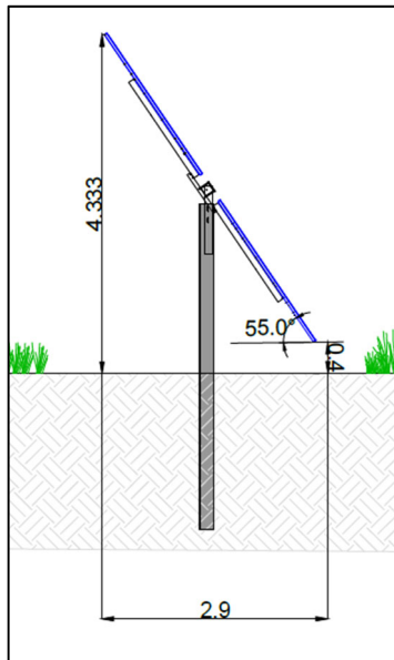
Prospetto all'inclinazione massima
