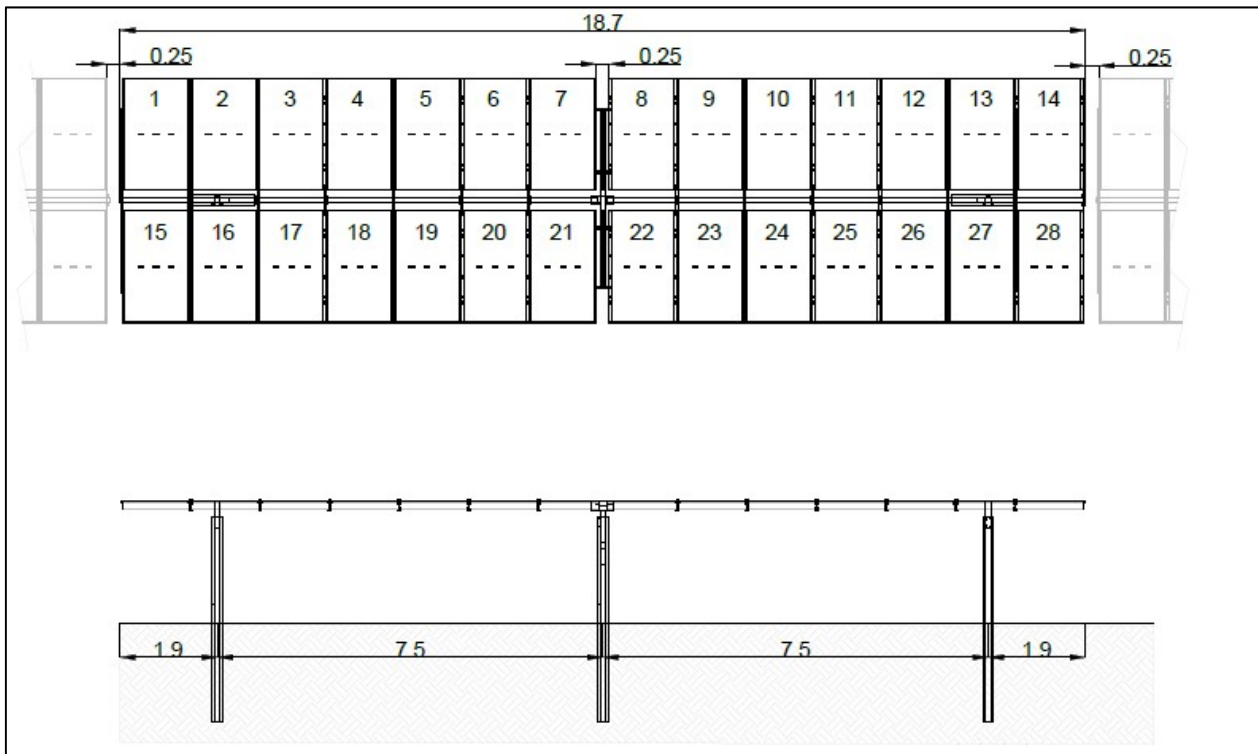
Prospetto frontale e pianta del Tracker
