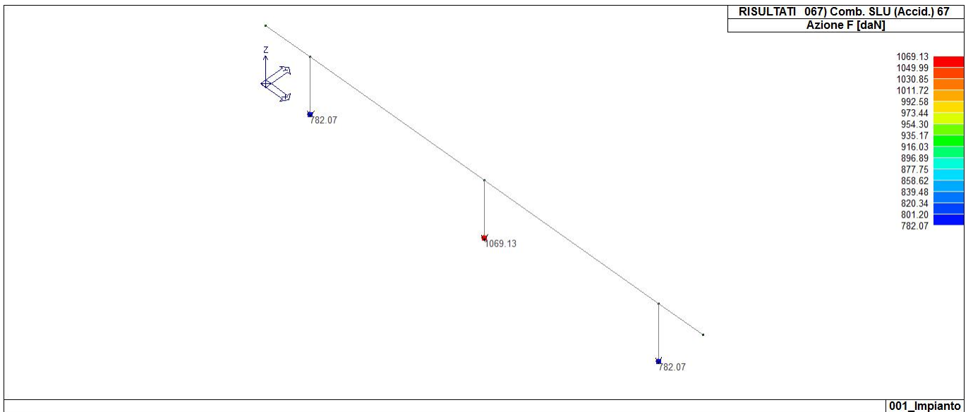
42_RIS_REAZIONI_067_Comb. SLU (Accid.) 67
