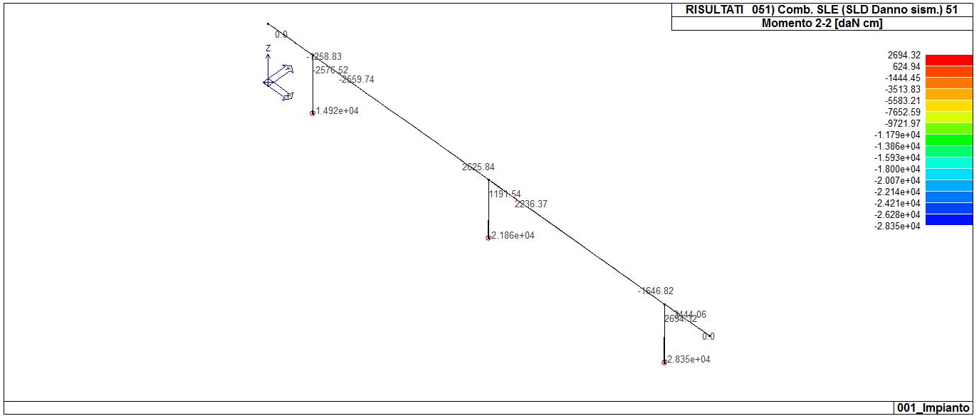
43_RIS_M2_051_Comb. SLE (SLD Danno sism.) 51
