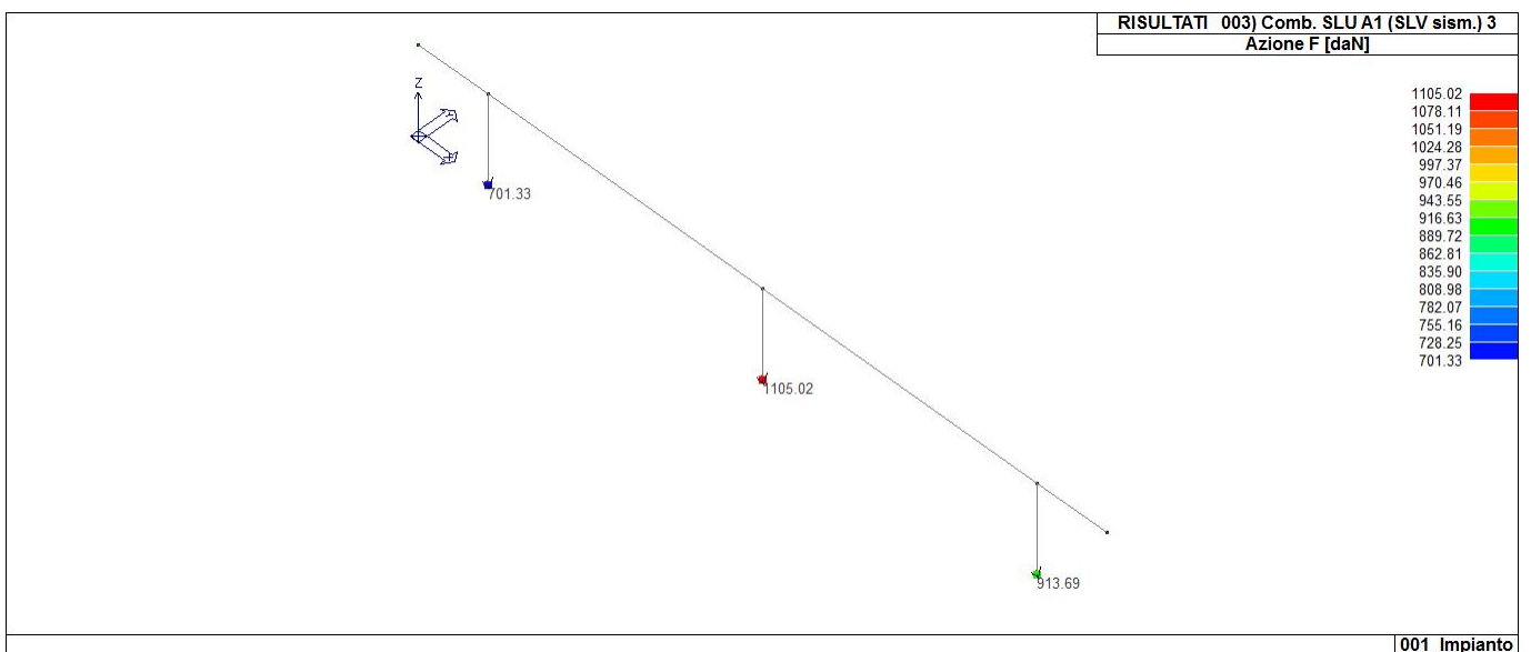
42_RIS_REAZIONI_003_Comb. SLU A1 (SLV sism.) 3
