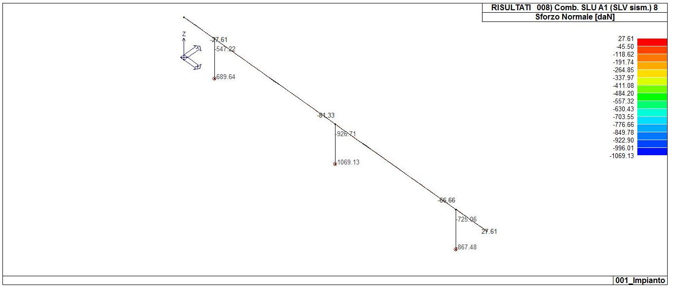
43_RIS_N_008_Comb. SLU A1 (SLV sism.) 8
