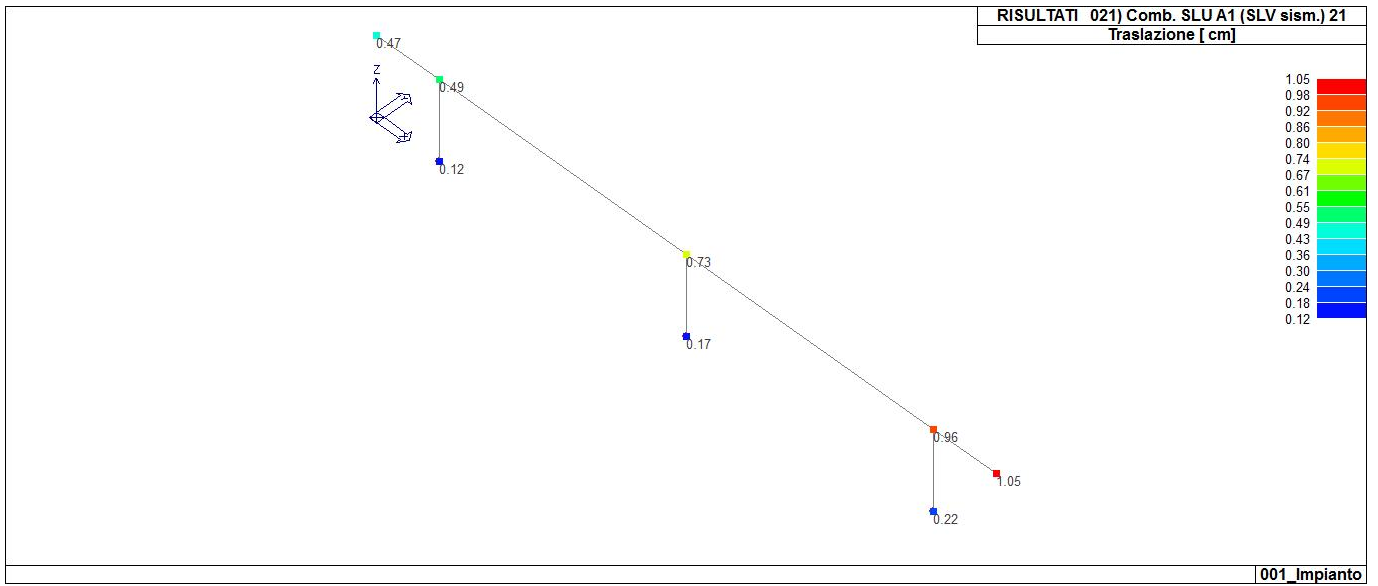
41_RIS_SPOSTAMENTI_021_Comb. SLU A1 (SLV sism.) 21
