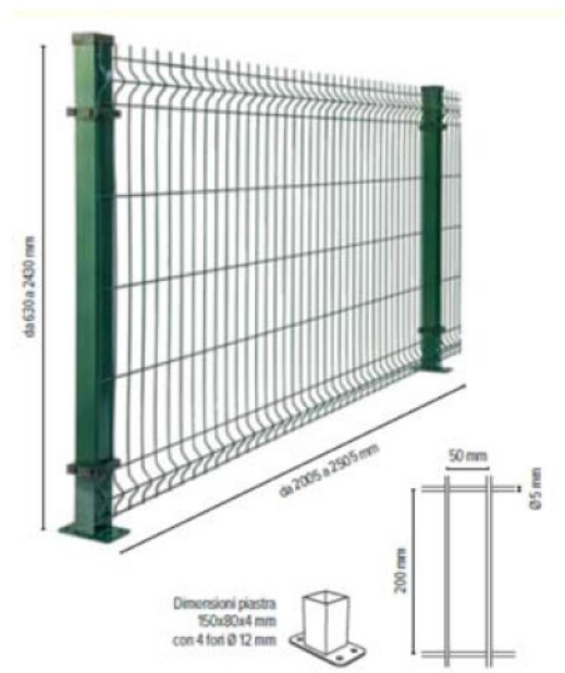
Tipologico di pannello della recinzione perimetrale
