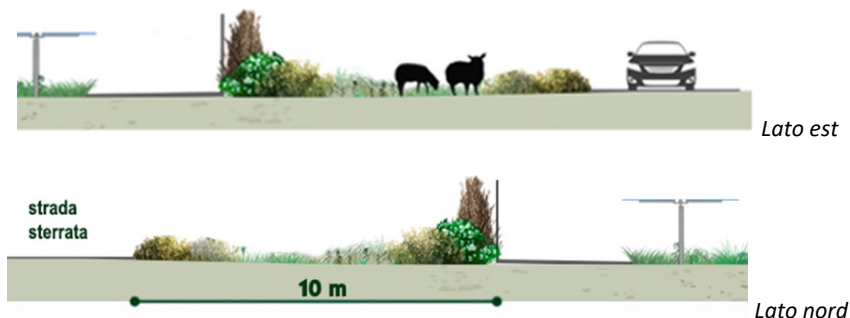
Sezioni rappresentative della fascia di rispetto di 10 m (lato est e nord)
