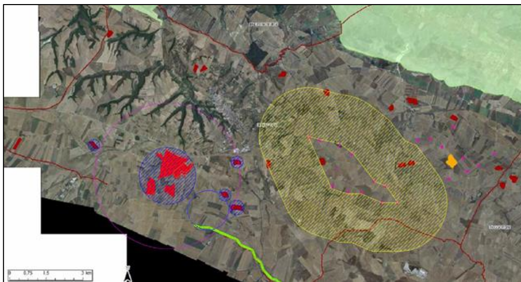
Figura 2: Impianti fotovoltaici ed eolici presenti nel SIT regionale ed oggetto della valutazione cumulativa con definizione del raggio di visibilità teorica di 3 Km (cerchio blu)
