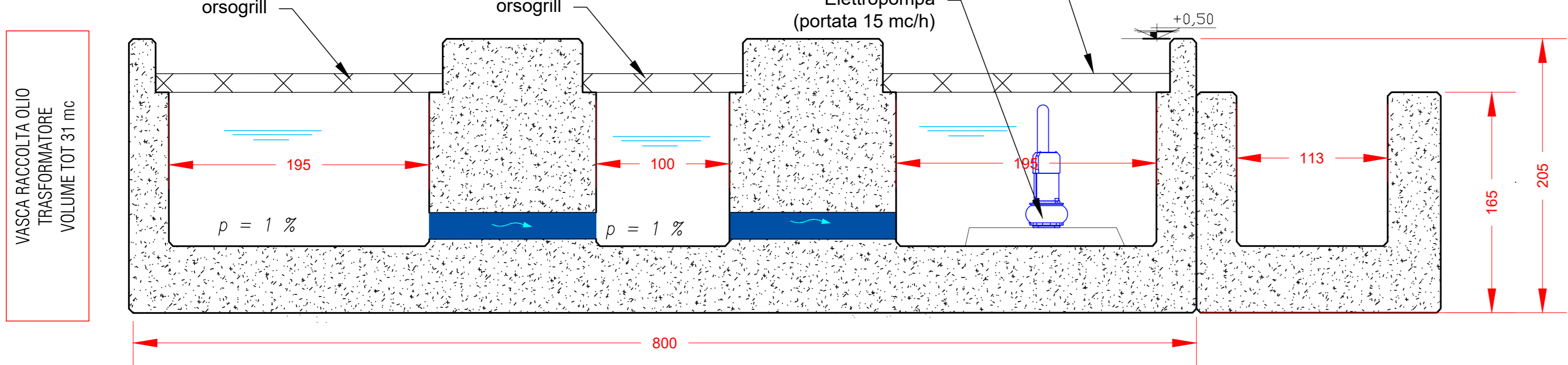
SCALA 1:50 IMPIANTO DI TRATTAMENTO
