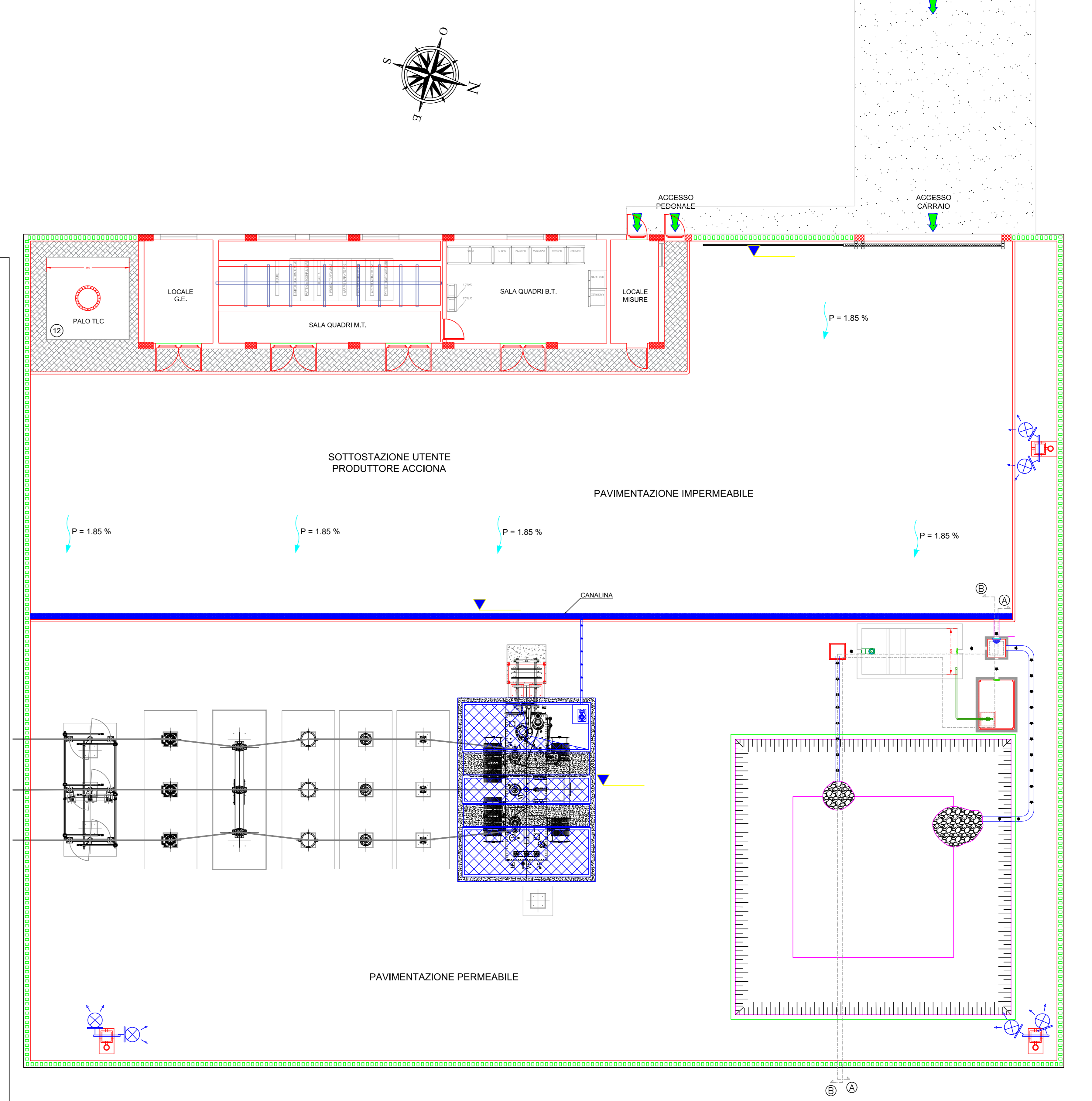
SCALA 1:100
