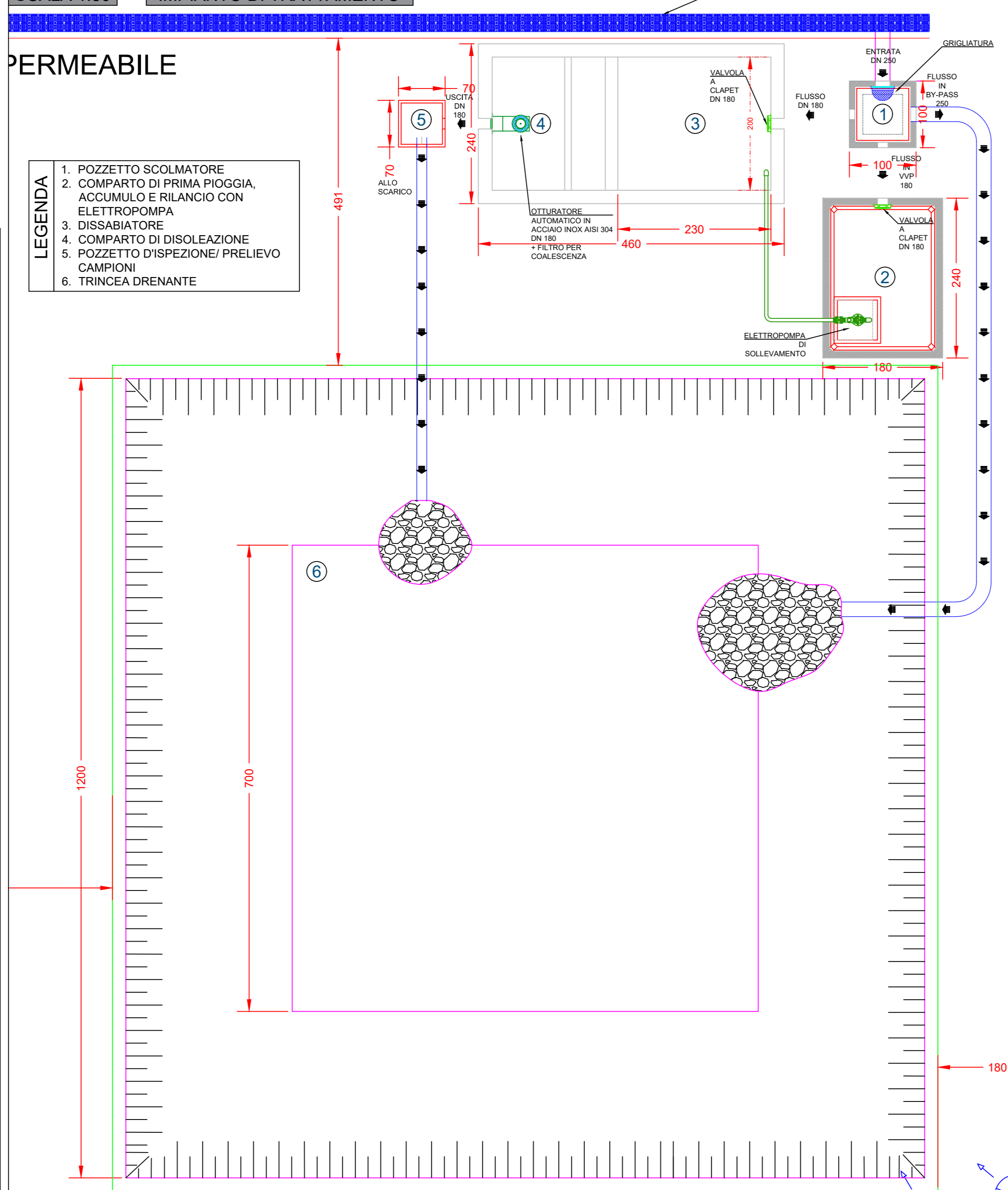
SCALA 1:50 IMPIANTO DI TRATTAMENTO
