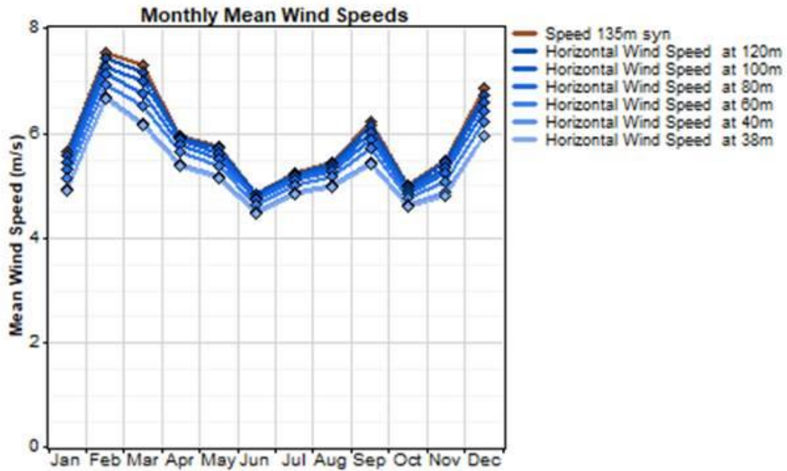
Figura 9: Profilo medio mensile di velocità del vento elaborato ad altezza mozzo
