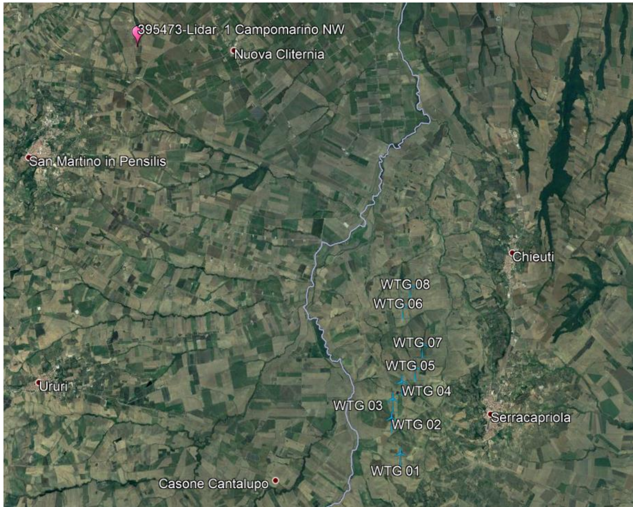
Figura 3: Posizione della Sensore Lidar rispetto all'impianto
