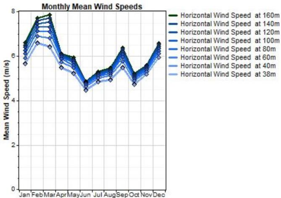
Figura 4: Lidar - Profilo medio mensile di velocità del vento a diverse altezze
