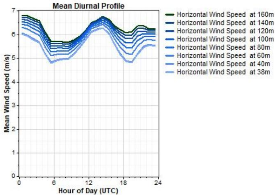
Figura 6: Lidar – Profilo medio diurno del vento
