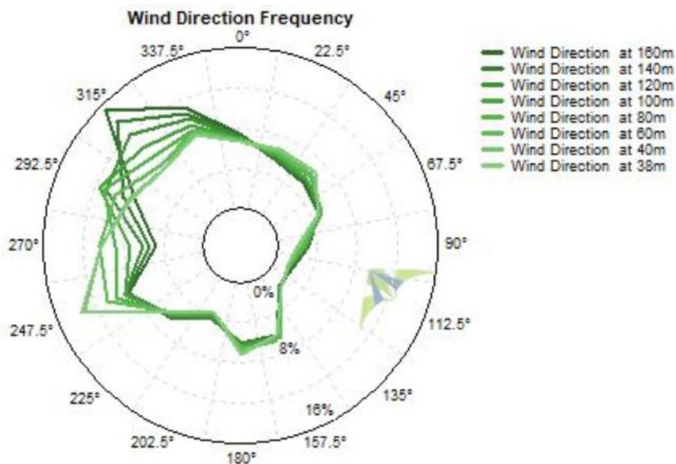
Figura 5: Lidar - Direzione prevalente del vento a diverse altezze
