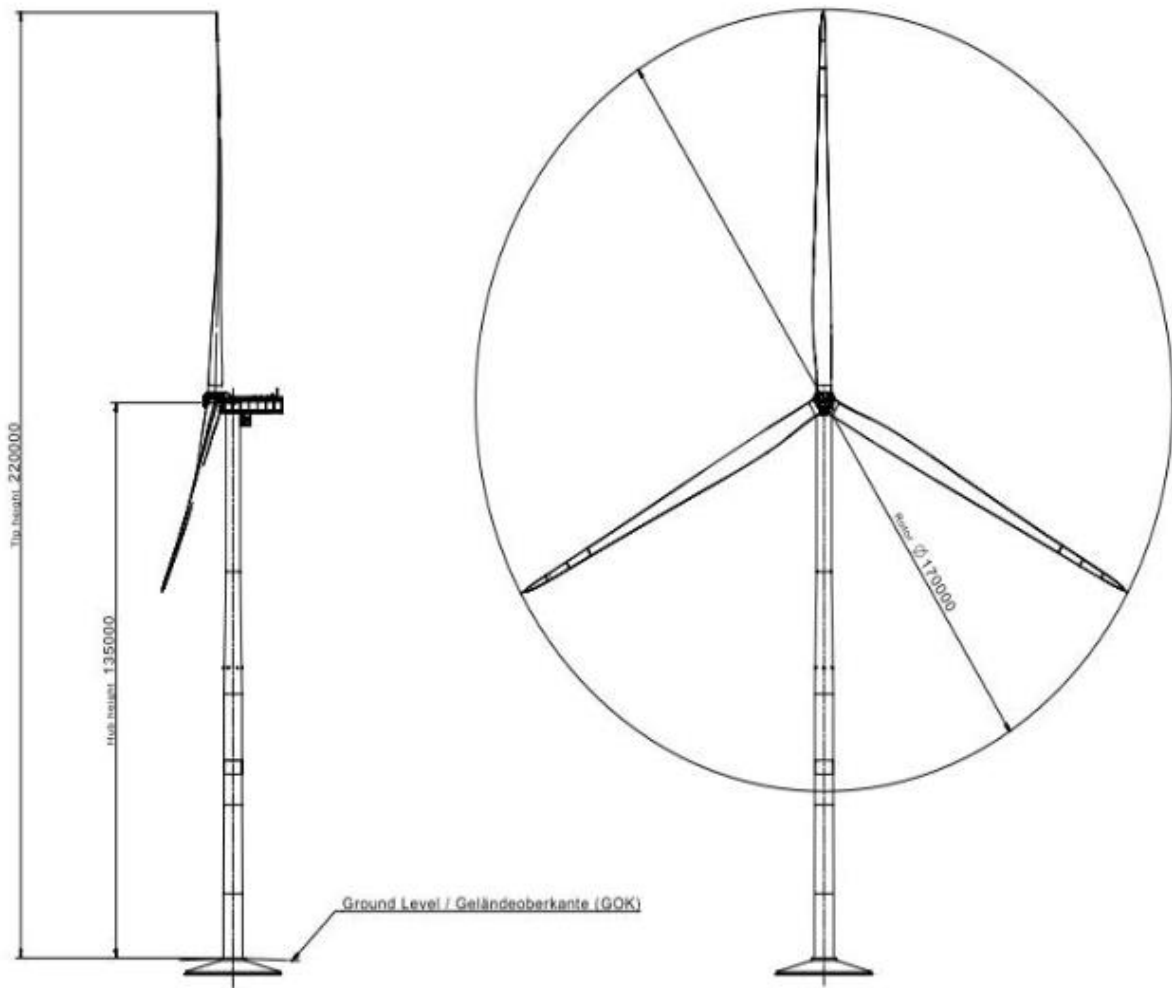
Figura 7: Vista e caratteristiche dell'aerogeneratore di riferimento
