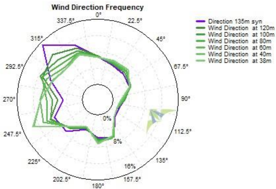
Figura 10: Direzione prevalente del vento elaborato ad altezza mozzo
