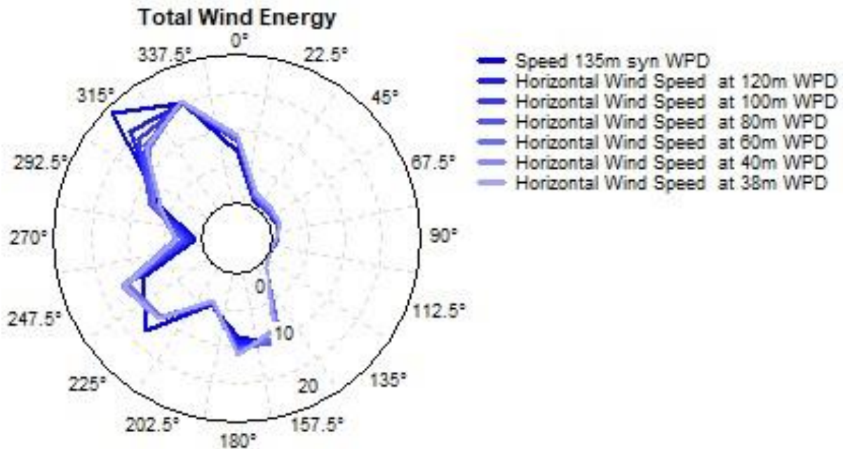
Figura 13: Energia totale del vento
