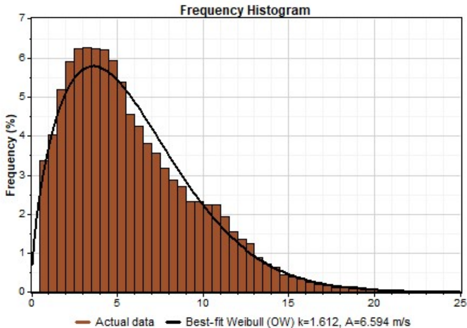
Figura 12: Distribuzione delle frequenze di Weibull
