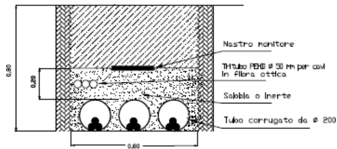
Figura 37 - Sezione su strada sterrata o terreno agricolo - posa di n°3 cavi MT
