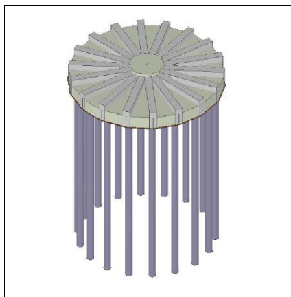
Figura 31 - Vista assometrica della struttura di fondazione
