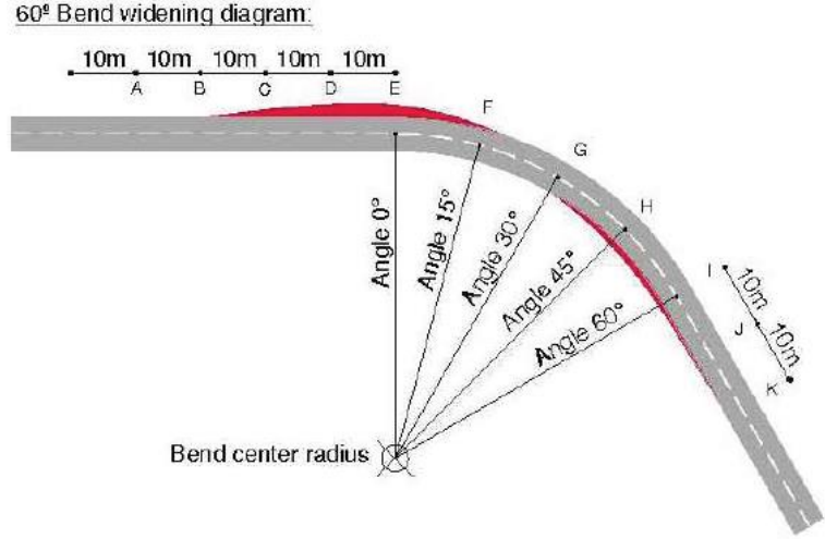
Figura 28 - Curvatura tipo con angolo di 60°
