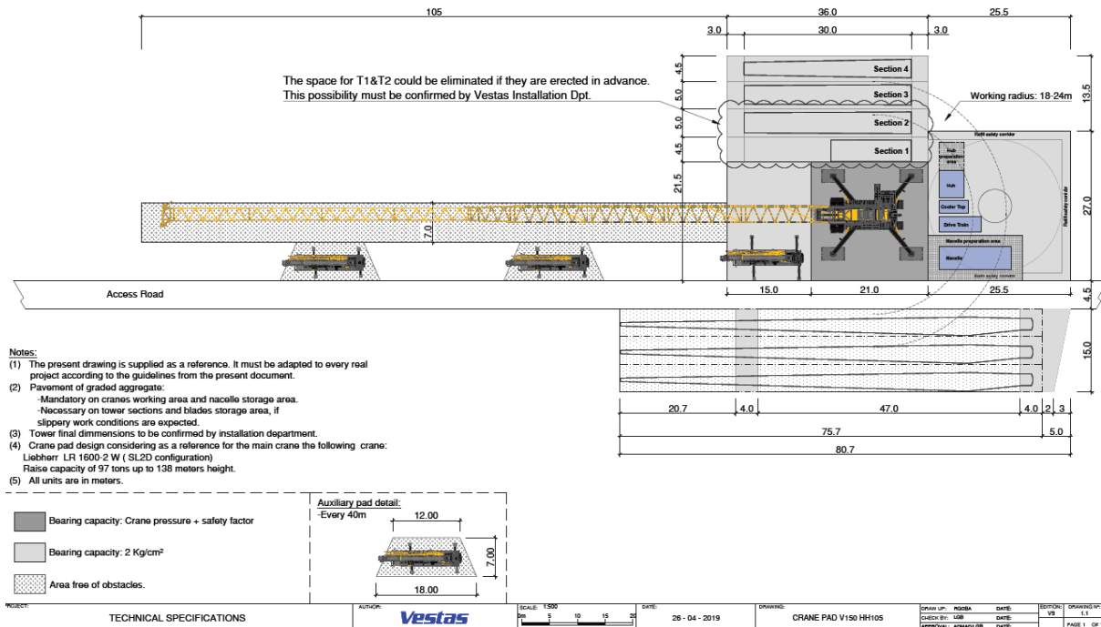
Figura 34 - schema piazzola
