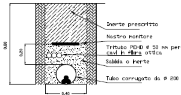
Figura 35 - Sezione su strada sterrata o terreno agricolo - posa di n°1 cavi MT
