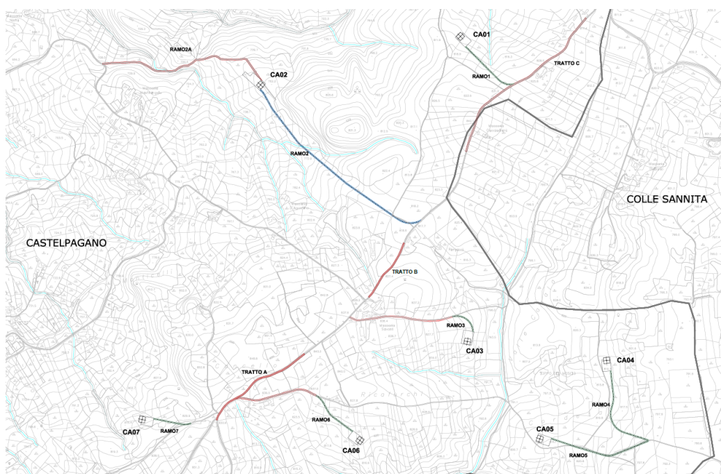
Figura 8 Viabilità interna al parco eolico (in verde i tratti di nuova costruzione, in blu le strade a carattere temporaneo ed in rosso i tratti da adeguare)
