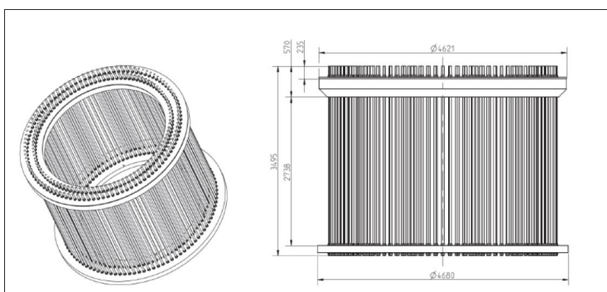
Figura 30 - Esempio di virola di fondazione
