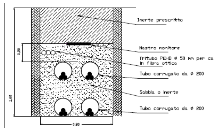
Figura 38 - Sezione su strada sterrata o terreno agricolo - posa di n°4 cavi MT
