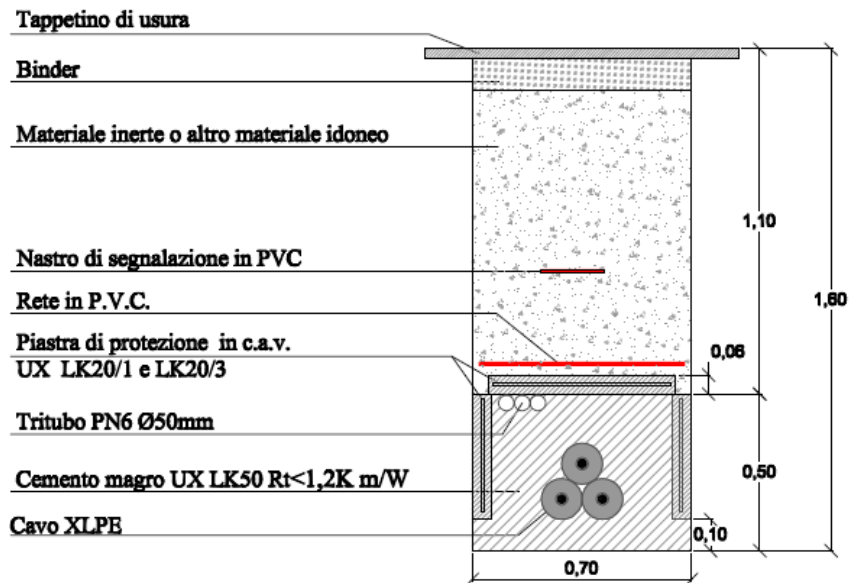
Figura 40: modalità di posa cavo 150 kV in AT posato a trifoglio nella sede stradale - sezione tipo W
