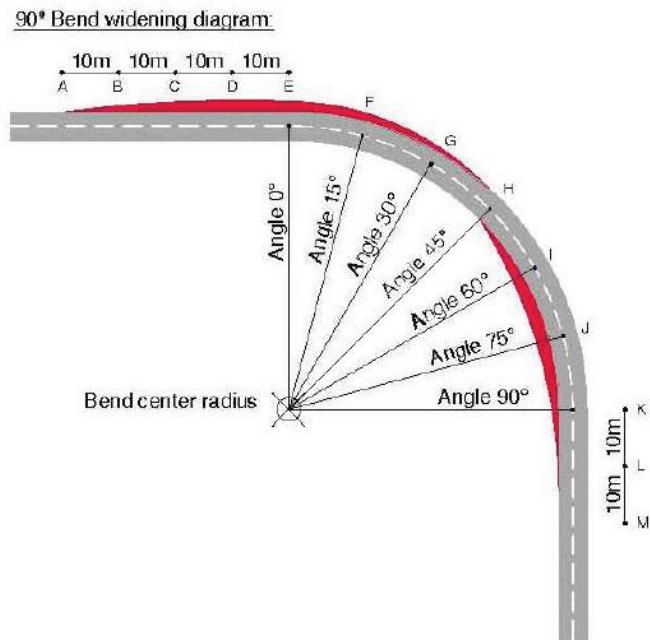
Figura 29 - Curvatura tipo con angolo di 90°
