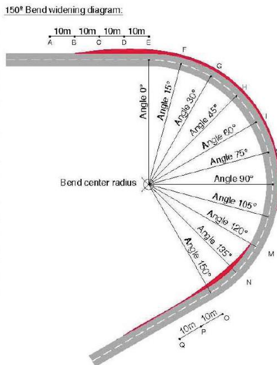
Figura 29 - Curvatura tipo con angolo di 150°
