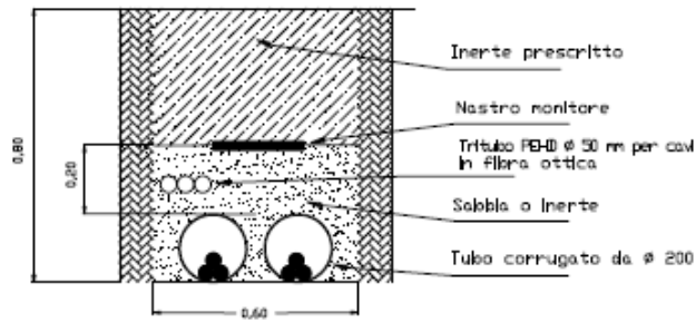
Figura 36 - Sezione su strada sterrata o terreno agricolo - posa di n°2 cavi MT
