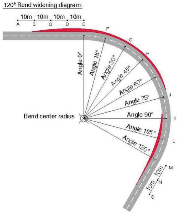
Figura 27 - Curvatura tipo con angolo di 120°
