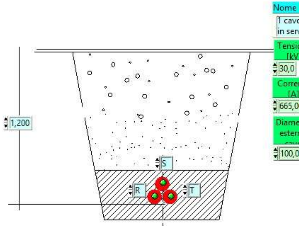
Fig. 1- Primo tratto circuito A - gruppo di tre cavi unipolari a trifoglio interrati 3 \times 1 \times 500 \text{ mm}^2 corrente in servizio normale
