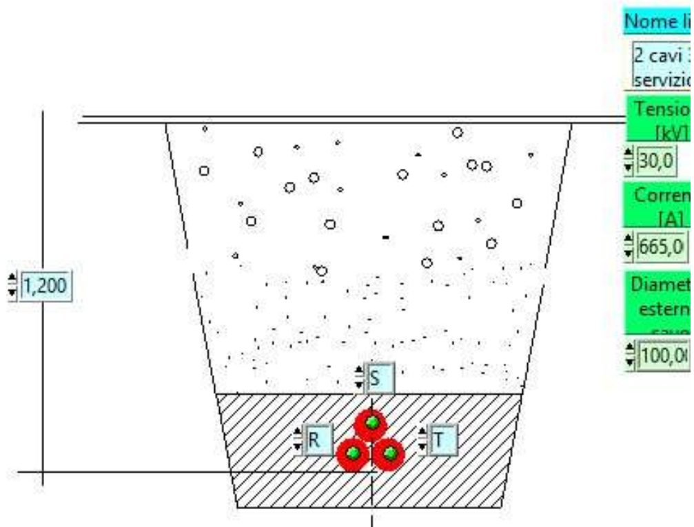
Fig. 4 - Primo tratto circuito B – due gruppi di tre cavi unipolari a trifoglio interrati: cavi 3 x 1 x 500 mm 2 corrente in servizio normale
