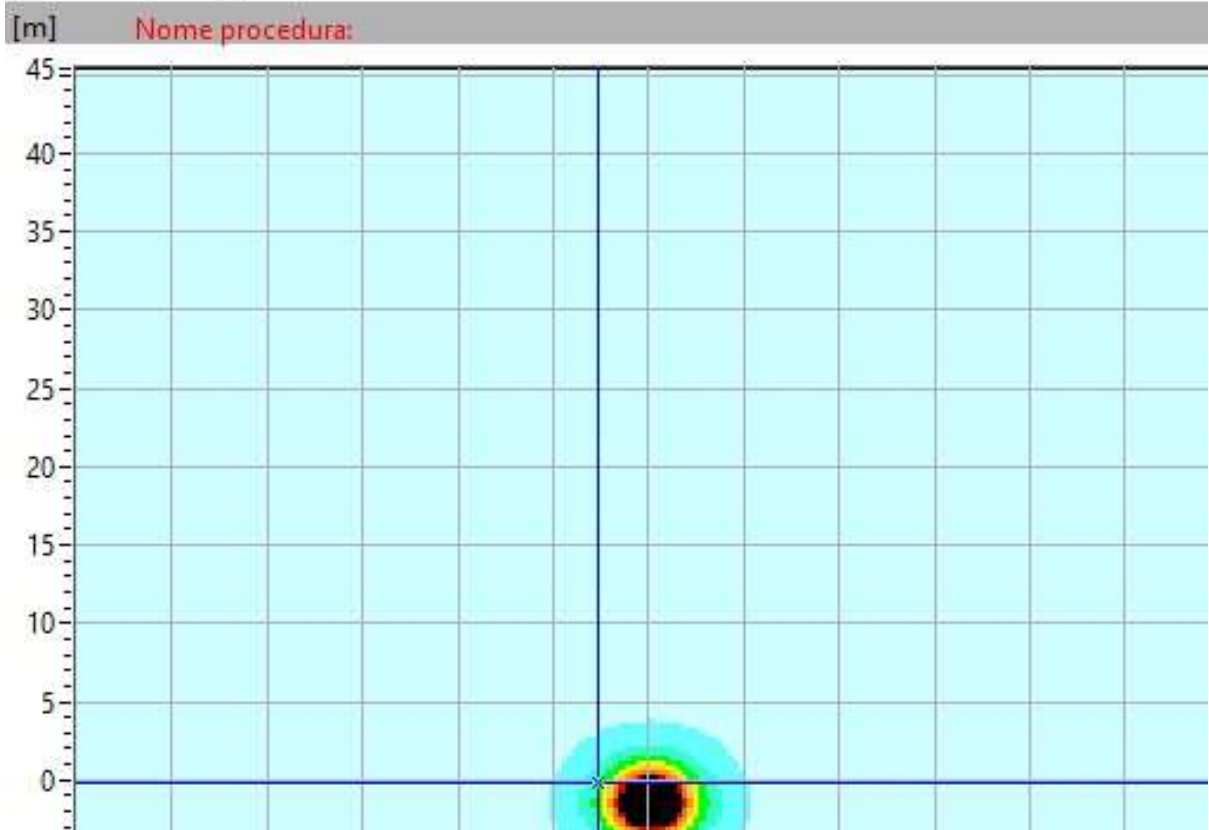
Fig. 15 – collegamento in cavo interrato a 150 kV stazione 150/30 kV – Stazione Elettrica di smistamento Terna a 150 kV di Morcone. corrente in servizio normale mappa verticale dell'induzione magnetica
