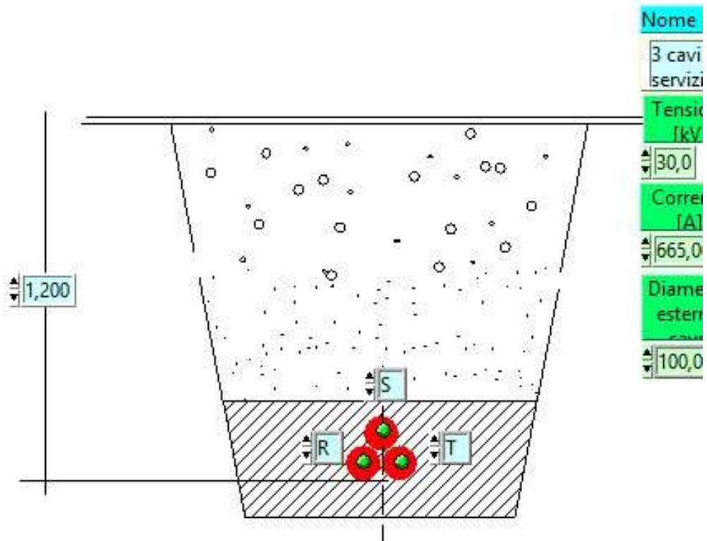
Fig. 7- Tratto in comune circuito A e B affiancati - tre gruppi di tre cavi unipolari a trifoglio interrati: cavi 3 x 1 x 500 mm 2 corrente in servizio normale
