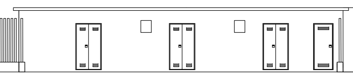
PROSPETTO ANTERIORE LOCALI QUADRI BT
