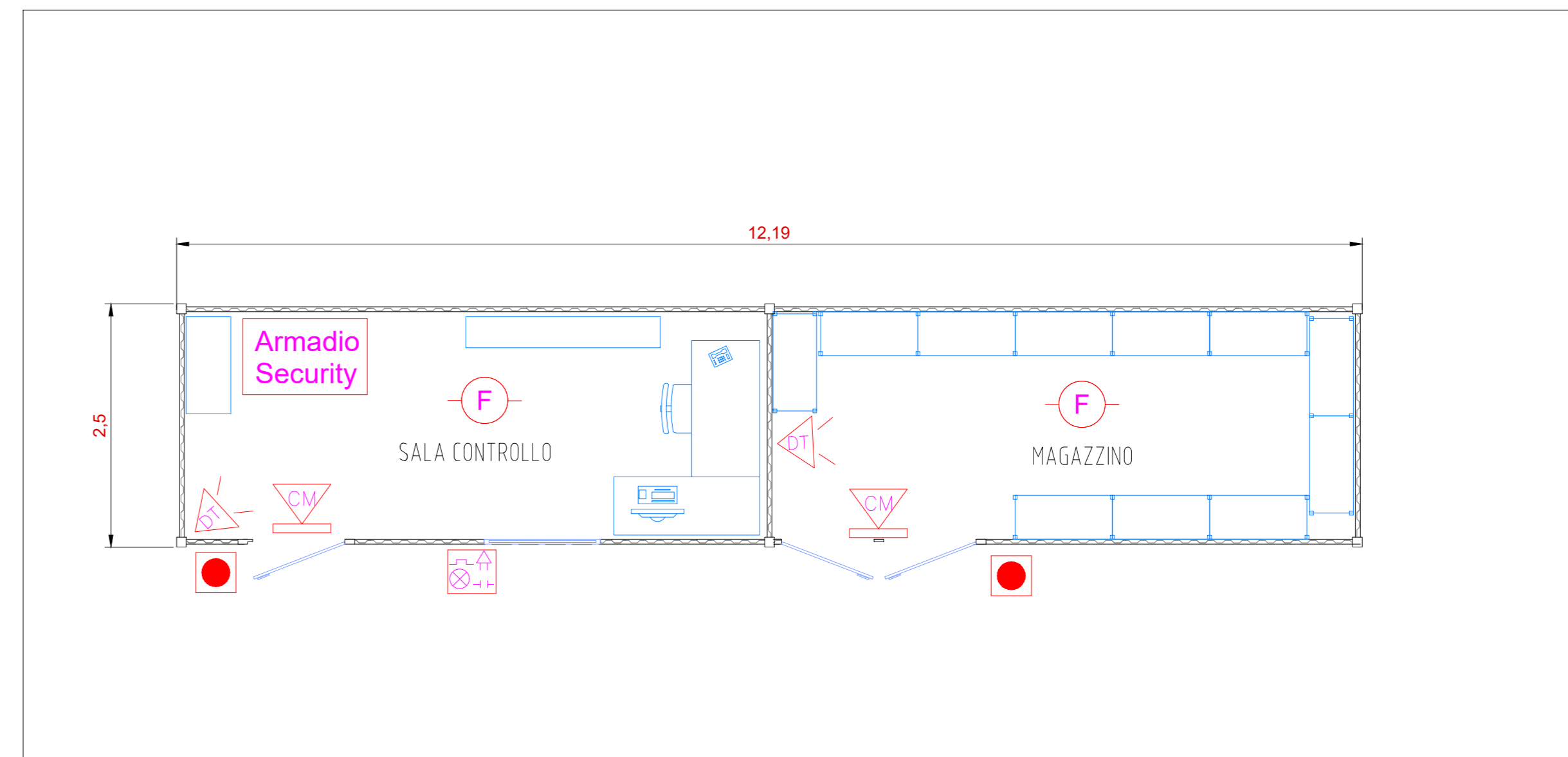
Layout impianto Vista C - Area 2 - scala 1:2000
