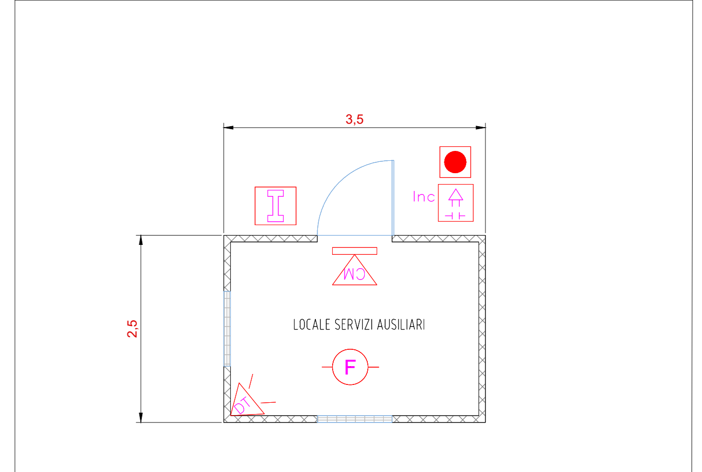
PARTICOLARE PLANIMETRICO - TIPICO POWER STATION - SCALA 1:50
