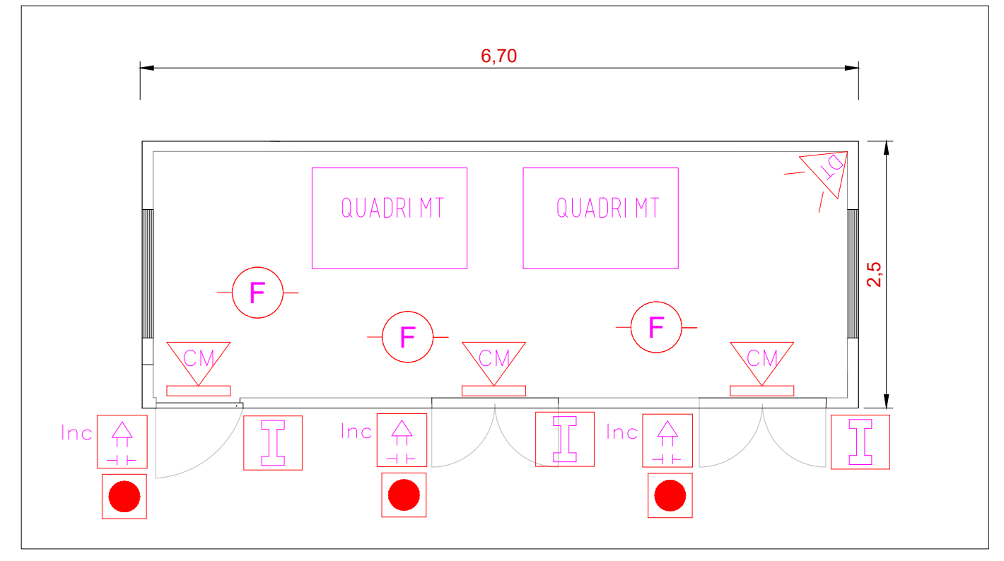
PARTICOLARE PLANIMETRICO - TIPICO CABINA RACCOLTA MT - SCALA 1:50
