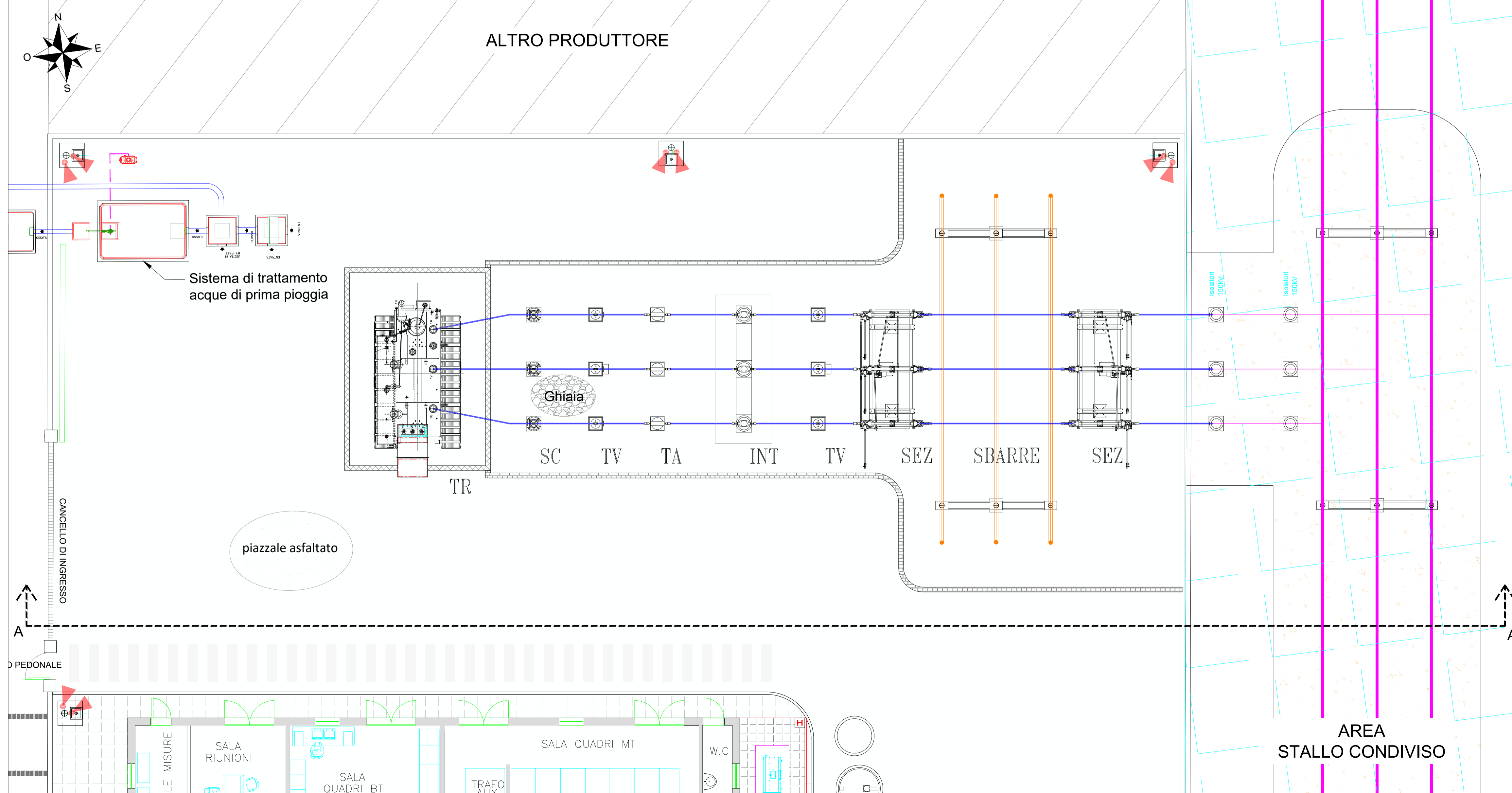
Planimetria elettromeccanica Stazione Utente - Scala 1:100
