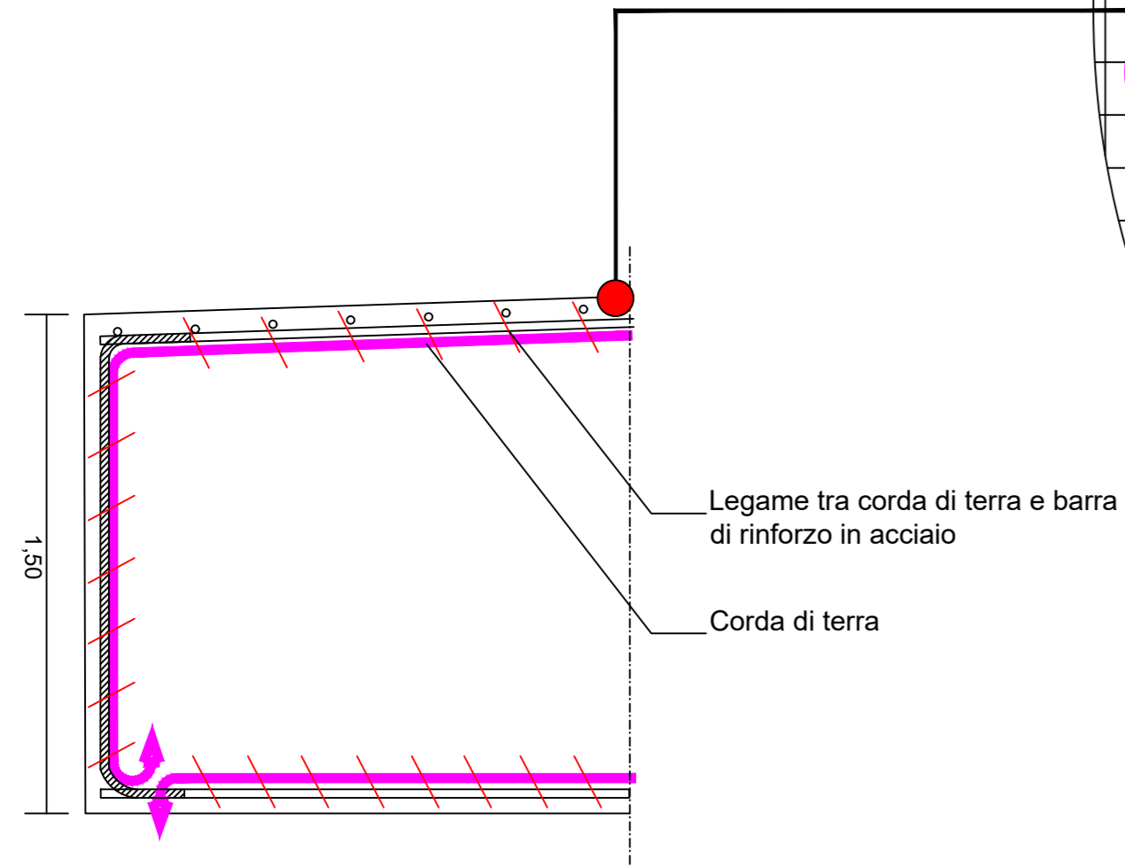
Particolare 2 scala 1:20
