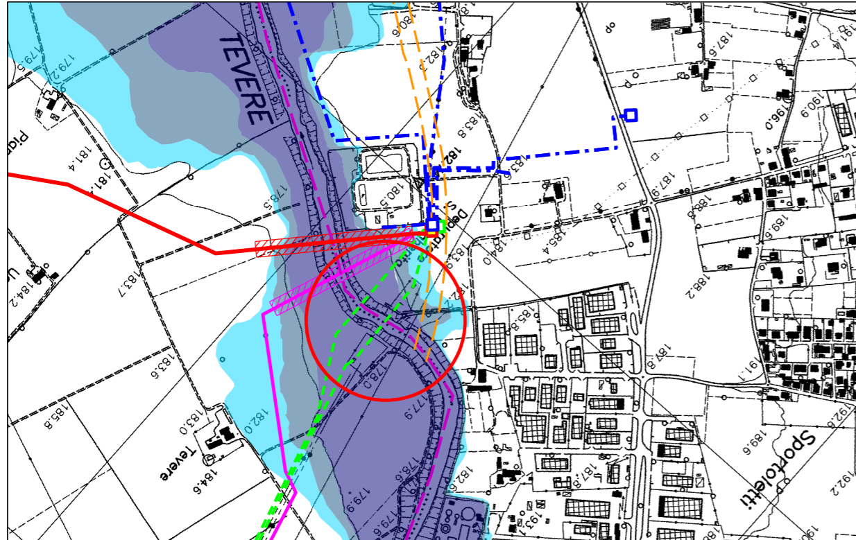
PIANO DI ASSETTO IDROGEOLOGICO
