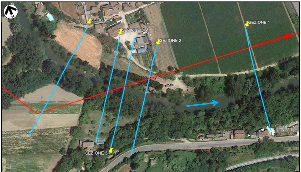
Figura 4.4.2/A – Planimetria del tratto di corso modellato con sezioni rilevate (in rosso tracciato del metanodotto)
