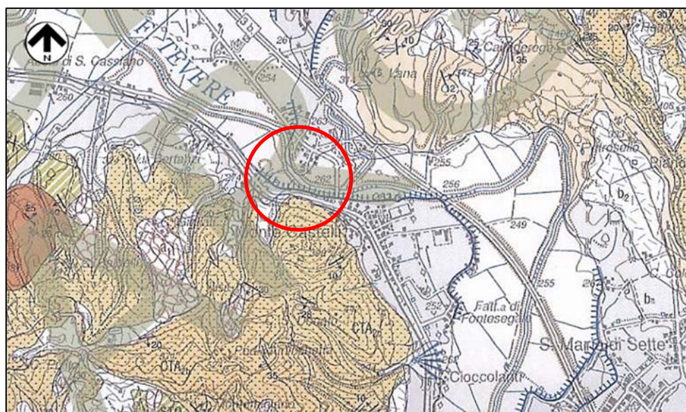
Figura 3.2/A – Stralcio carta geologica CARG 299 con localizzazione della sezione di attraversamento
