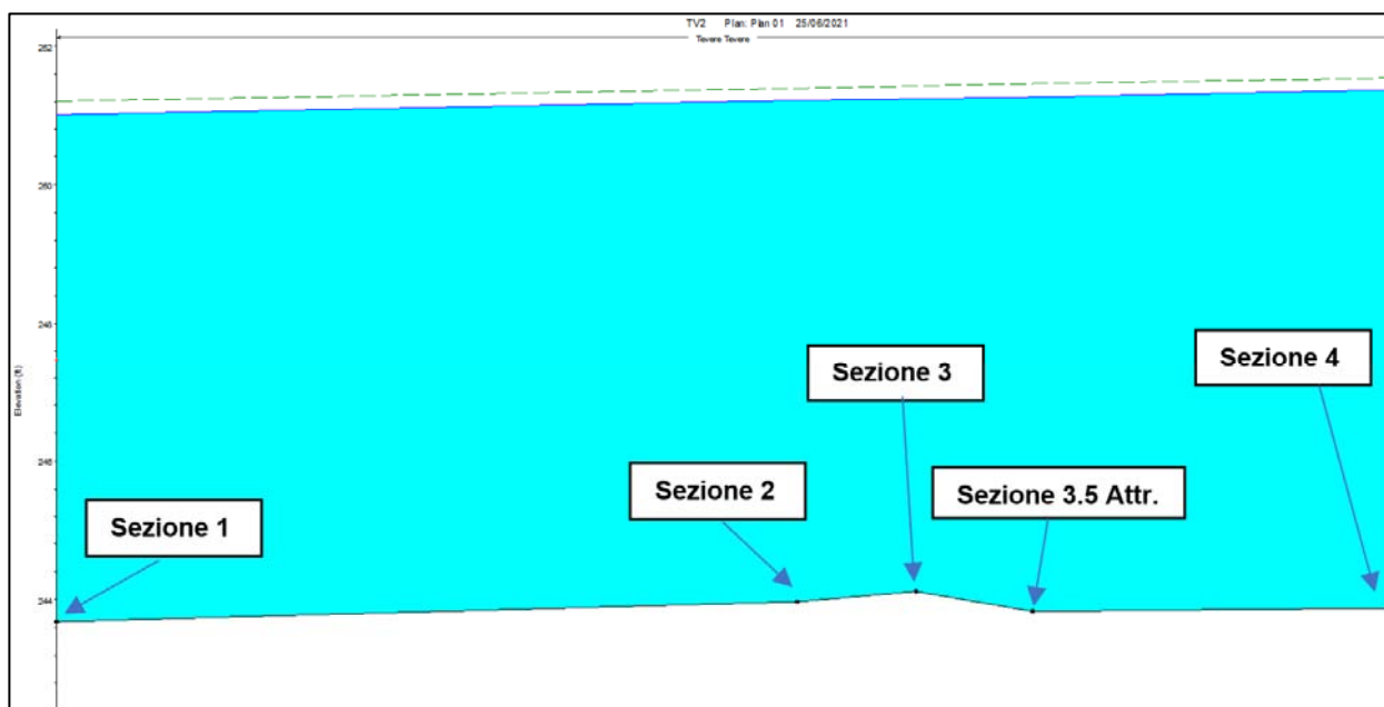
Figura 4.3.3/A – Profilo longitudinale con livello di piena duecentennale
