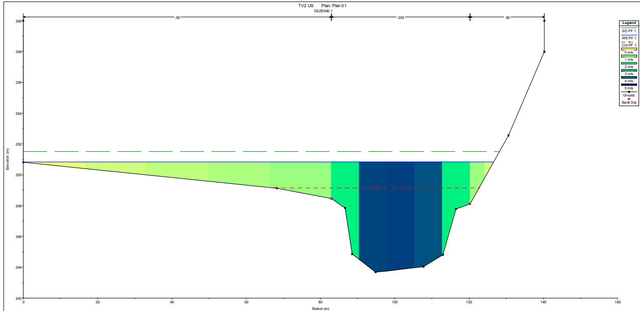
Sezione 1
