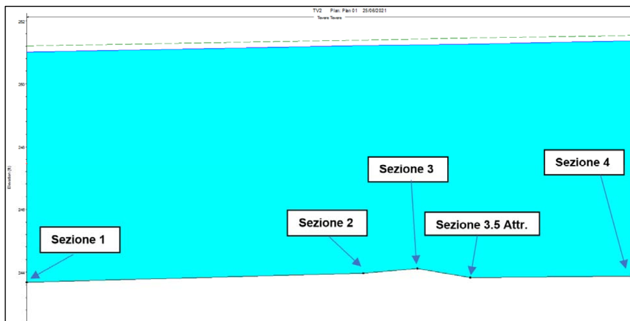
Figura 4.3/B – Sezione longitudinale con profilo di piena duecentennale
