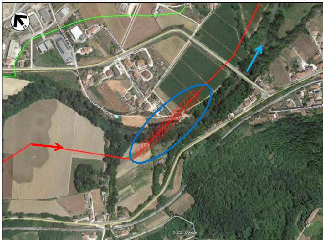
Figura 2/C – Immagine aerea con localizzazione della sezione di attraversamento (su base Google Earth)
