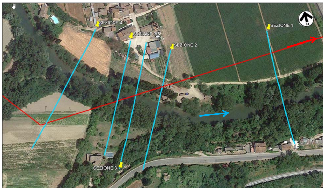
Figura 4.2/A – Planimetria del tratto di corso modellato, con ubicazione delle sezioni di modellazione (in rosso tracciato del metanodotto)
