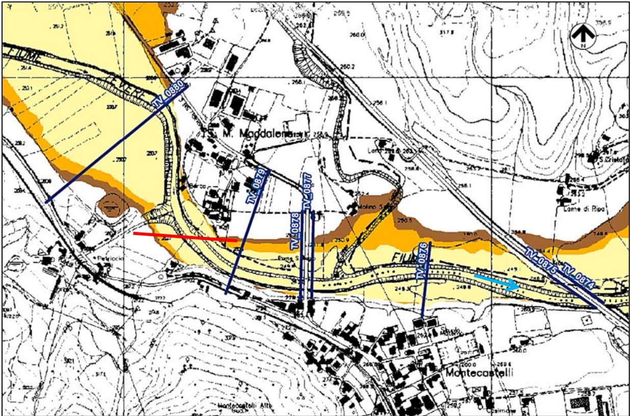
Figura 3/B – Stralcio della mappa di pericolosità del PGRAAC (TAV. 11 P) con ubicazione delle sezioni PAI
