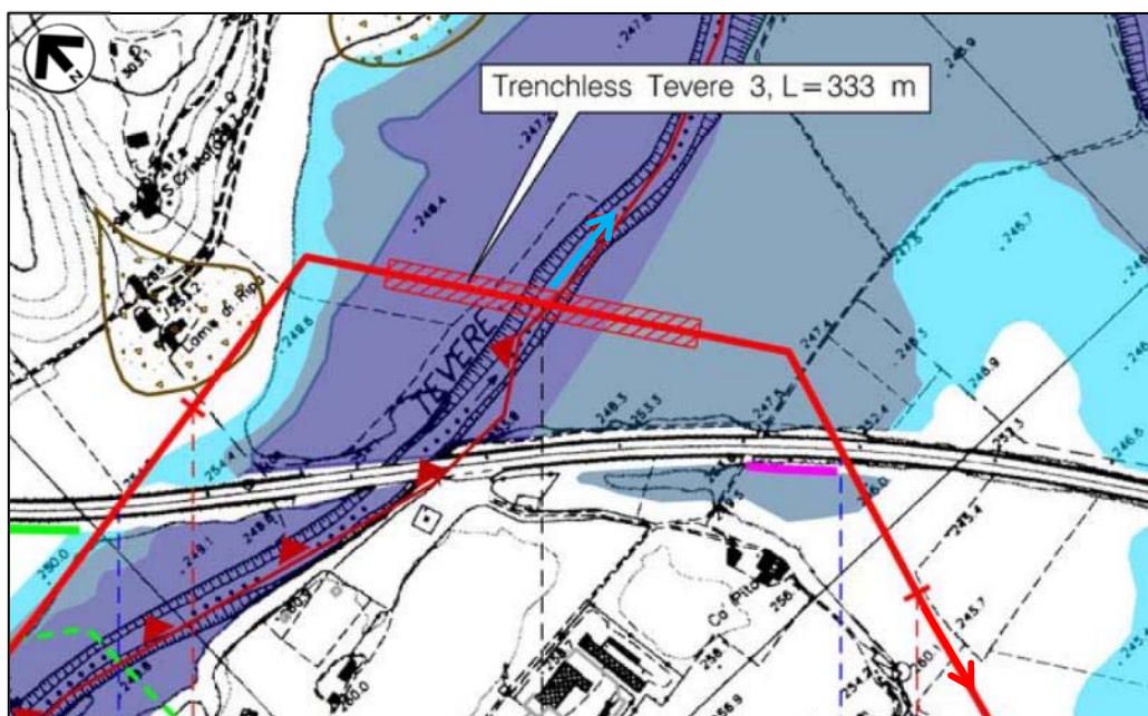
Figura 4.1/A – Situazione di pericolosità da alluvione nel tratto di attraversamento (da mappe di pericolosità PRGAAC, ridisegnato)
