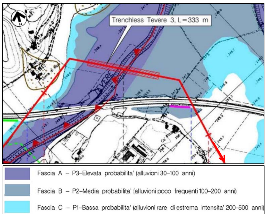
Figura 6.1/A – Situazione di pericolosità da alluvione nel tratto di attraversamento (da mappe di pericolosità PRGAAC, ridisegnato)
