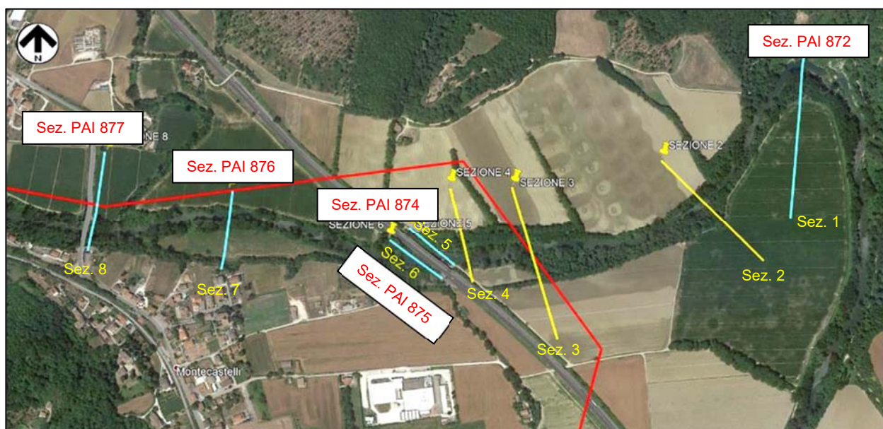
Figura 4.4.2/A – Planimetria del tratto di corso modellato con riportate le sezioni di studio (in rosso tracciato del metanodotto, in azzurro sez. tratte da PAI, in giallo sez. rilevate)
