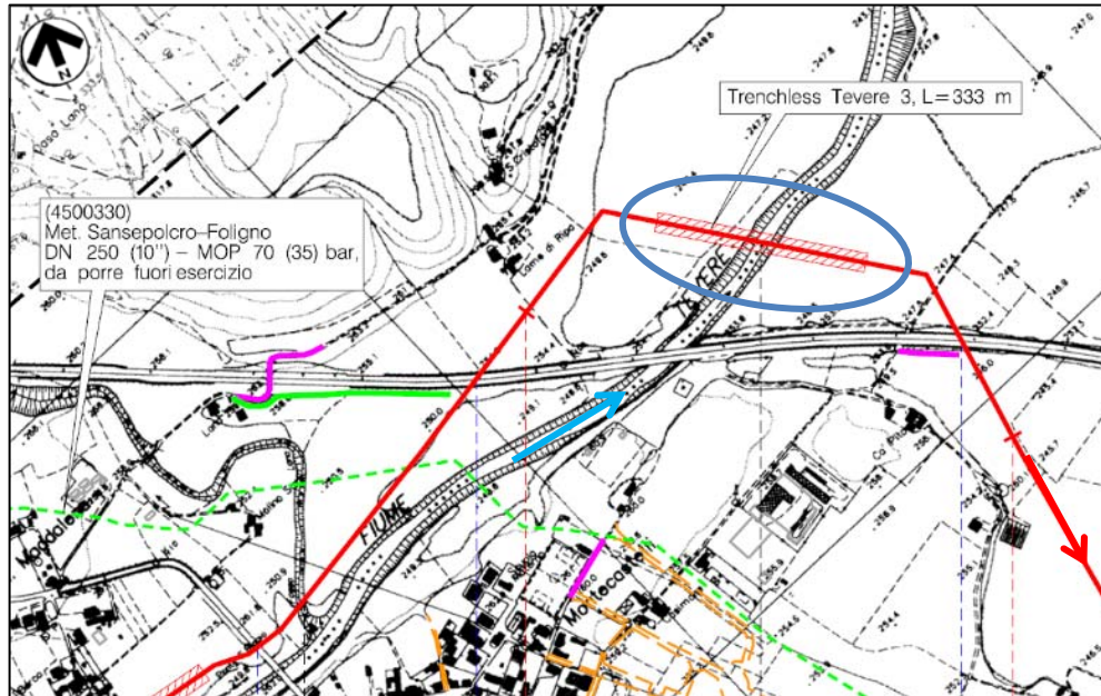
Figura 2/B – Stralcio CTR con localizzazione dell'attraversamento
