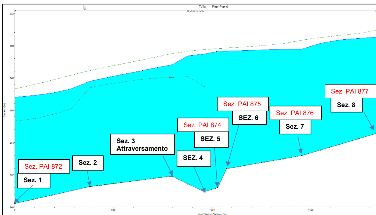
Figura 4.4.3/A – Profilo longitudinale con livelli di piena duecentennale, con indicazione delle sezioni utilizzate per la modellazione locale
