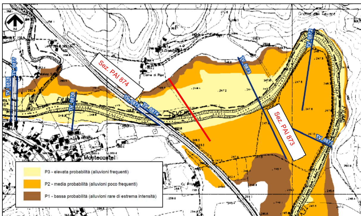
Figura 4.1/B – Stralcio della mappa di pericolosità del PRGAAC (TAV. 11 P) con ubicazione sezioni PAI (in rosso sezione di attraversamento)
