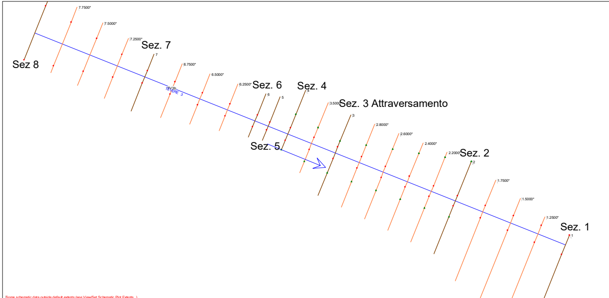
Figura 4.2/A- Schema planimetrico delle sezioni utilizzate per la modellazione (in marrone: sezioni rilevate, in rosso sezioni interpolate)
