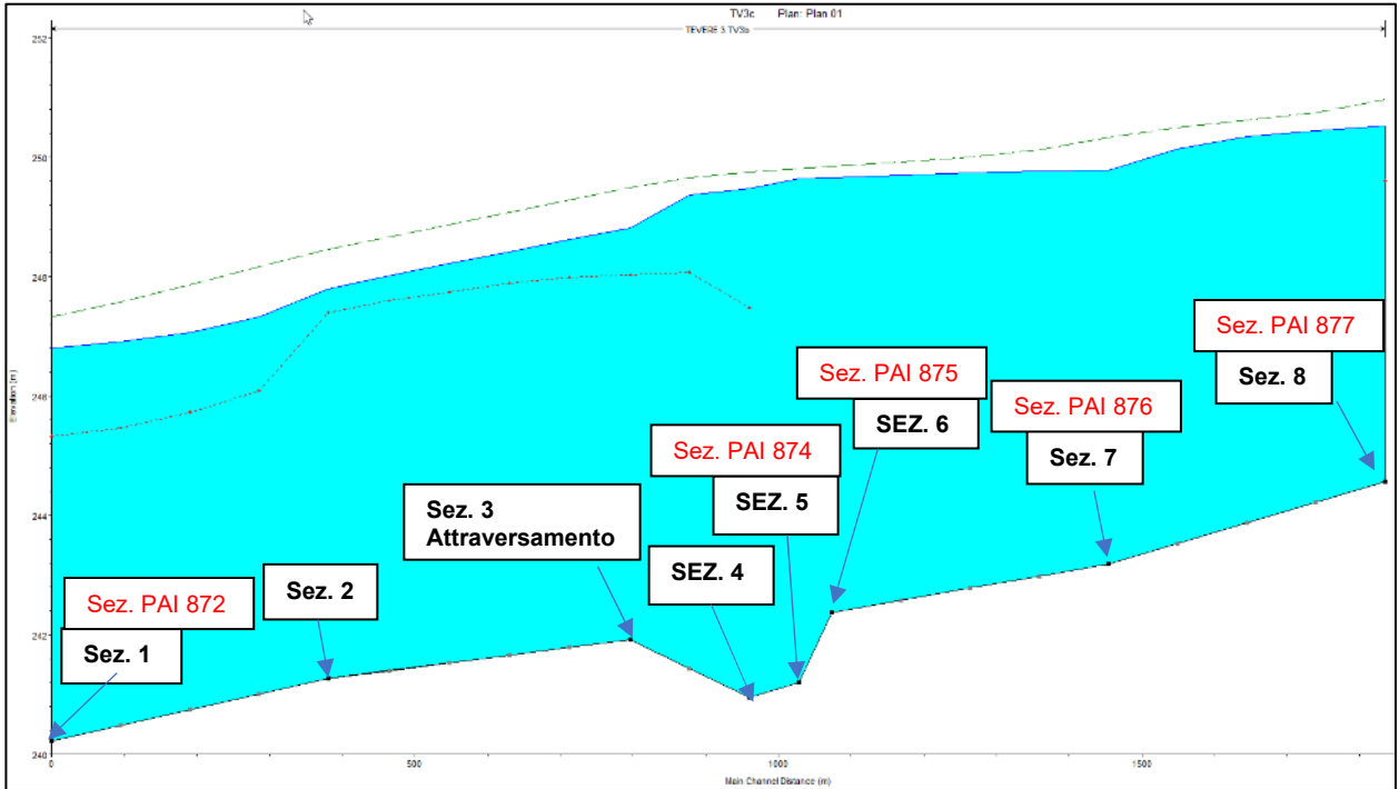
Figura 4.3/A – Profilo longitudinale con livello di piena duecentennale
