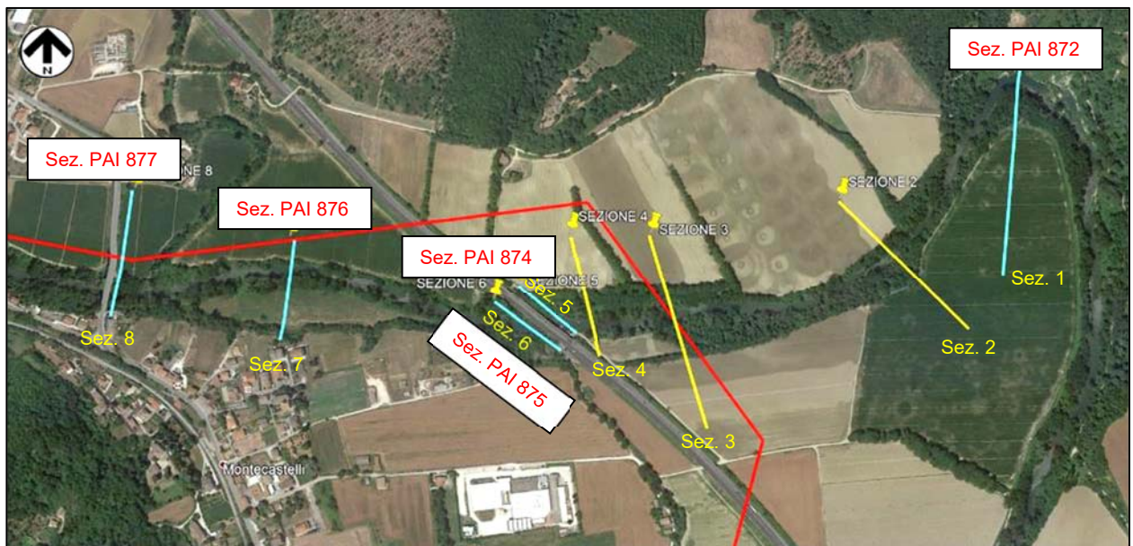
Figura 4.2/B- Planimetria del tratto di corso modellato con riportate le sezioni di studio (in rosso tracciato del metanodotto, in azzurro sez. PAI, in giallo sez. rilevate)
