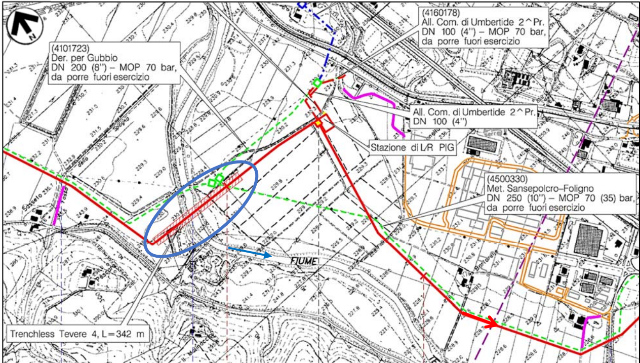
Figura 1/B – Stralcio CTR con localizzazione dell’attraversamento
