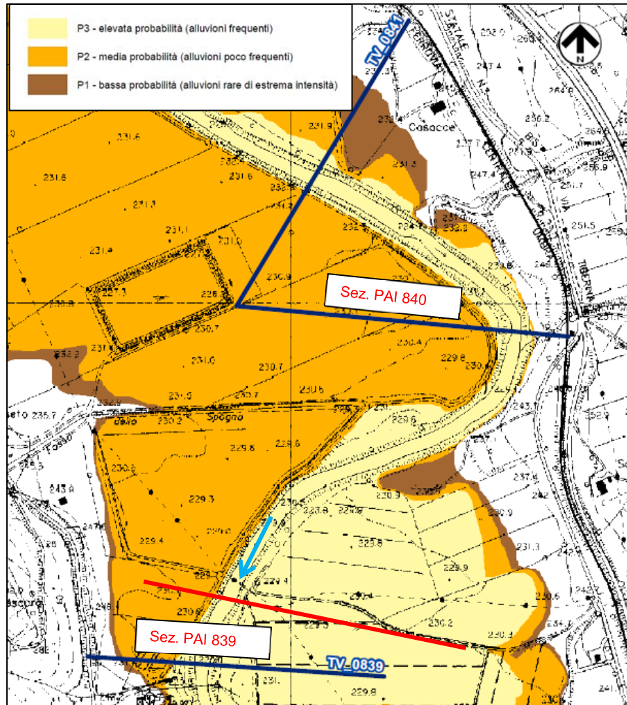
Figura 3/B – Stralcio della mappa di pericolosità del PGRAAC (TAV. 18 P) con ubicazione sezioni PAI
