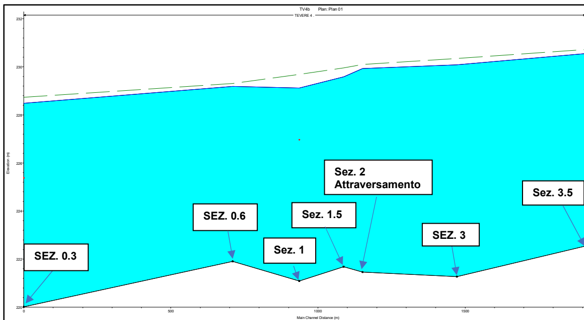
Figura 4.3/A – Profilo longitudinale con livelli di piena duecentennali
