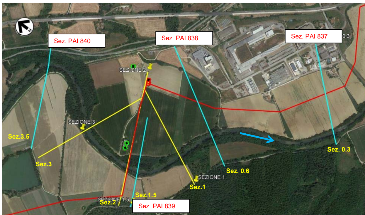
Figura 4.2/A– Immagine aerea del tratto di corso modellato con riportate le sezioni di studio (in rosso tracciato del metanodotto, in azzurro sez. PAI, in giallo sez. rilevate)
