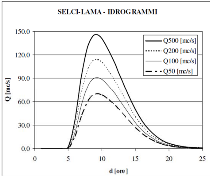
Figura 3/A – Idrogrammi e portate per la sezione di chiusura del T. Selci (da R. Umbria, Analisi Idrologiche reticolo secondario Alto Tevere)
