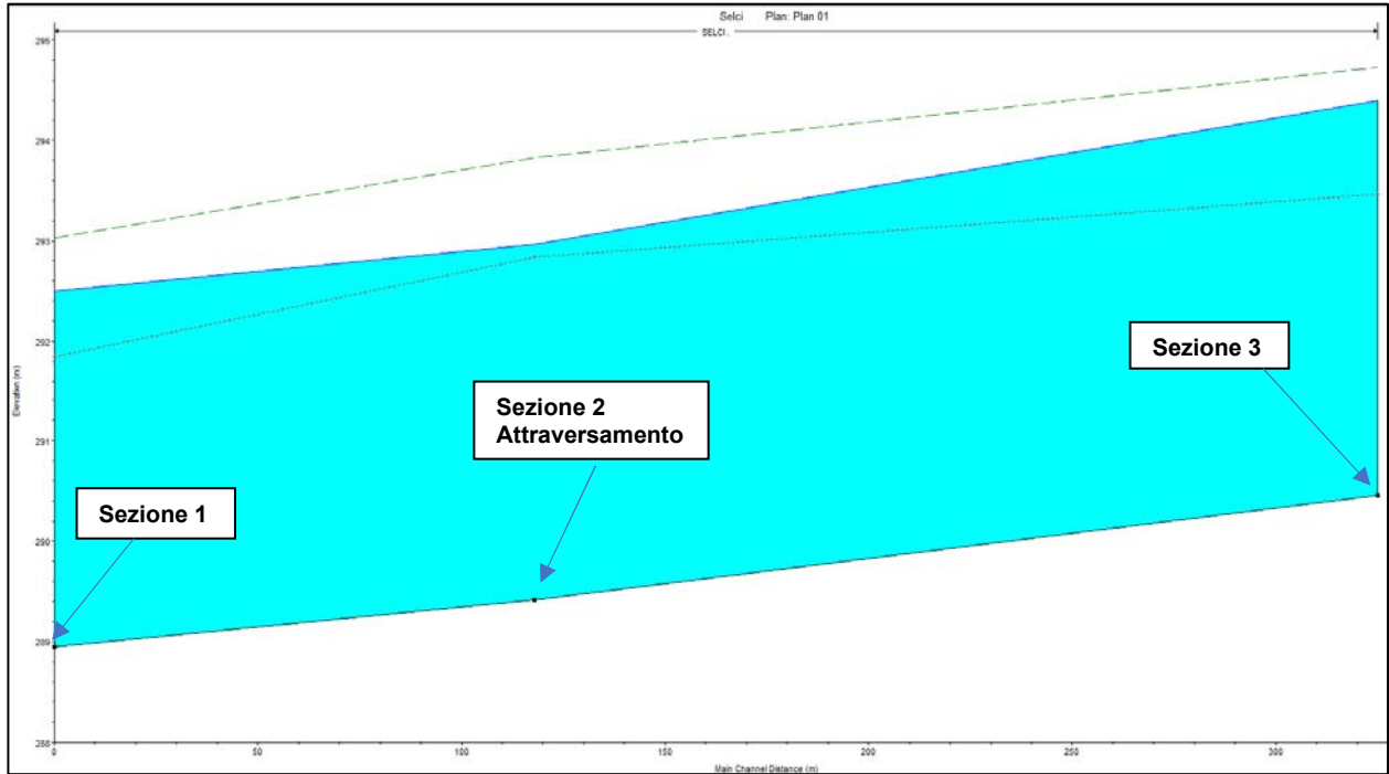
Figura 4.2/B – Profilo longitudinale in alveo con livelli idrici duecentennali
