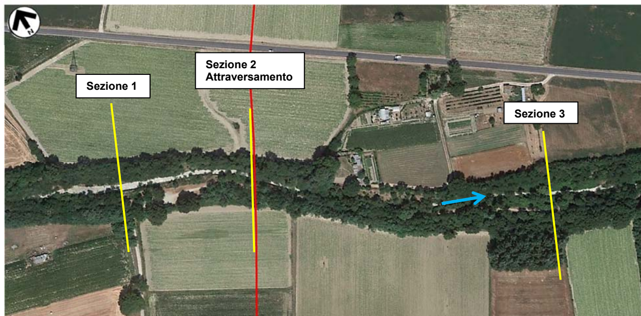
Figura 4.2/A – Planimetria del tratto di corso modellato con riportate le sezioni di studio (in rosso tracciato del metanodotto)
