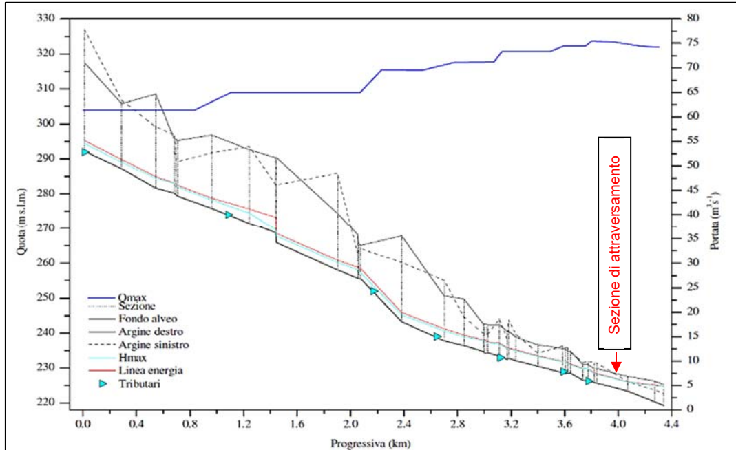
Figura 4.3/A – Involuppo dei massimi livelli calcolati per l'evento di piena con tempo di ritorno 200 anni. E' riportata anche la geometria dell'alveo.
