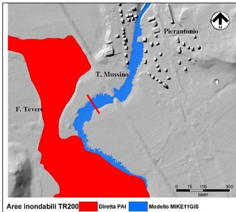
Figura 4.3/B - Mappa delle aree inondabili da parte del T. Mussino (in azzurro) per T_r=200 anni (linea rossa: sezione di attraversamento)
