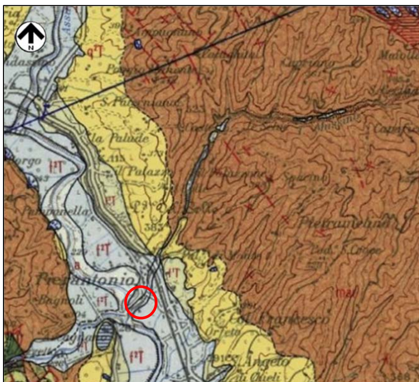
Figura 3.2/A – Stralcio della Carta Geologica d'Italia Fig. 122 Perugia
