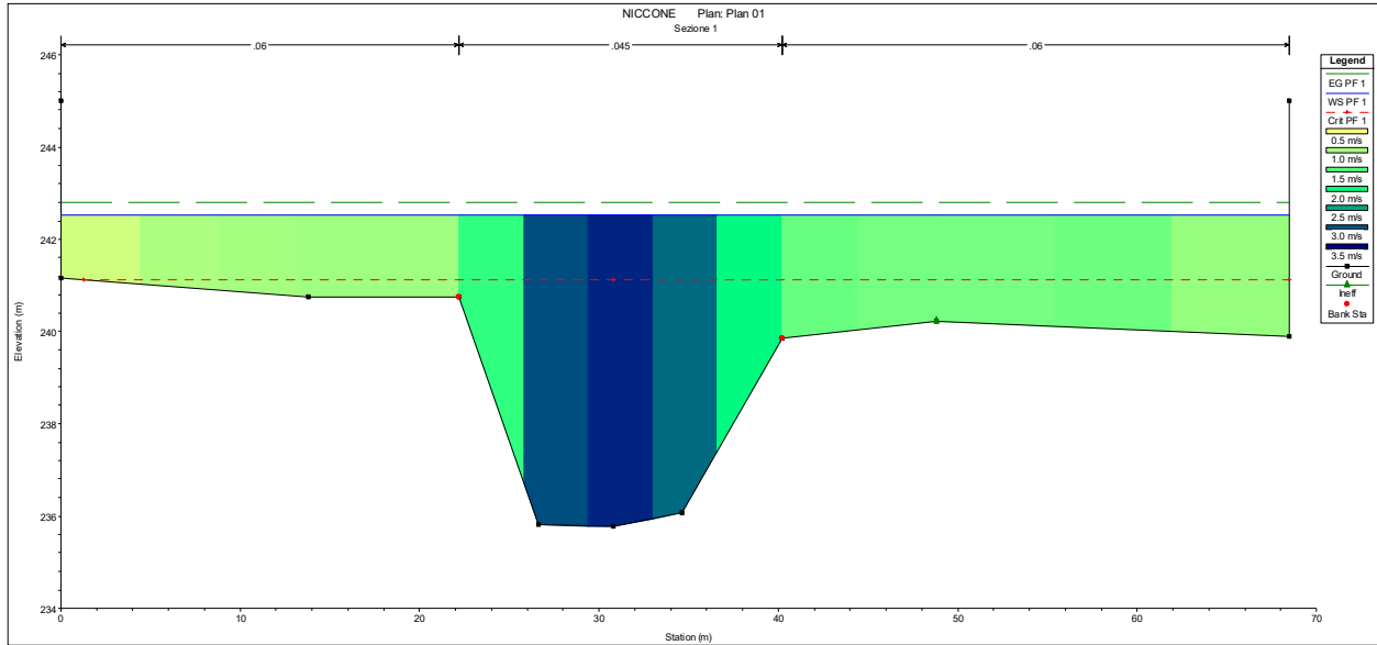
Sezione 1
