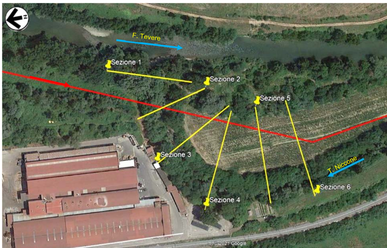
Figura 4.2.2/A – Planimetria del tratto di corso modellato con riportate le sezioni di studio (in rosso tracciato metanodotto, in giallo sez. rilevate)
