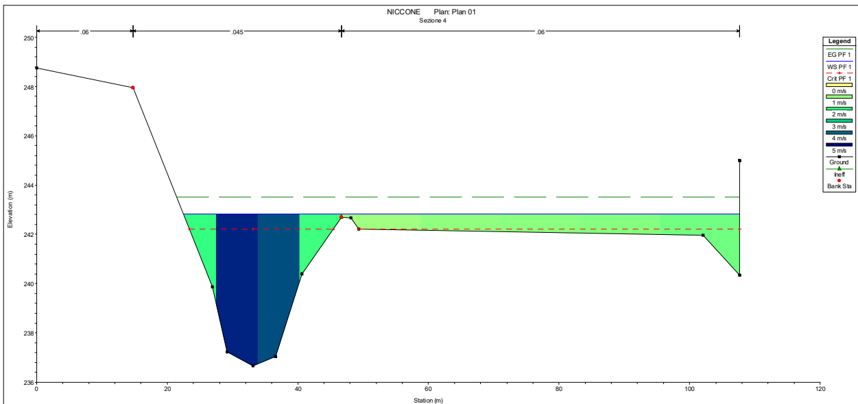
Sezione 4
