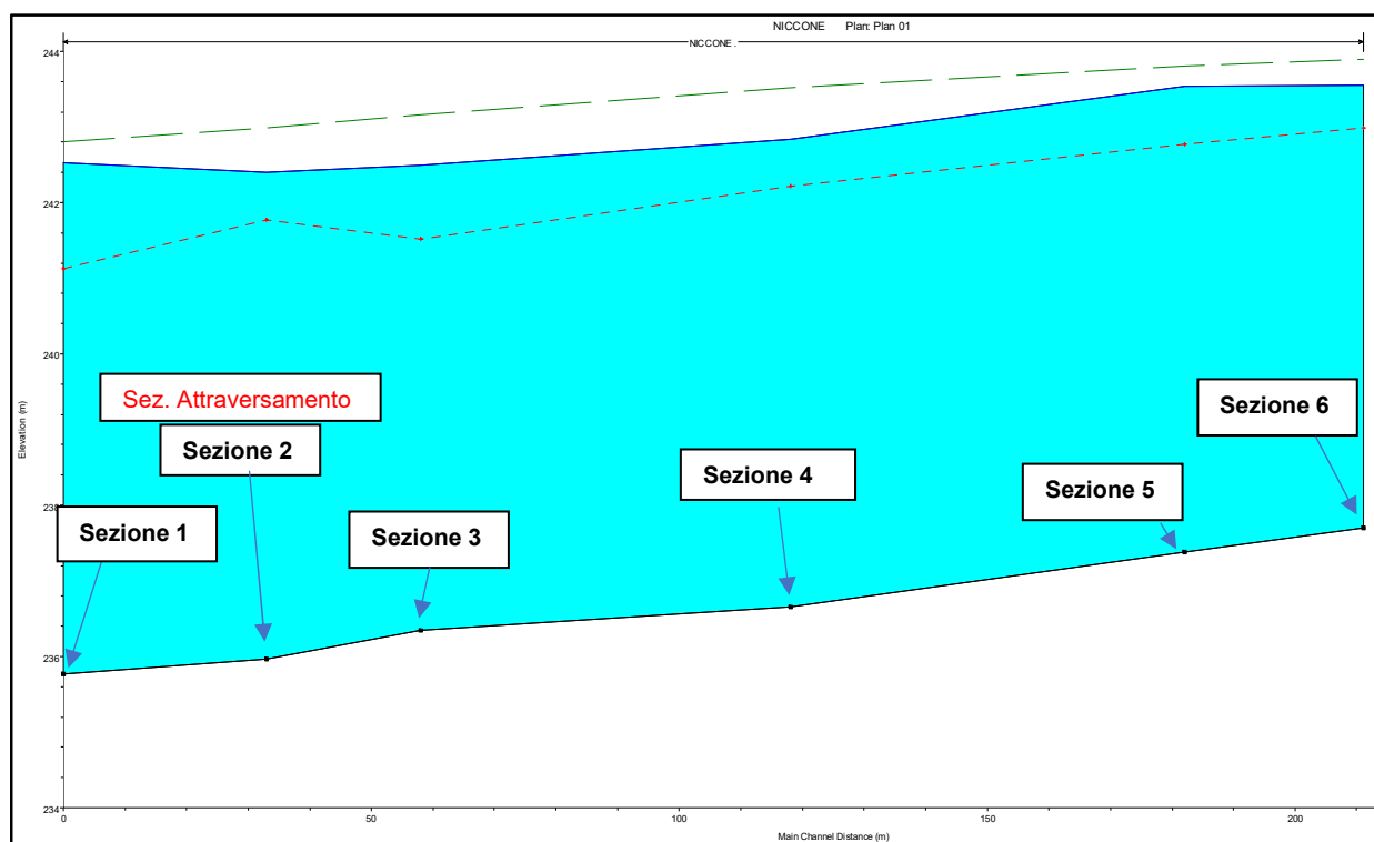
Profilo longitudinale con livelli di piena duecentennale
