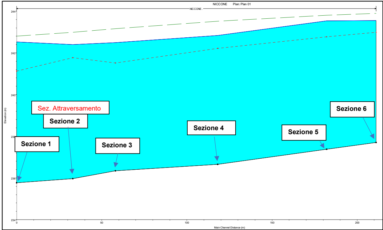
Figura 4.2.3/A - Profilo longitudinale con livelli di piena duecentennale
