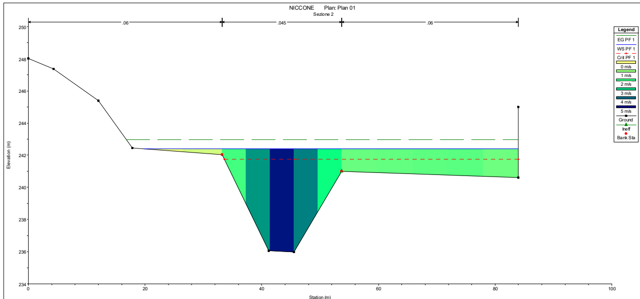
Sezione 2 Attraversamento
