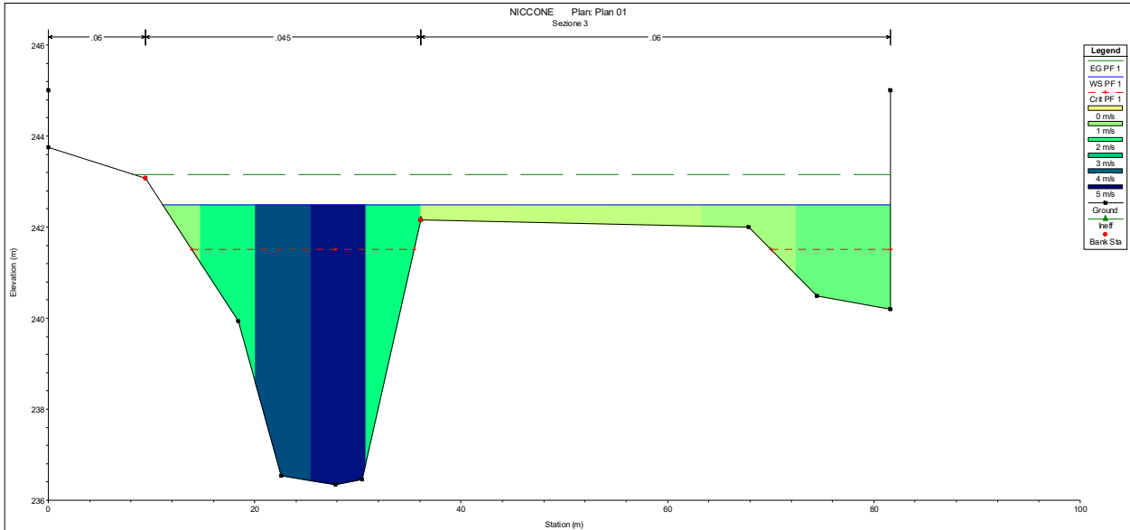
Sezione 3
