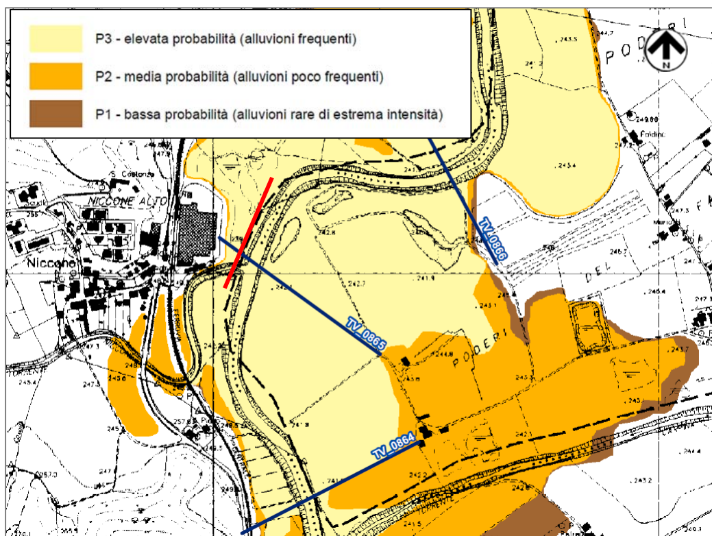
Figura 4.1/A – Stralcio della mappa di pericolosità del PGRAAC (TAV. 11 P) (in rosso sezione di attraversamento)
