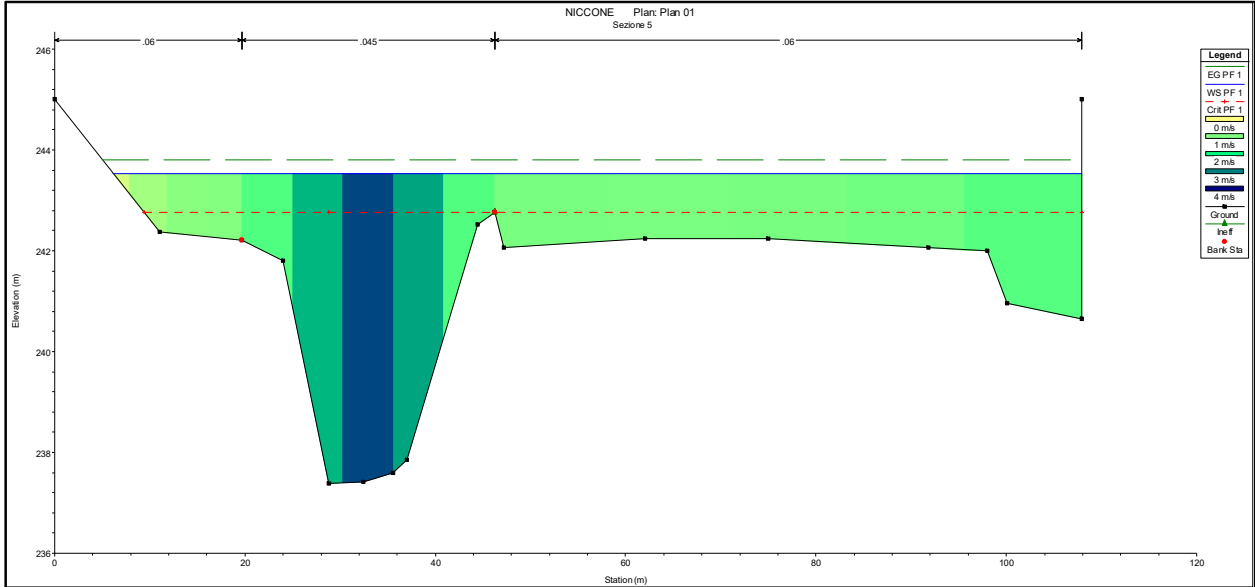
Sezione 5
