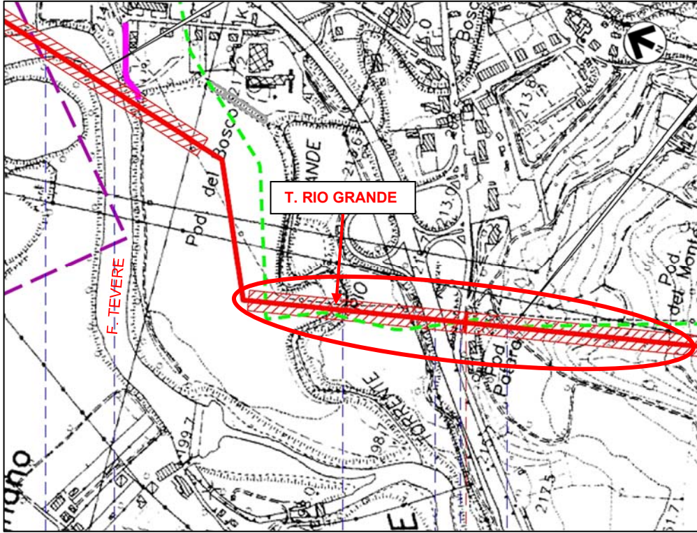
Figura 1/B – Stralcio CTR con localizzazione dell'attraversamento
