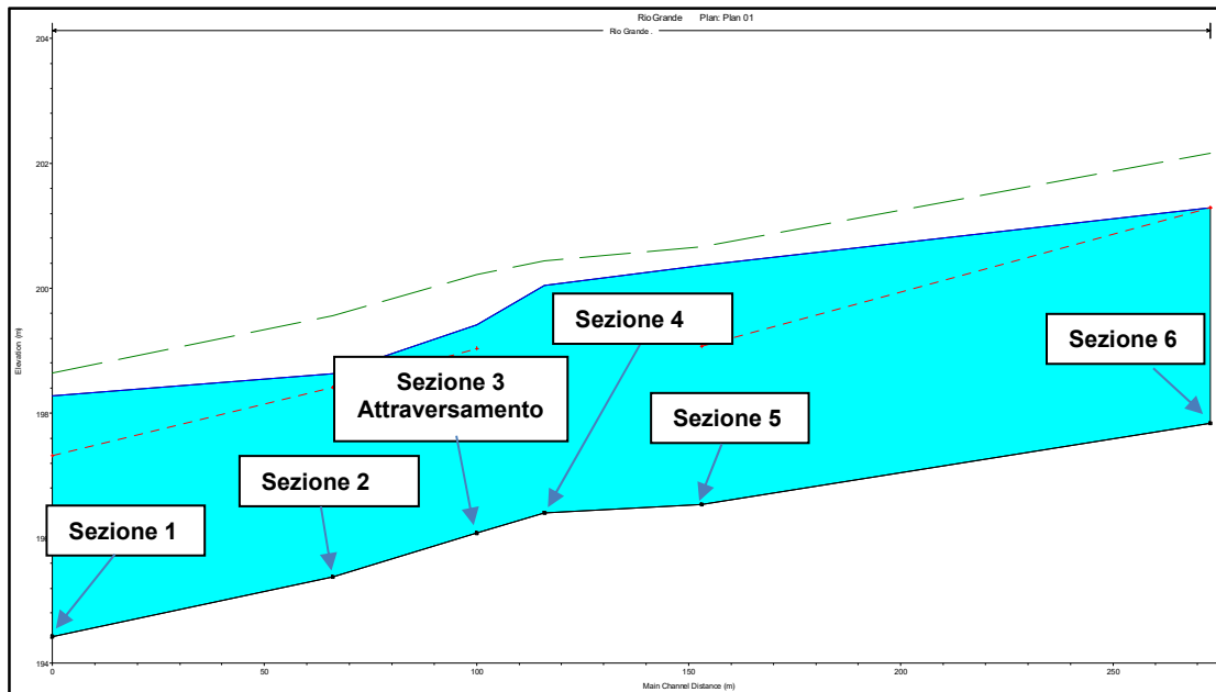
- Figura 4.2.3/A – Profilo longitudinale con livello idrico
