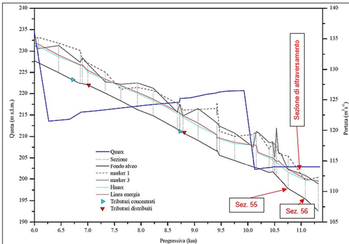
Figura 4.1/C – Involuppo dei massimi livelli calcolati per l'evento di piena con tempo di ritorno 200 anni. E' riportata anche la geometria dell'alveo (da Studio CNR-IRPI).
