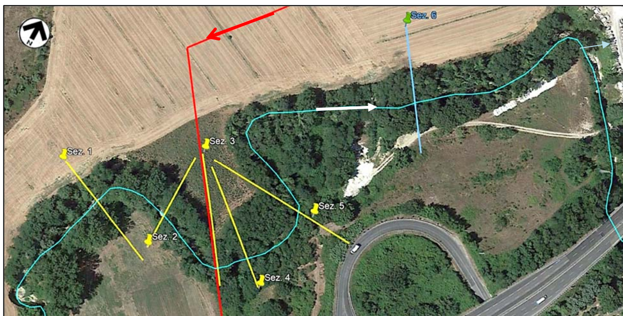
Figura 4.2.2/A – Ubicazione delle sezioni idrauliche (in rosso tracciato metanodotto, in giallo sezioni rilevate, in azzurro sezioni PAI)
