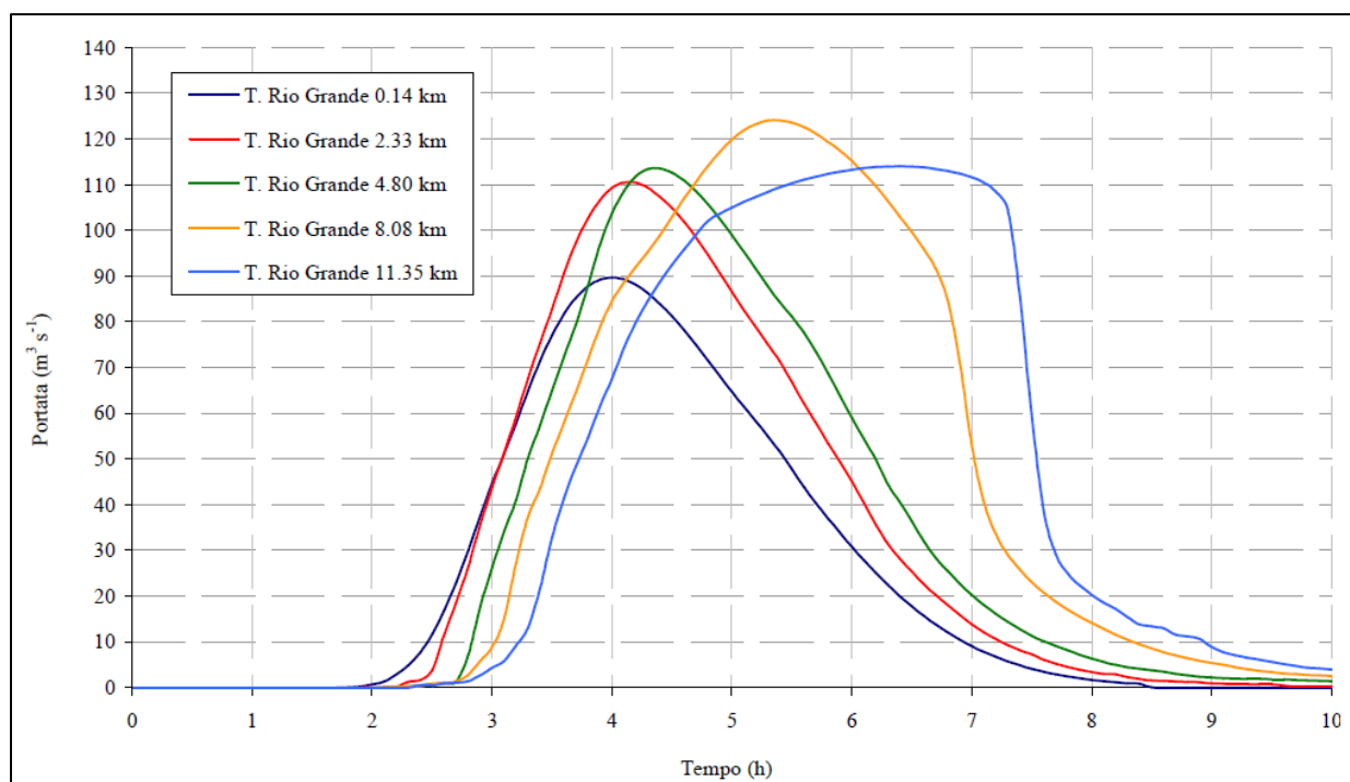
Figura 3/B – Idrogrammi di piena in diverse sezioni (da Studio CNR-IRPI)
