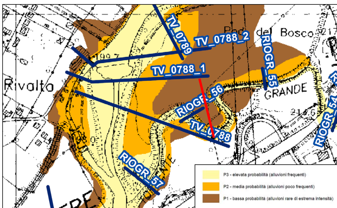
Figura 4.1/A – Localizzazione delle sezioni di studio CNR-IRPI su mappa PRGA (linea rossa: attraversamento metanodotto)
