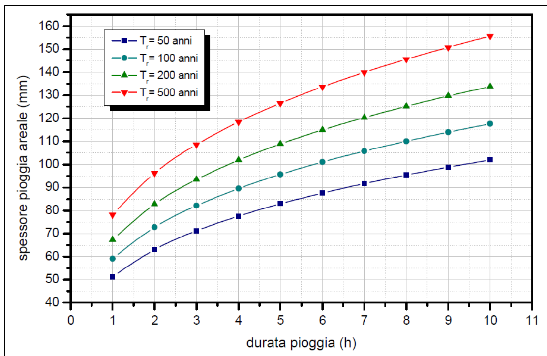
Figura 3/A – Linee segnalatrici di possibilità pluviometrica per il bacino del T. Rio Grande (da studio CNR-IRPI)
