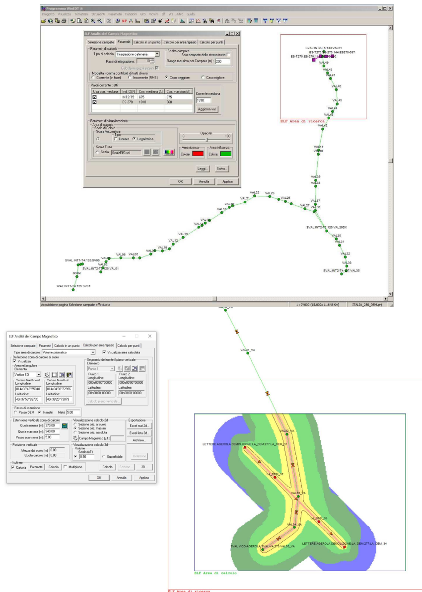
Figura 2 – Schema del modello impostato per le valutazioni CEM sul sistema WinEDT
