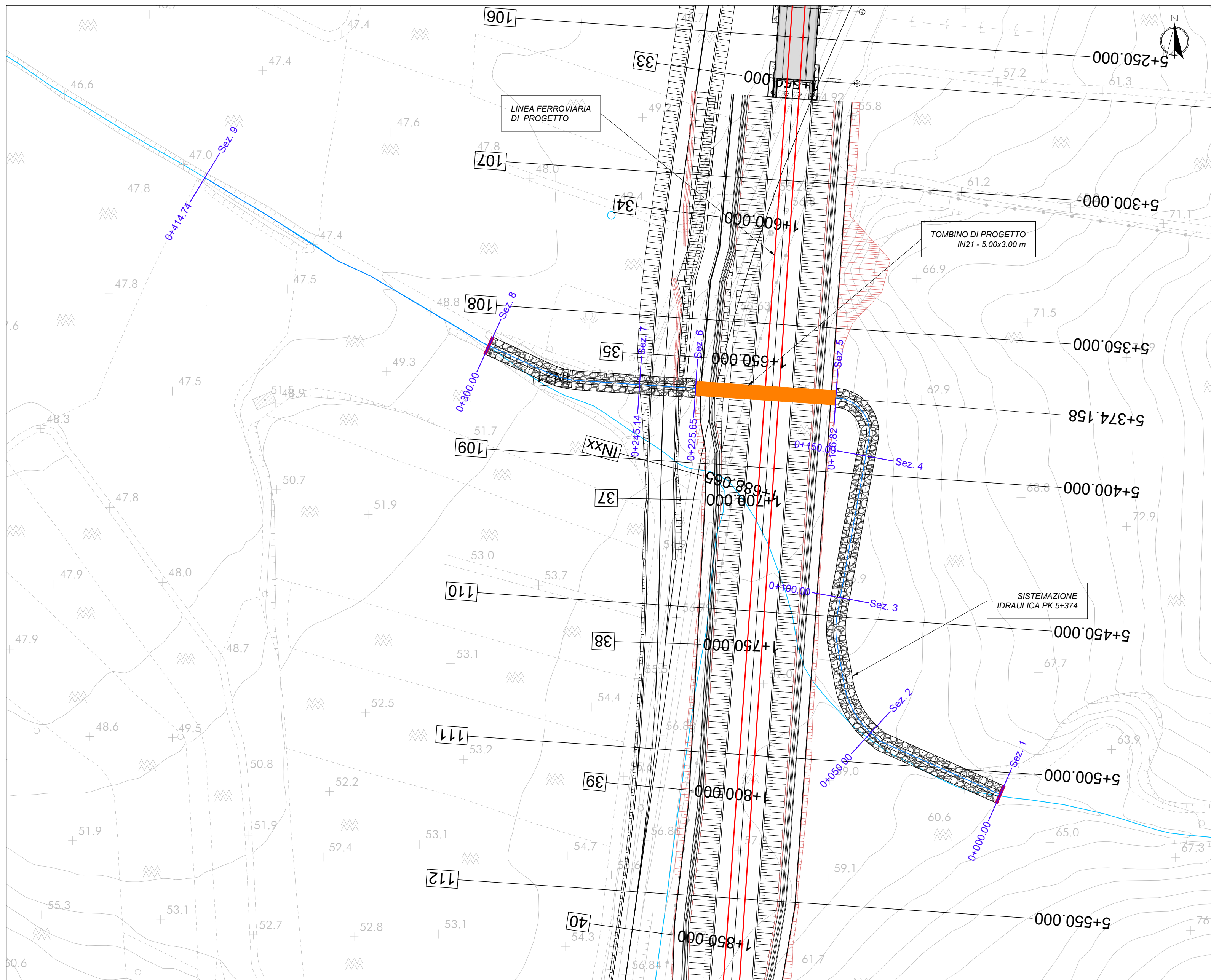
PLANIMETRIA - Scala 1:1000
