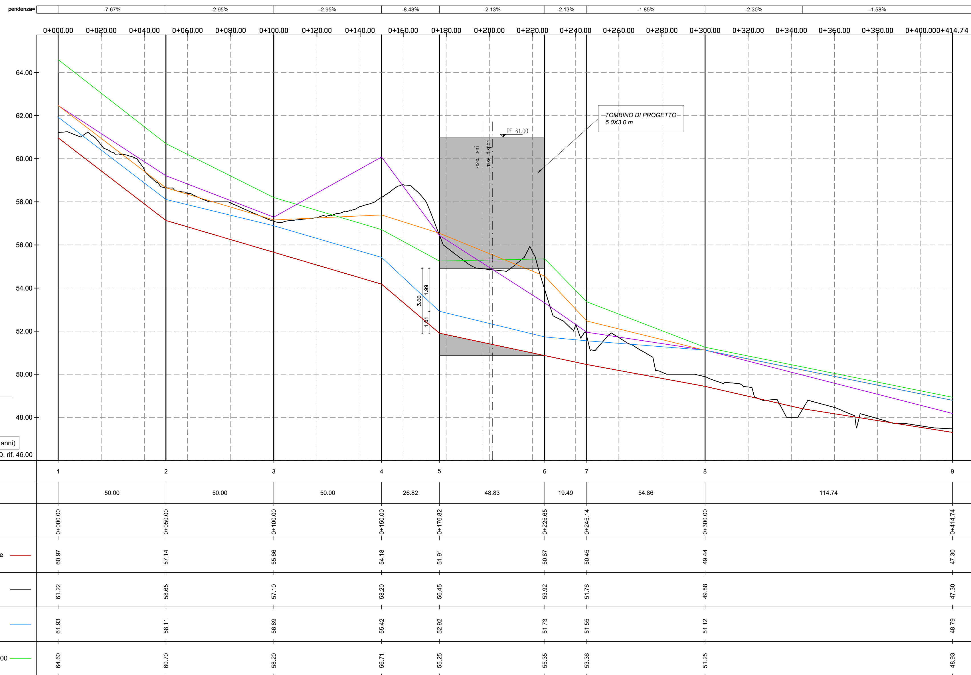
PROFILO - Scala 1:1000/100
