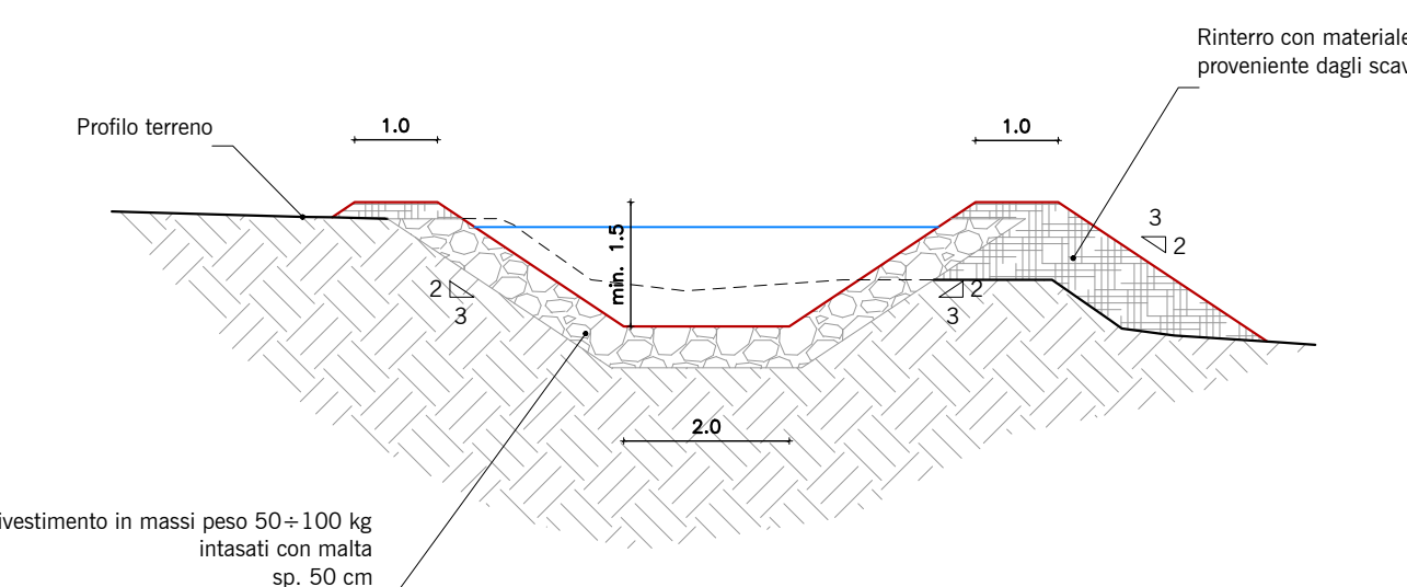
SEZIONE TIPO SISTEMAZIONE SCALA 1:100
