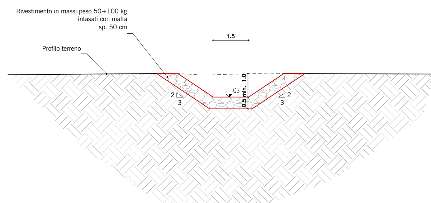
SEZIONE TIPO SISTEMAZIONE SCALA 1:100
