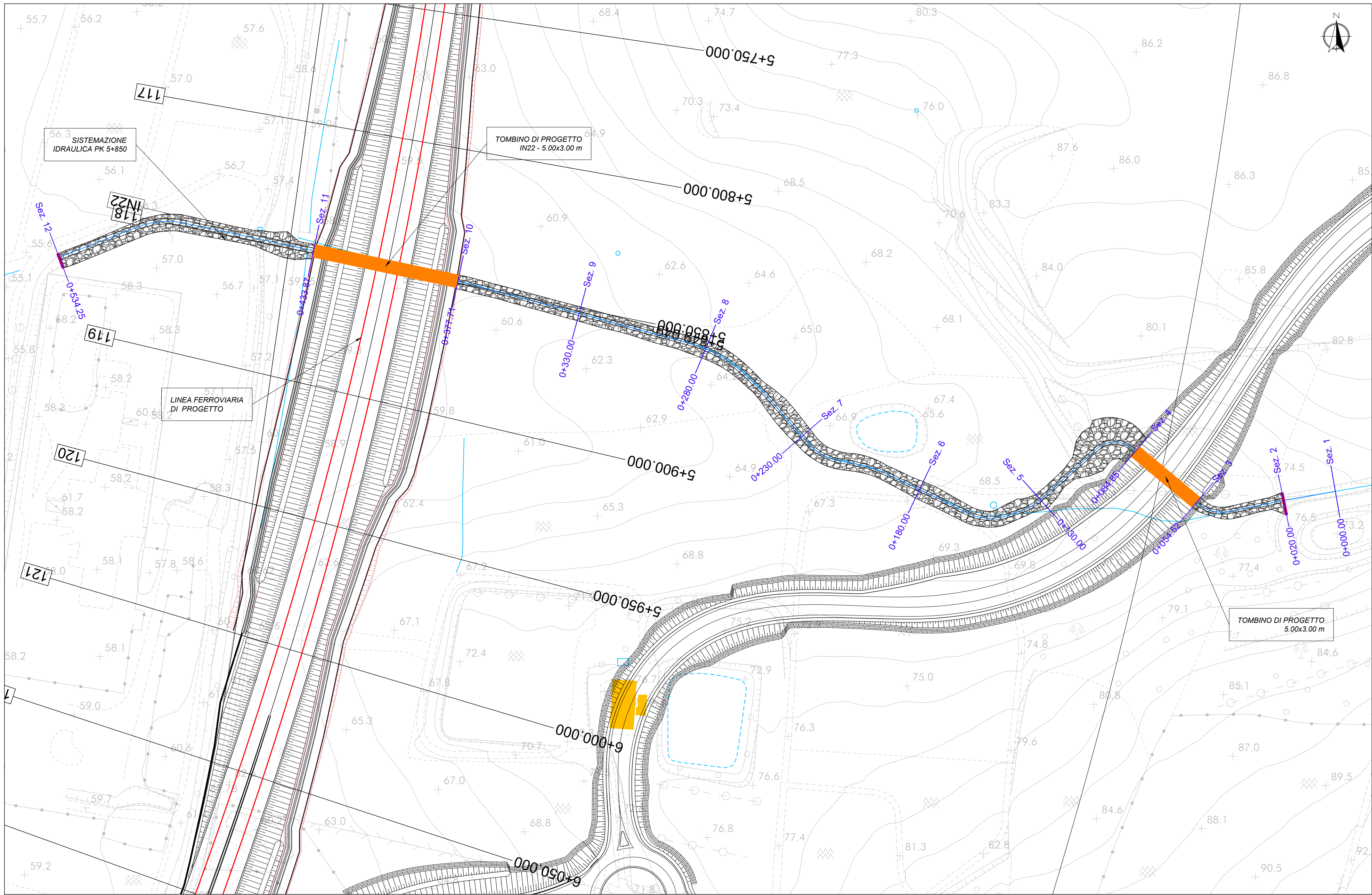
PLANIMETRIA - Scala 1:1000
