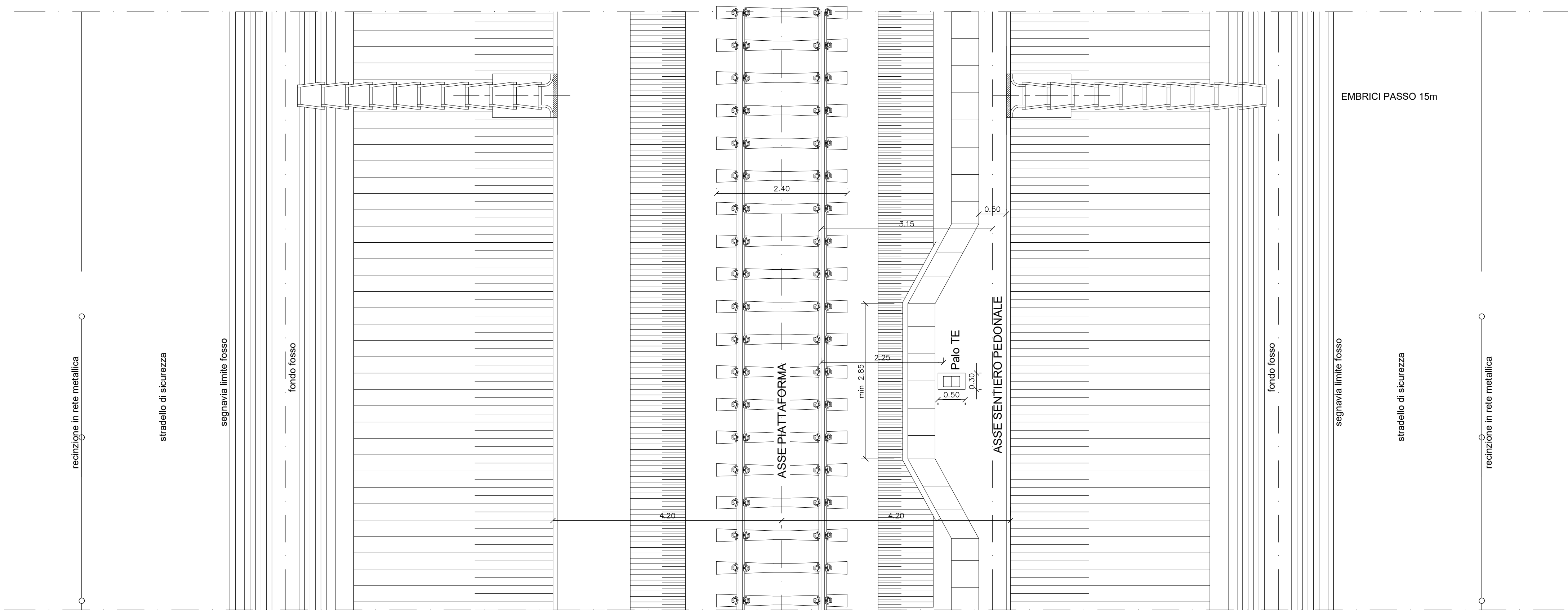
PIANTA TIPO IN RILEVATO 1:50
