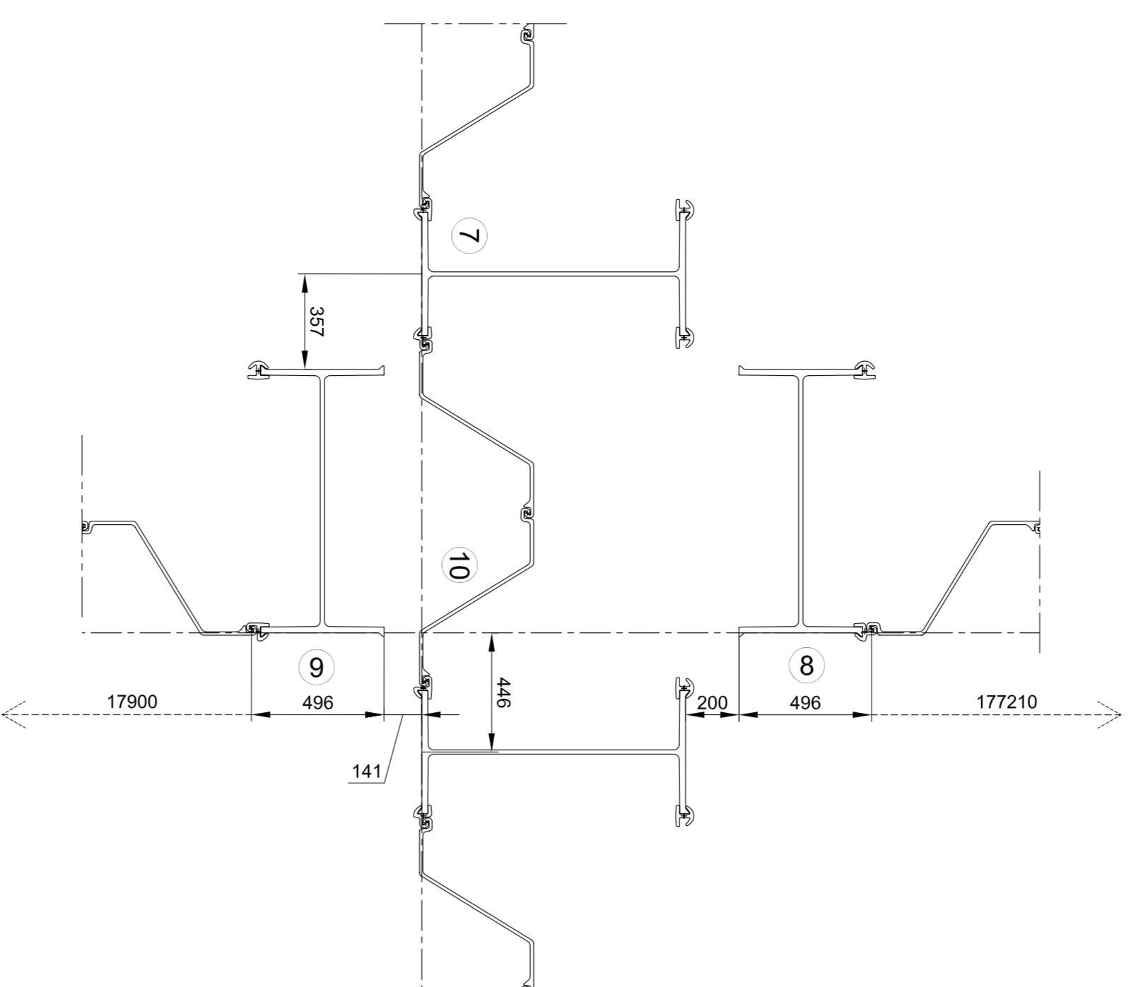
Particolare D (1/20)
