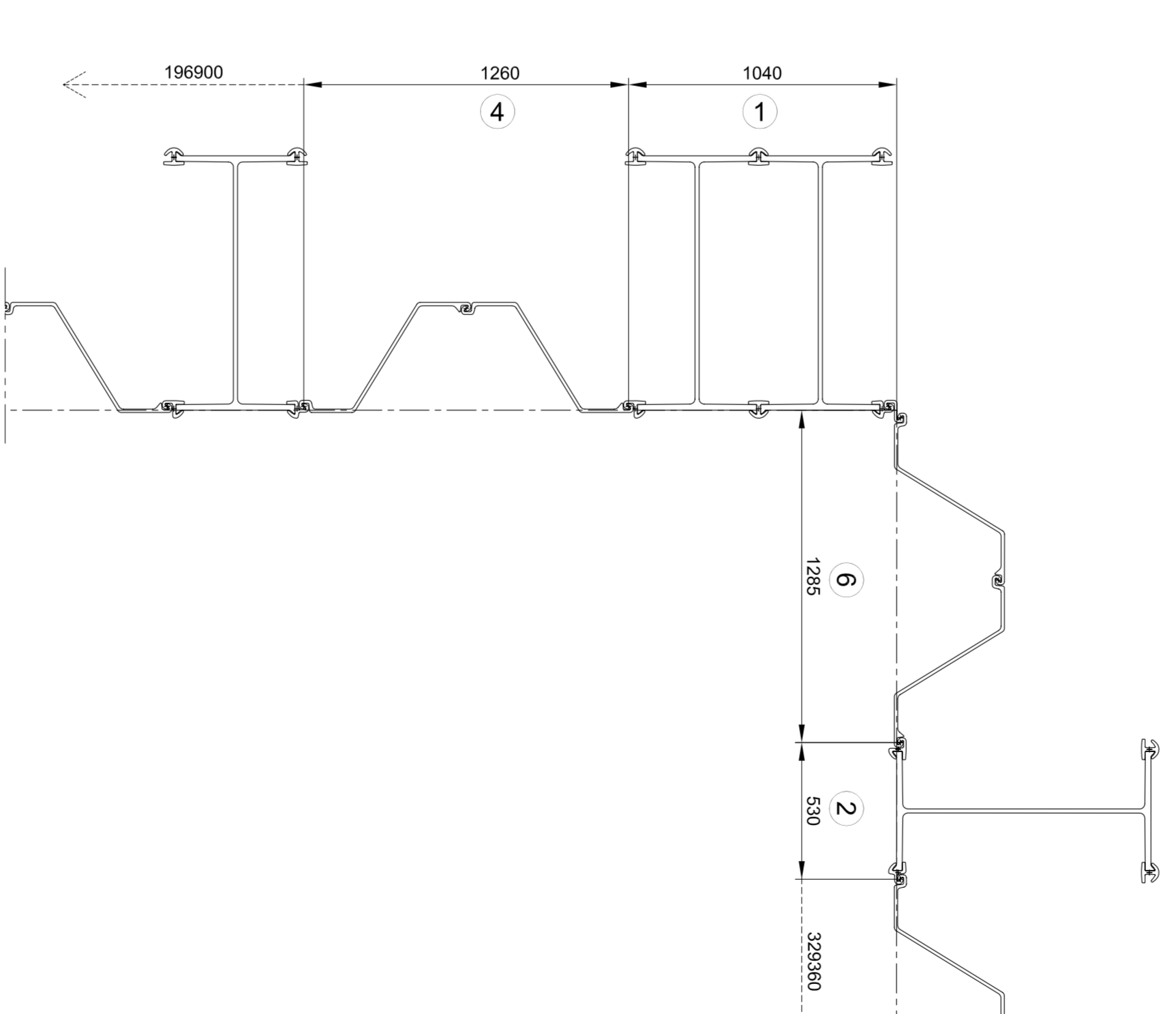
Particolare C (1/20)
