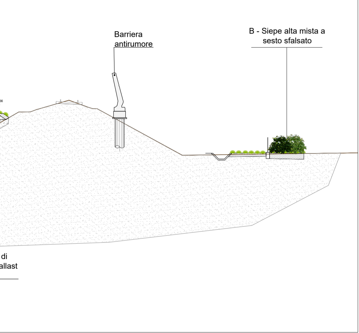
4 - SEZIONE 145 km 7+200 Sc. 1:200
