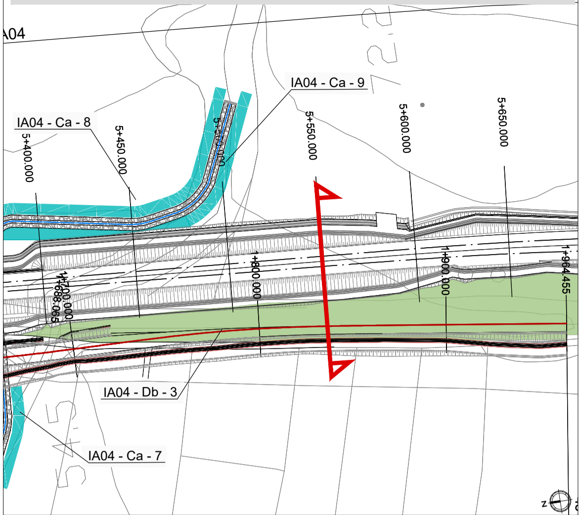
3 - SEZIONE 112 km 5+550 Sc. 1:200
