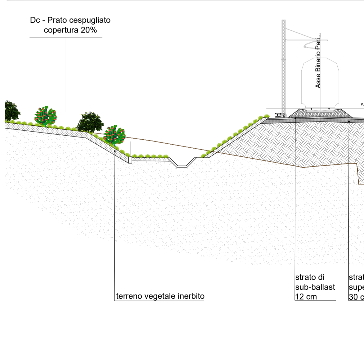
3 - SEZIONE 112 km 5+550 Sc. 1:200
