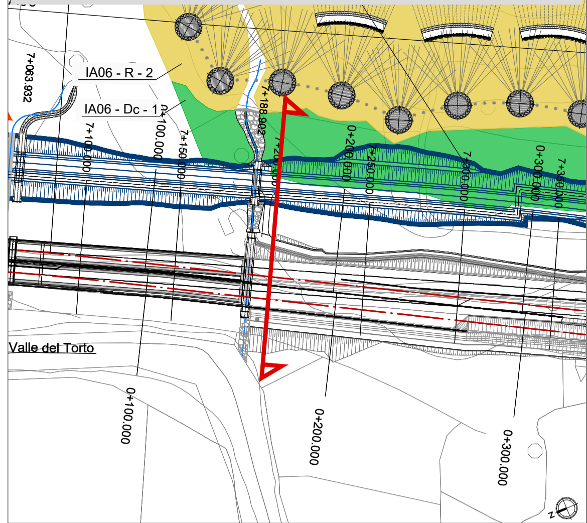
4 - SEZIONE 145 km 7+200 Sc. 1:200
