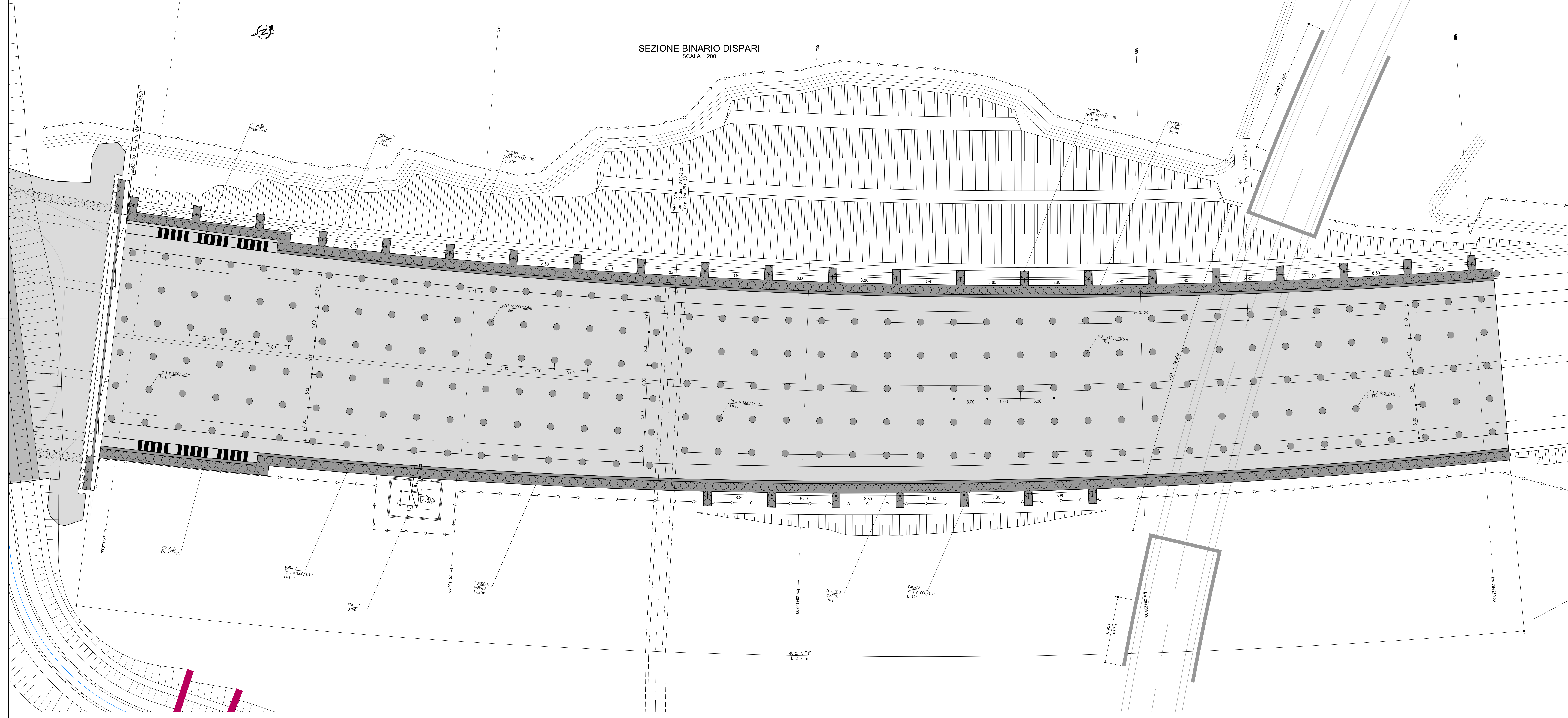
SEZIONE BINARIO DISPARI SCALA 1:200
