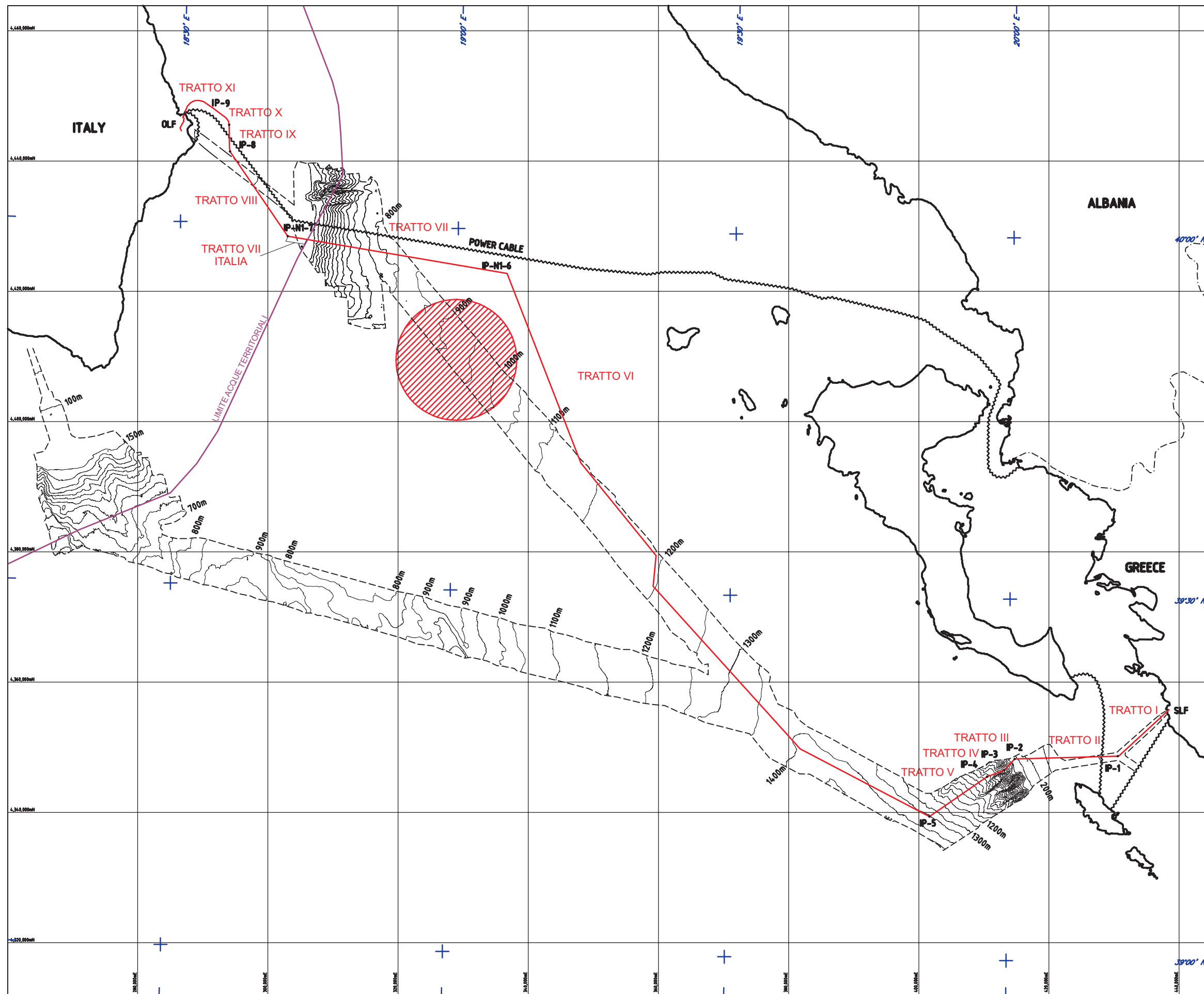
FIGURA 3.1 METANODOTTO DI INTERCONNESSIONE ITALIA - GRECIA TRACCIATO OFF-SHORE
