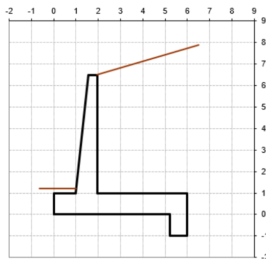
Figura 2.2 – Sezione tipologica
