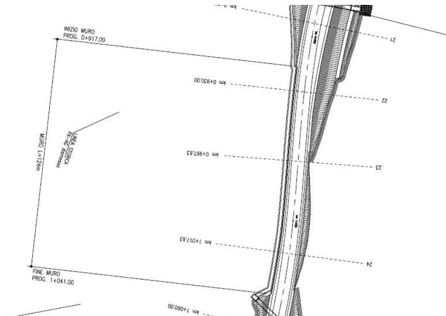
Figura 2.1 – Planimetria di progetto (posizione definitiva)
